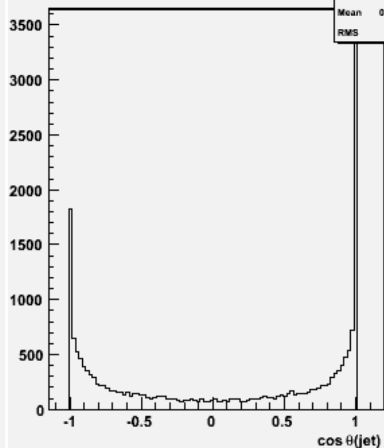
cos \theta for 2-jets :w102529 e1e1ssss_o
