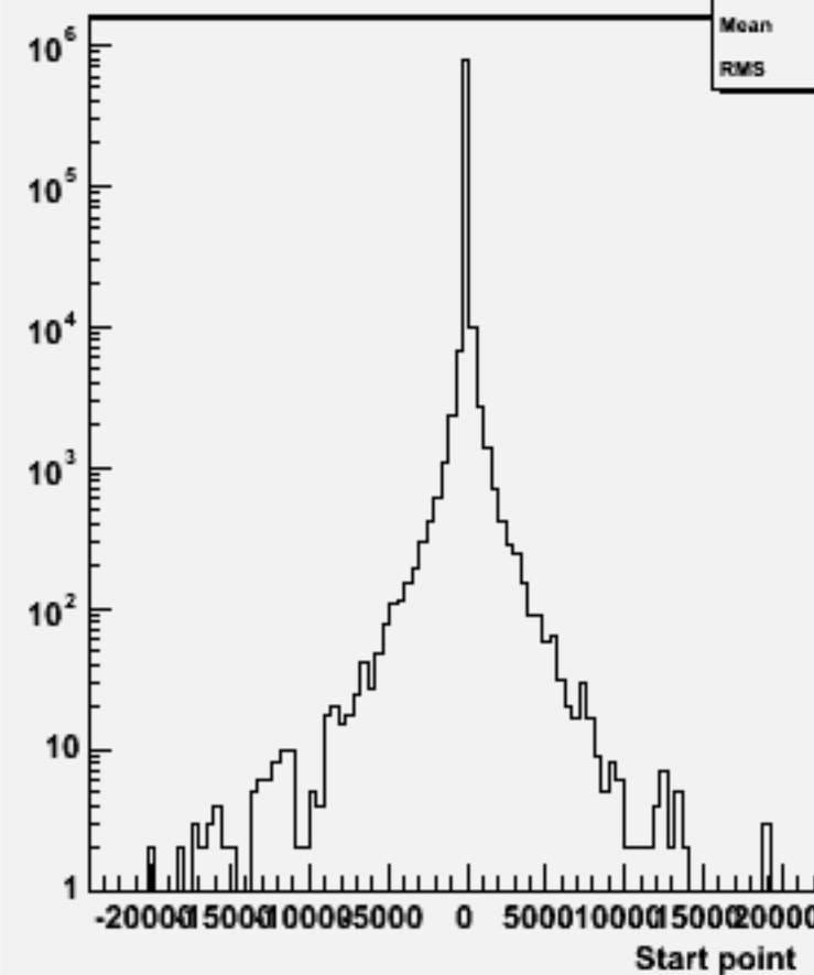
Start point Z : w102529 e1e1ssss_o
