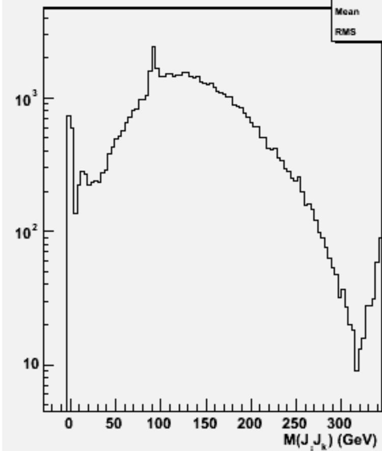
2jets mass(All comb)w102529 e1e1ssss_o
