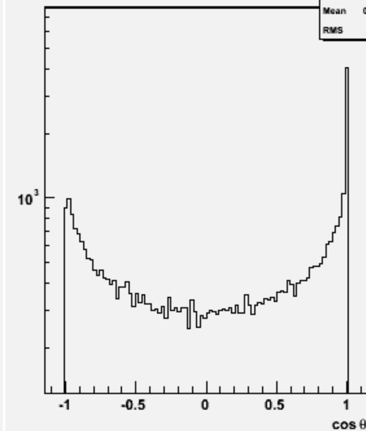
Jet cosθ (All jets)w102529 e1e1ssss_o
