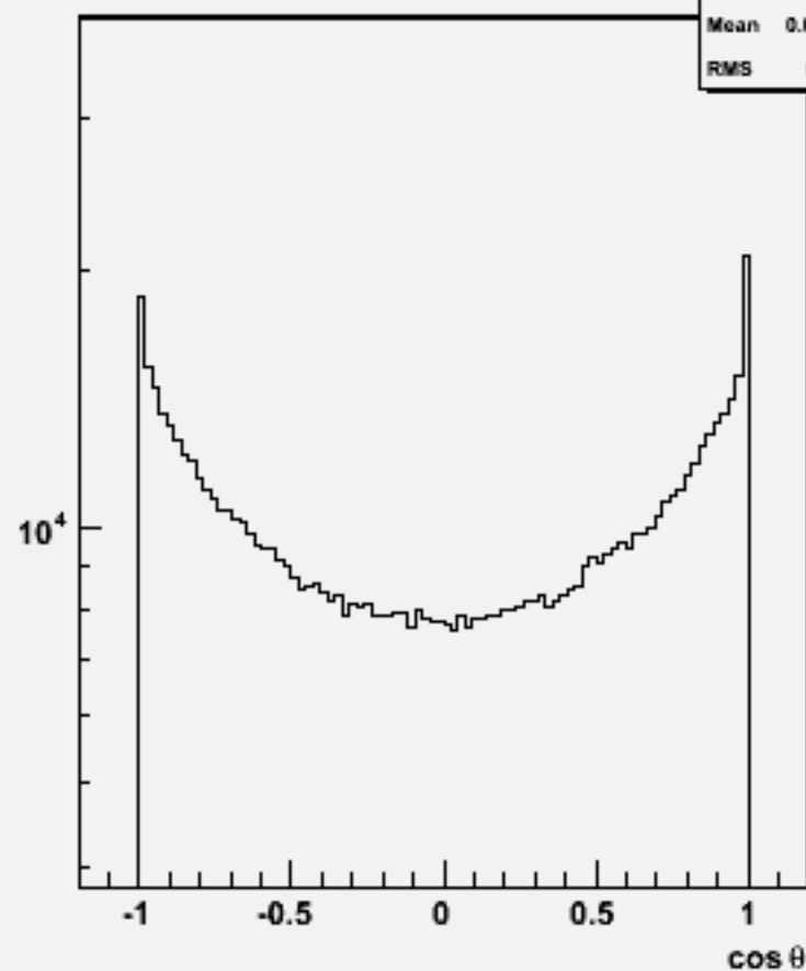
Particle cosθ : w102529 e1e1ssss_o
