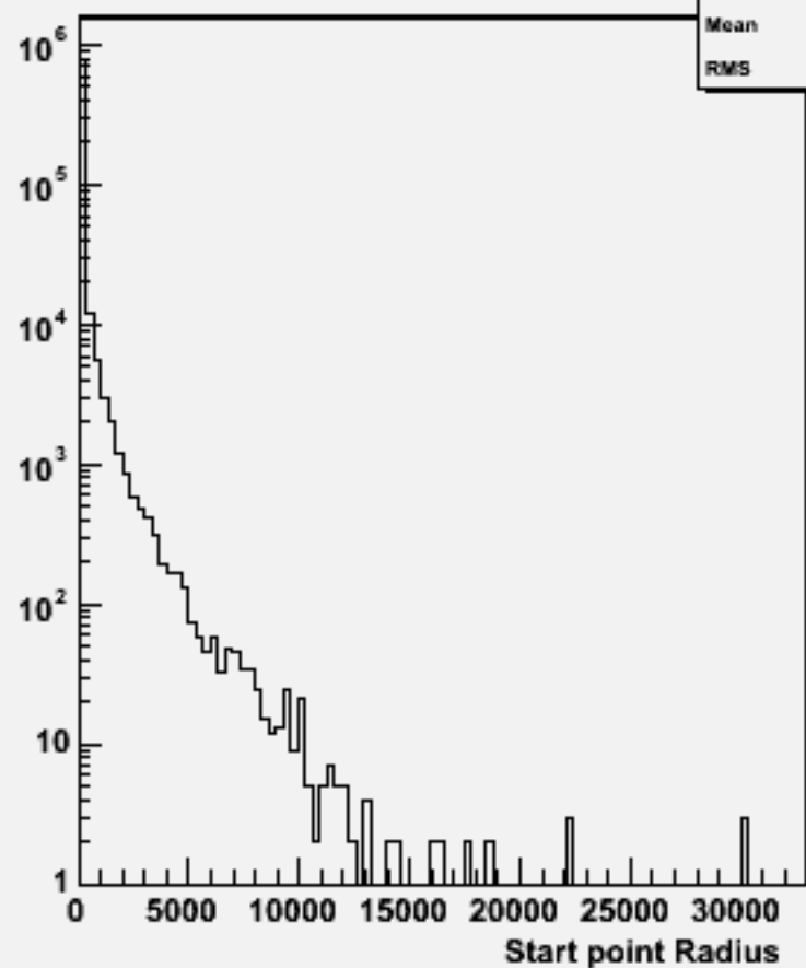
Start point R : w102529 e1e1ssss_o
