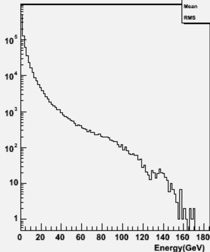
Particle Energy : w102529 e1e1ssss_o
