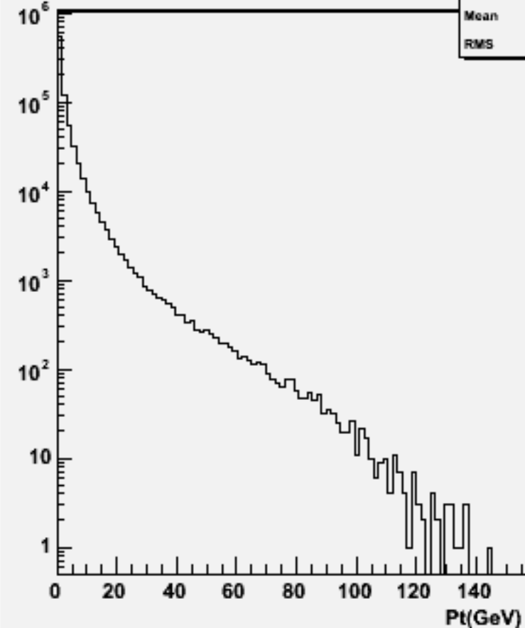
Particle Pt : w102529 e1e1ssss_o
