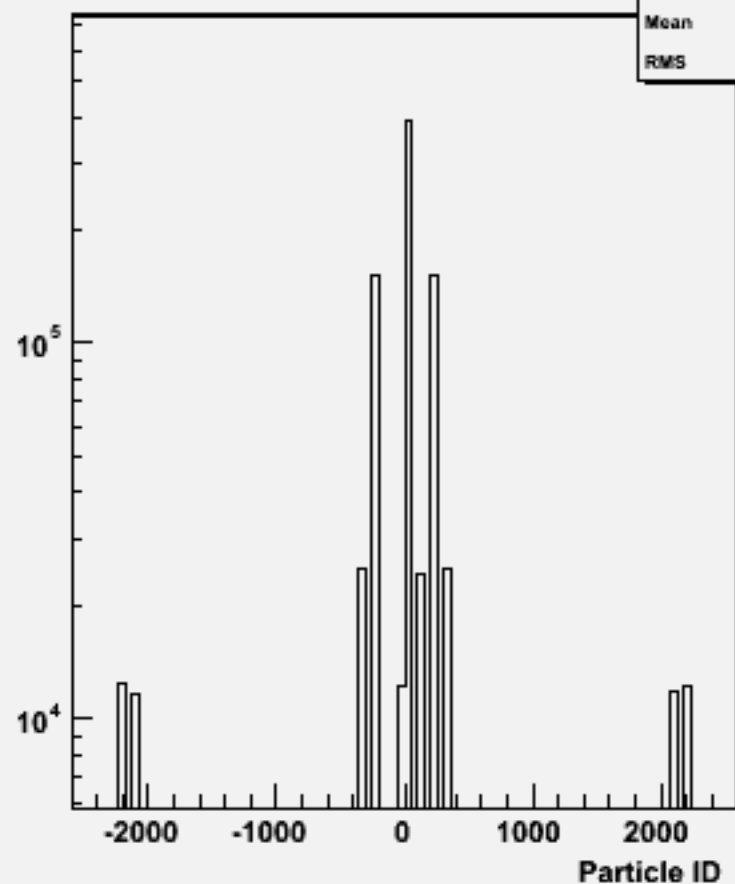
Particle ID : w102529 e1e1ssss_o
