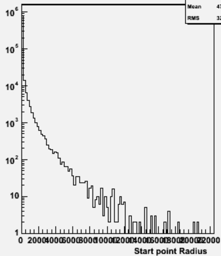
Start point R : w102528 e1e1ssss_o
