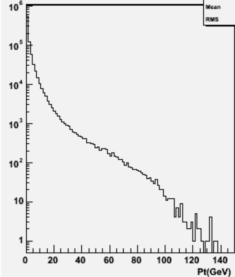
Particle Pt : w102528 e1e1ssss_o
