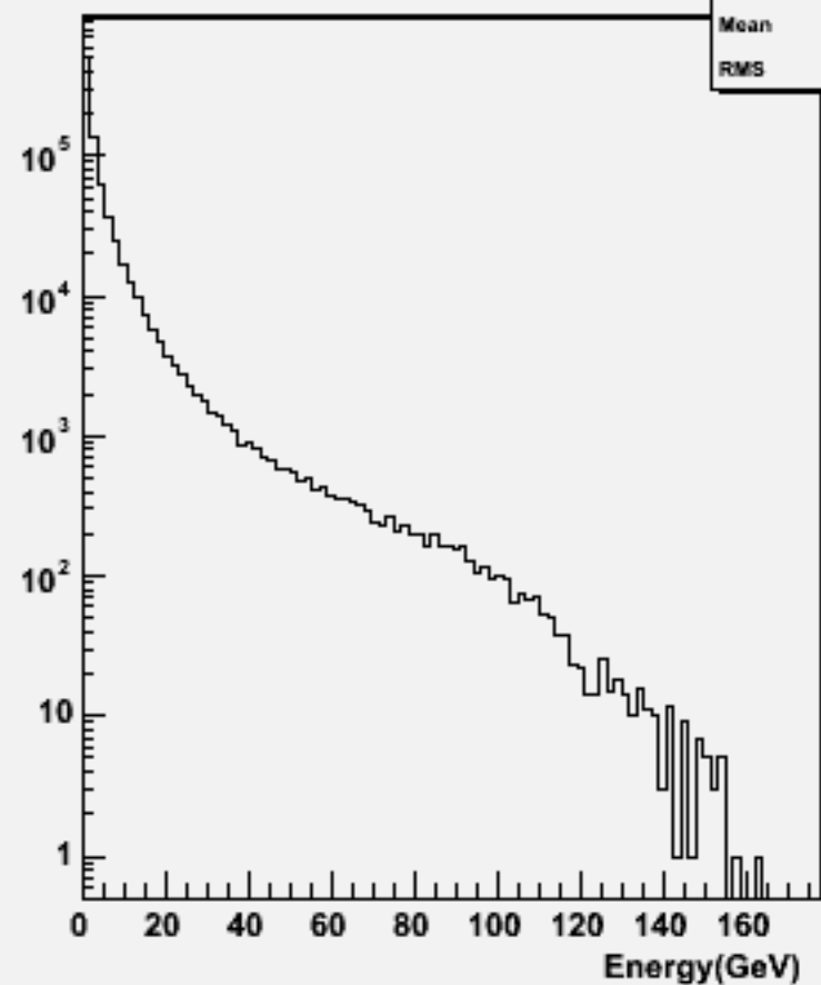
Particle Energy : w102528 e1e1ssss_o
