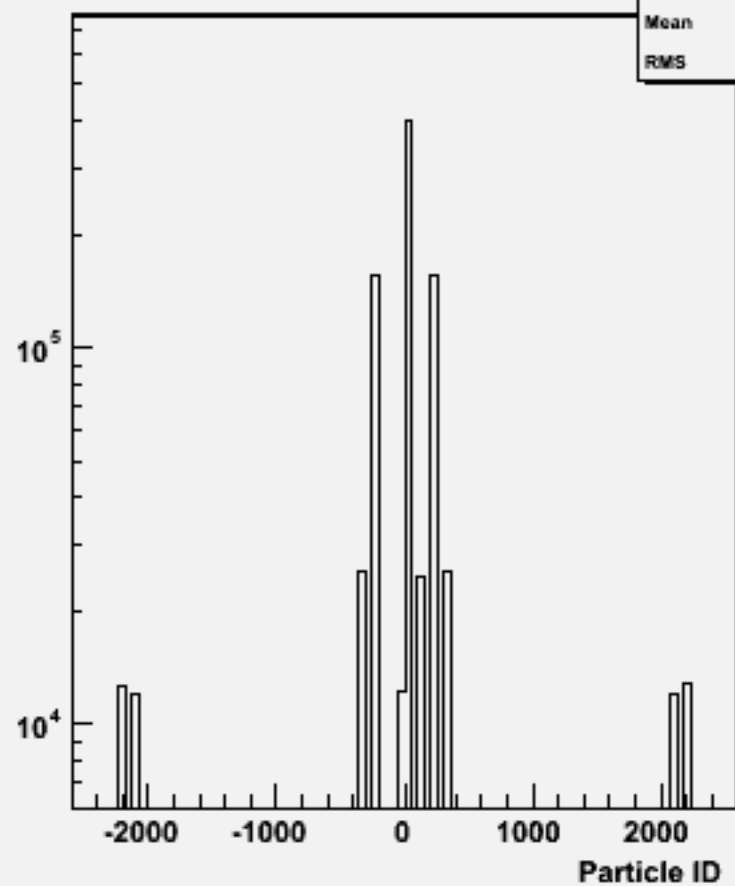
Particle ID : w102528 e1e1ssss_o
