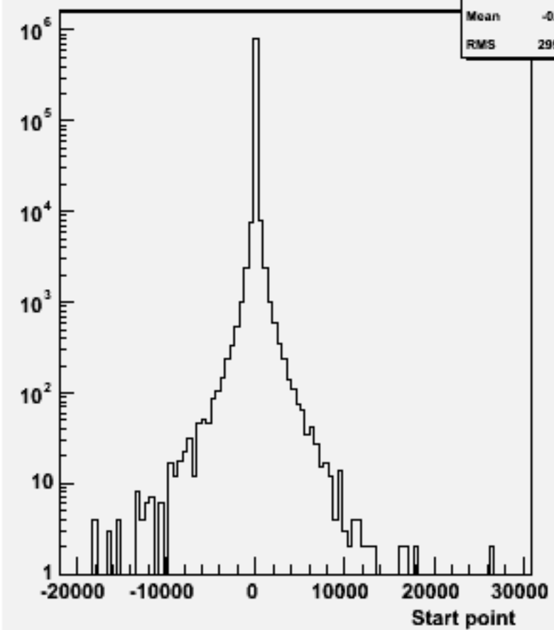
Start point Z : w102528 e1e1ssss_o
