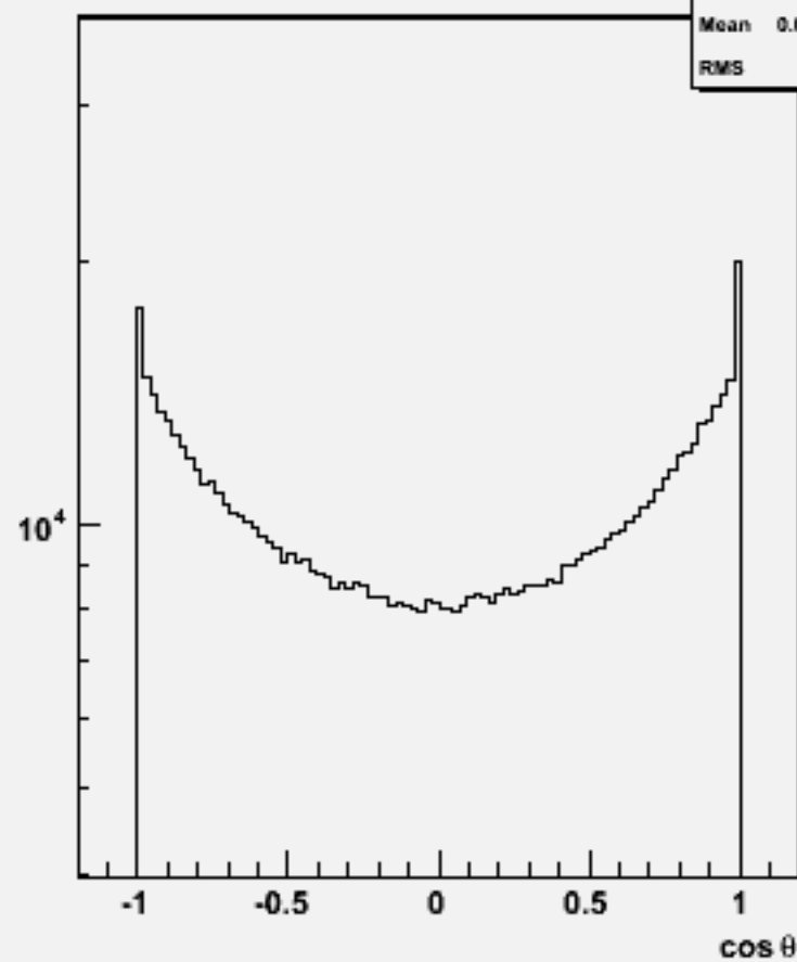
Particle cos \theta : w102528 e1e1ssss_o
