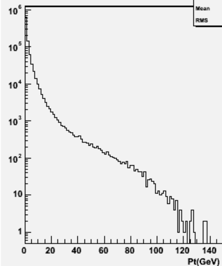
Particle Pt : w102525 e1e1ddb_o
