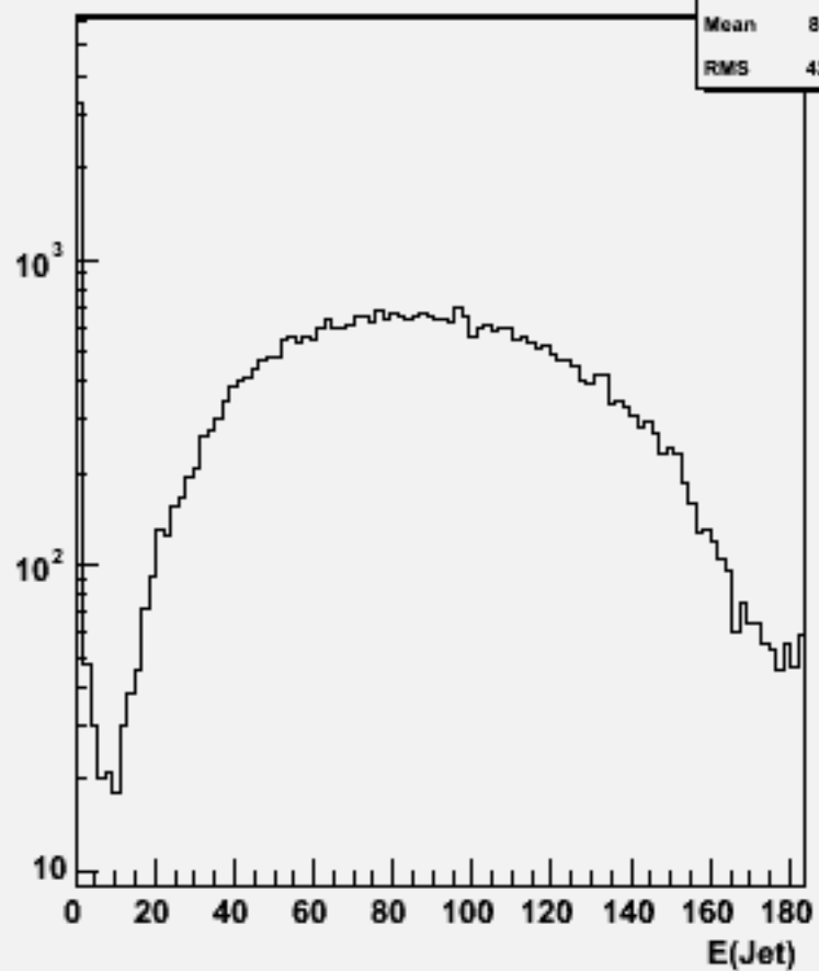
Jet energies(All jets)w102525 e1e1ddb_o
