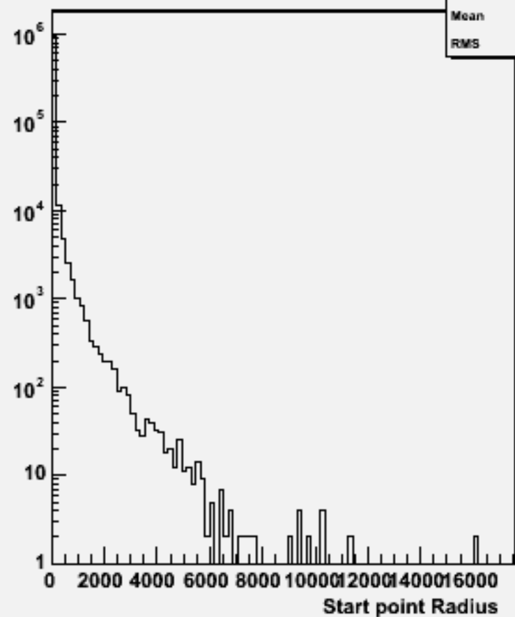
Start point R : w102525 e1e1ddb_o
