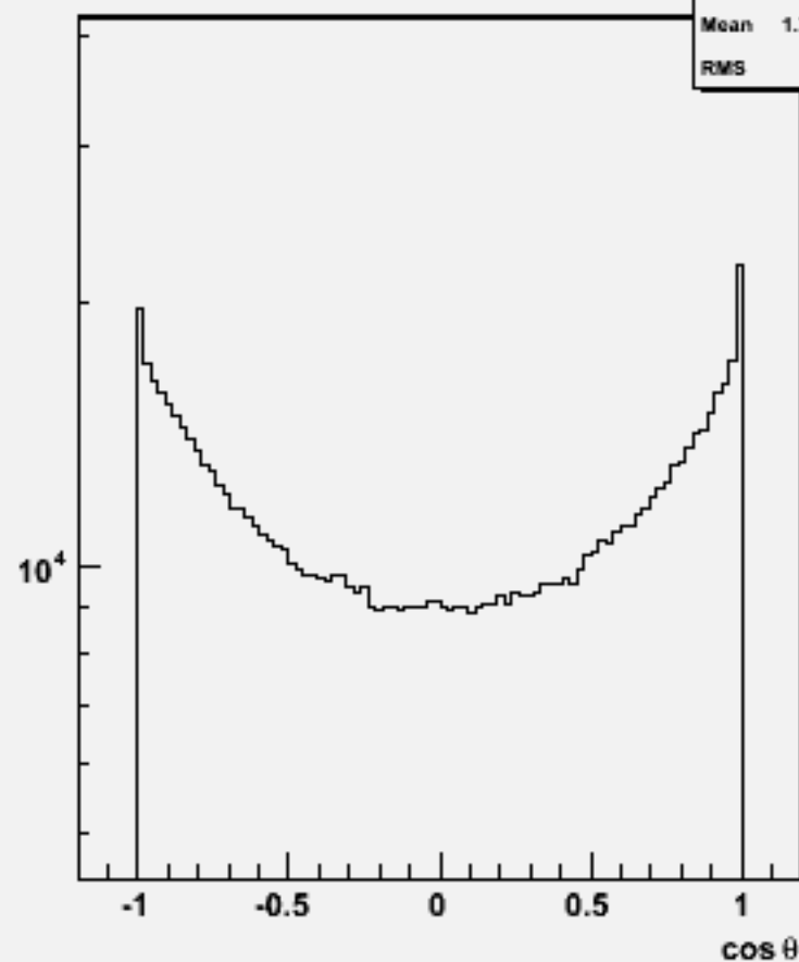
Particle cos \theta : w102525 e1e1ddb_o
