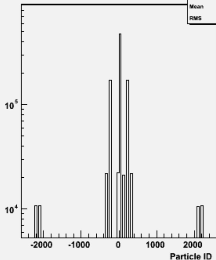
Particle ID : w102525 e1e1ddb_o
