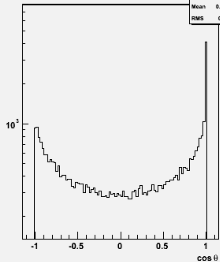
Jet cosθ (All jets)w102525 e1e1ddb_o
