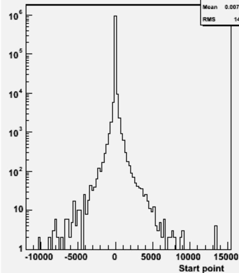
Start point Z : w102525 e1e1ddb_o
