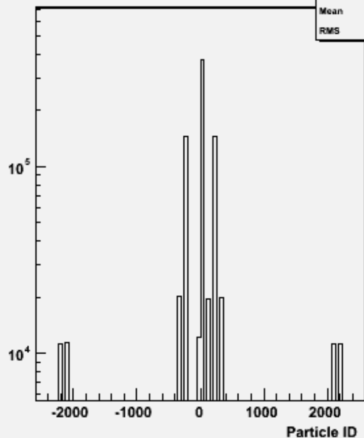
Particle ID : w102522 e1e1ddss_o
