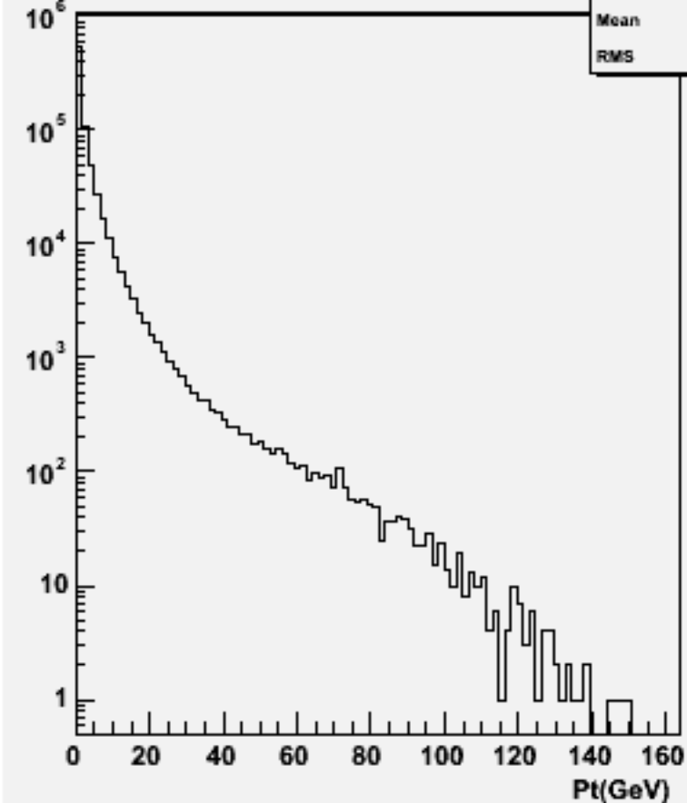
Particle Pt : w102522 e1e1ddss_o
