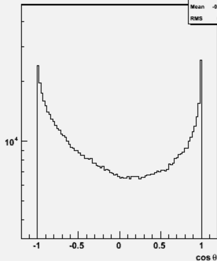
Particle cos \theta : w102522 e1e1ddss_o
