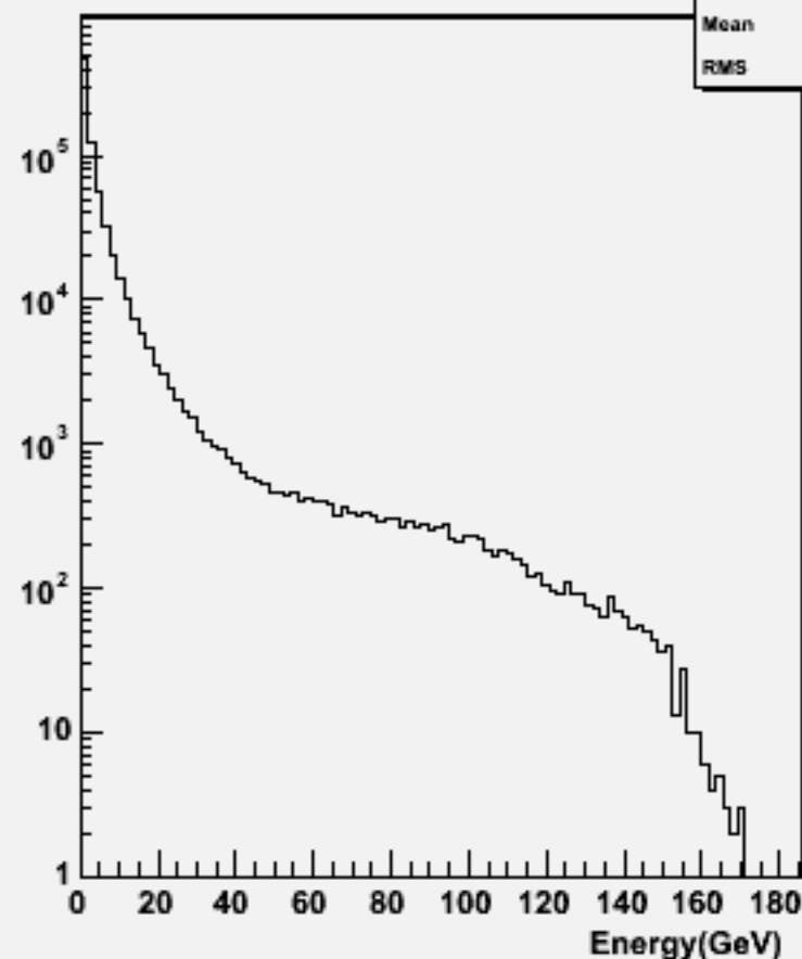
Particle Energy : w102522 e1e1ddss_o
