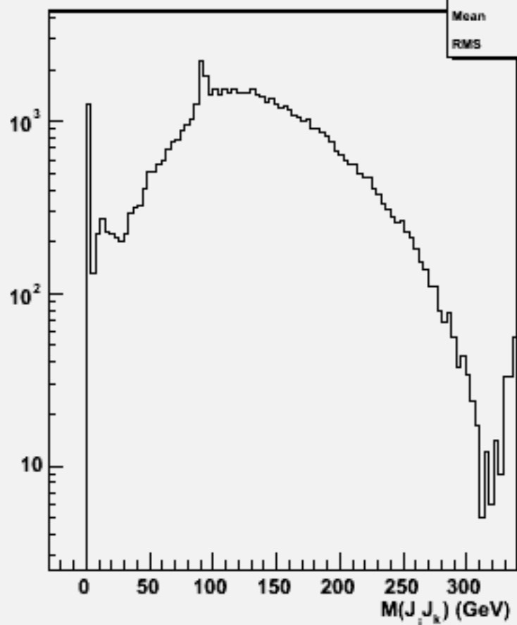
2jets mass(All comb)w102521 e1e1ddss_o
