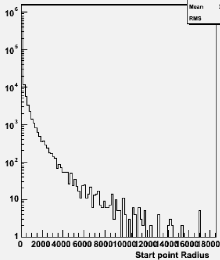
Start point R : w102521 e1e1ddss_o
