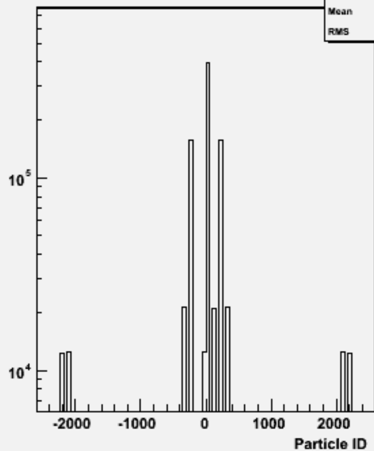
Particle ID : w102521 e1e1ddss_o
