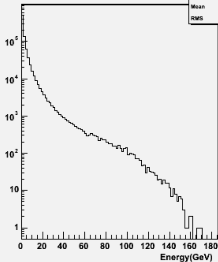
Particle Energy : w102521 e1e1ddss_o
