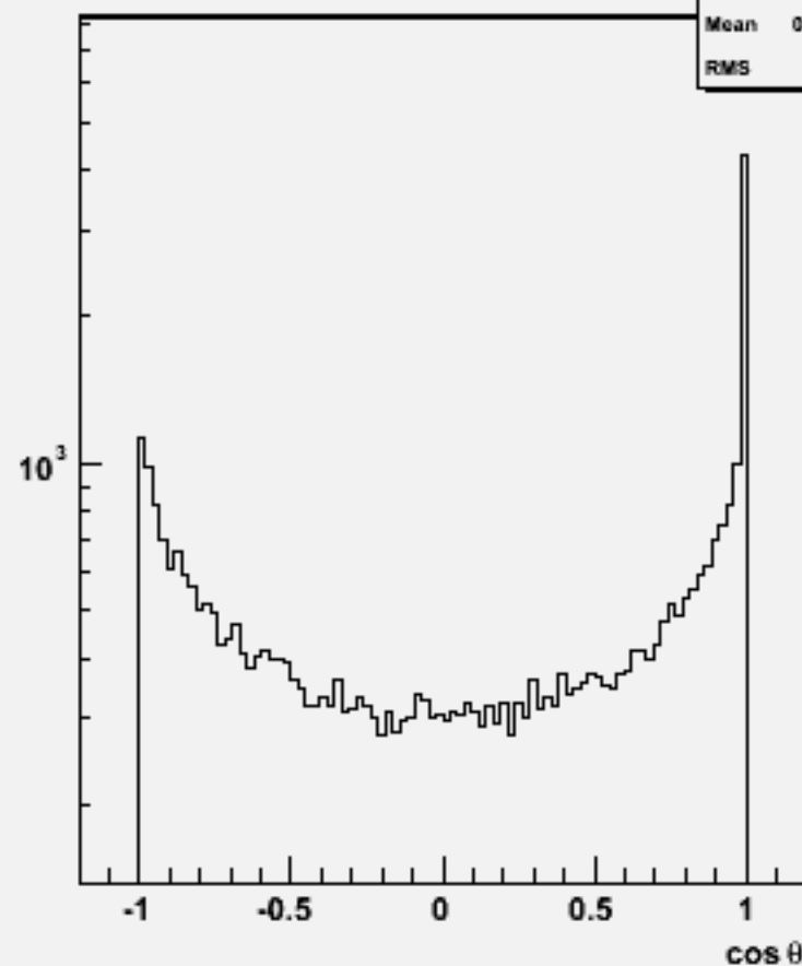
Jet cos \theta (All jets)w102521 e1e1ddss_o
