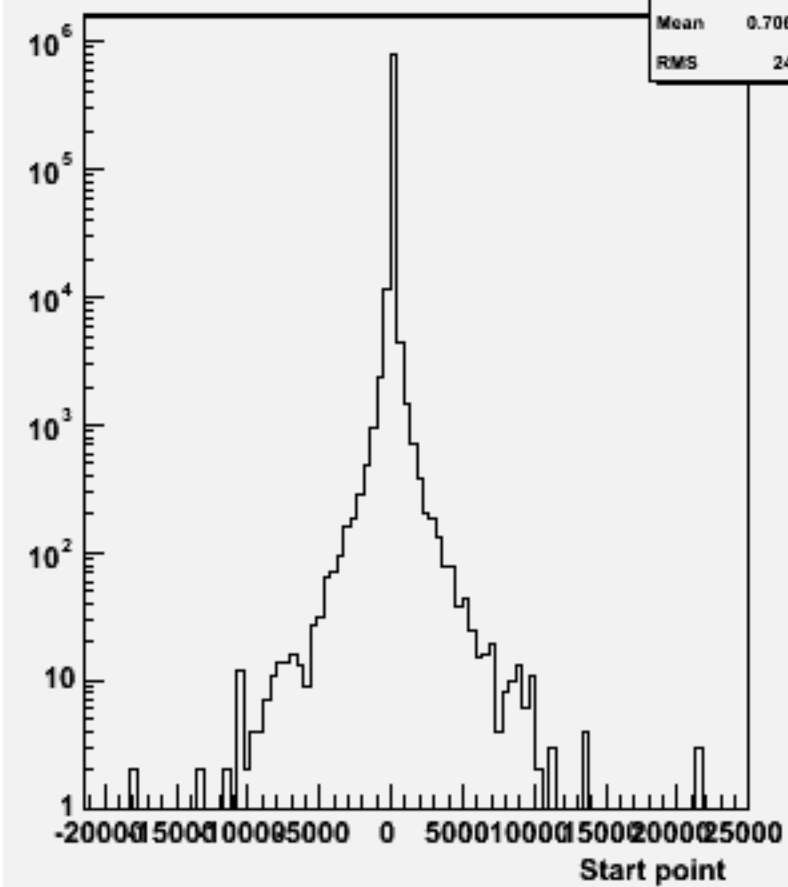
Start point Z : w102521 e1e1ddss_o
