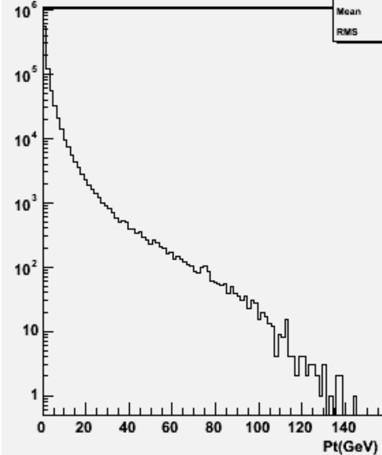
Particle Pt : w102521 e1e1ddss_o
