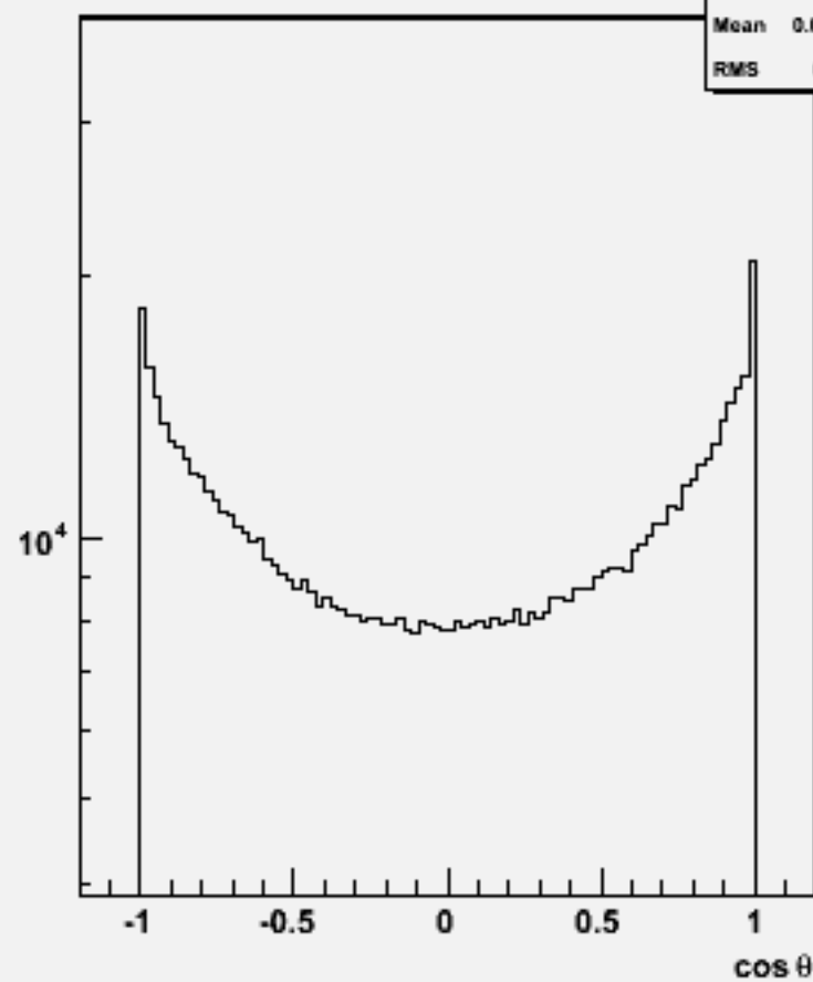
Particle cos \theta : w102521 e1e1ddss_o
