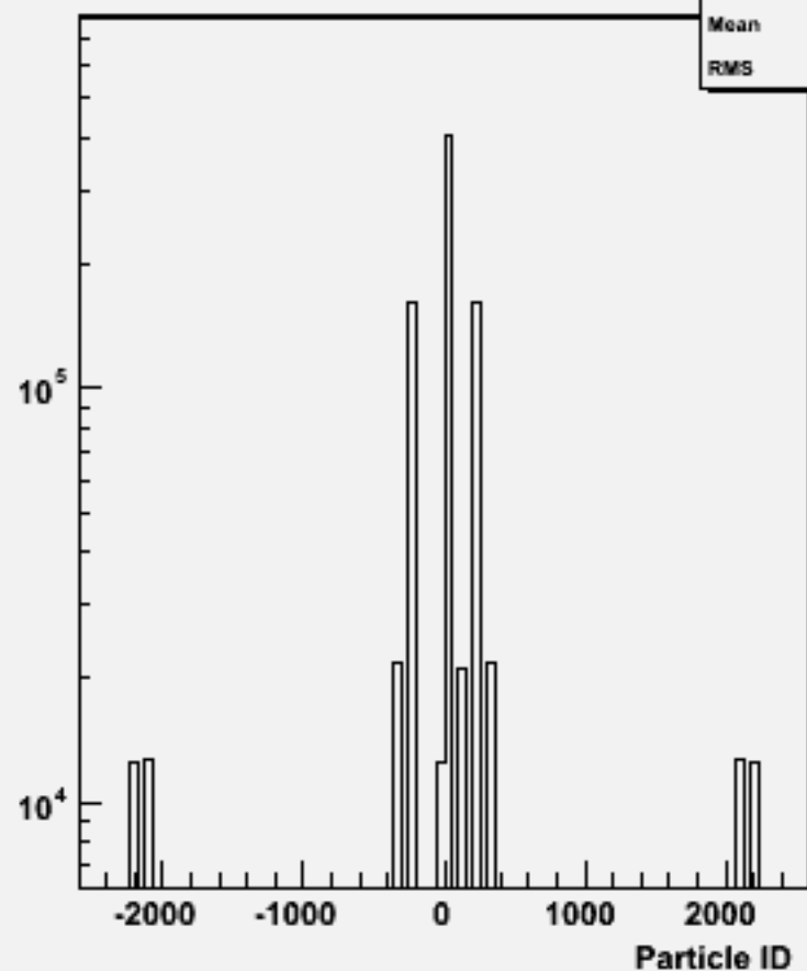
Particle ID : w102520 e1e1ddss_o
