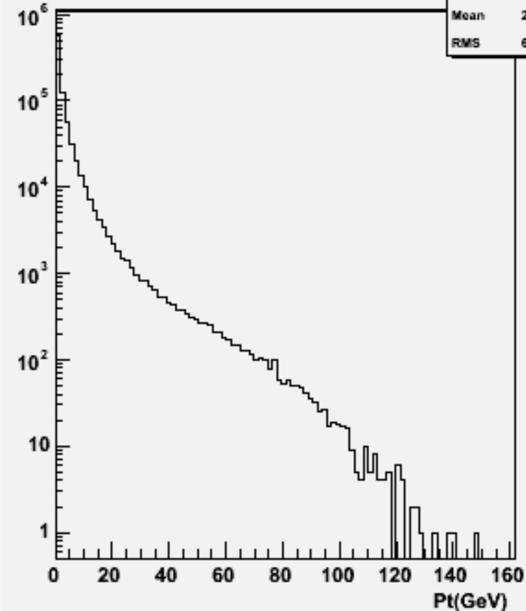
Particle Pt : w102520 e1e1ddss_o
