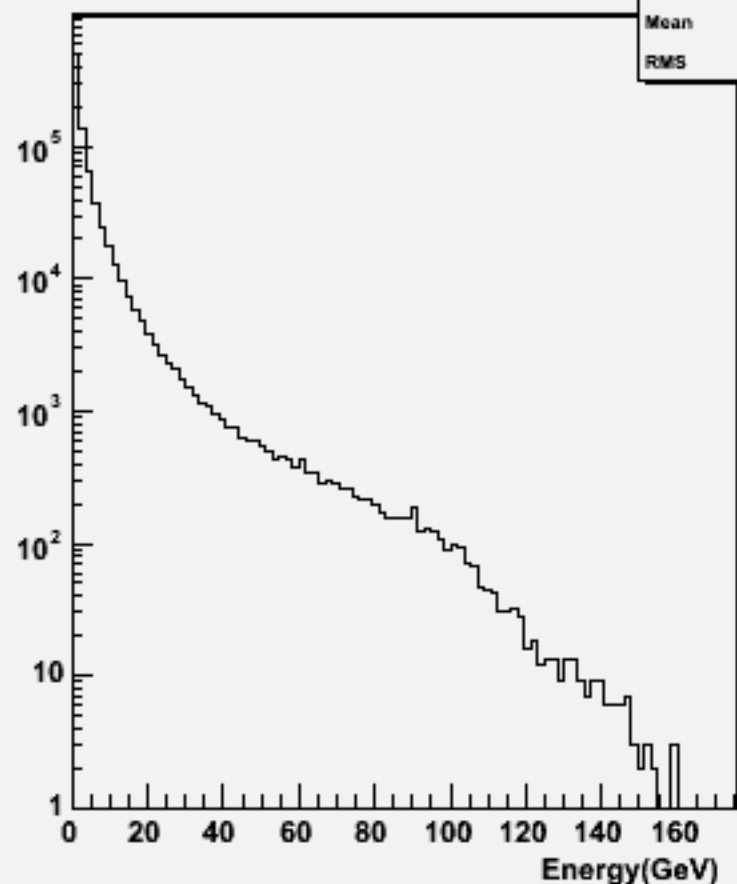
Particle Energy : w102520 e1e1ddss_o
