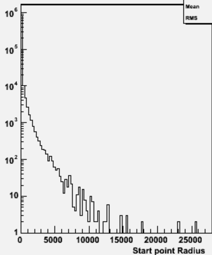
Start point R : w102520 e1e1ddss_o
