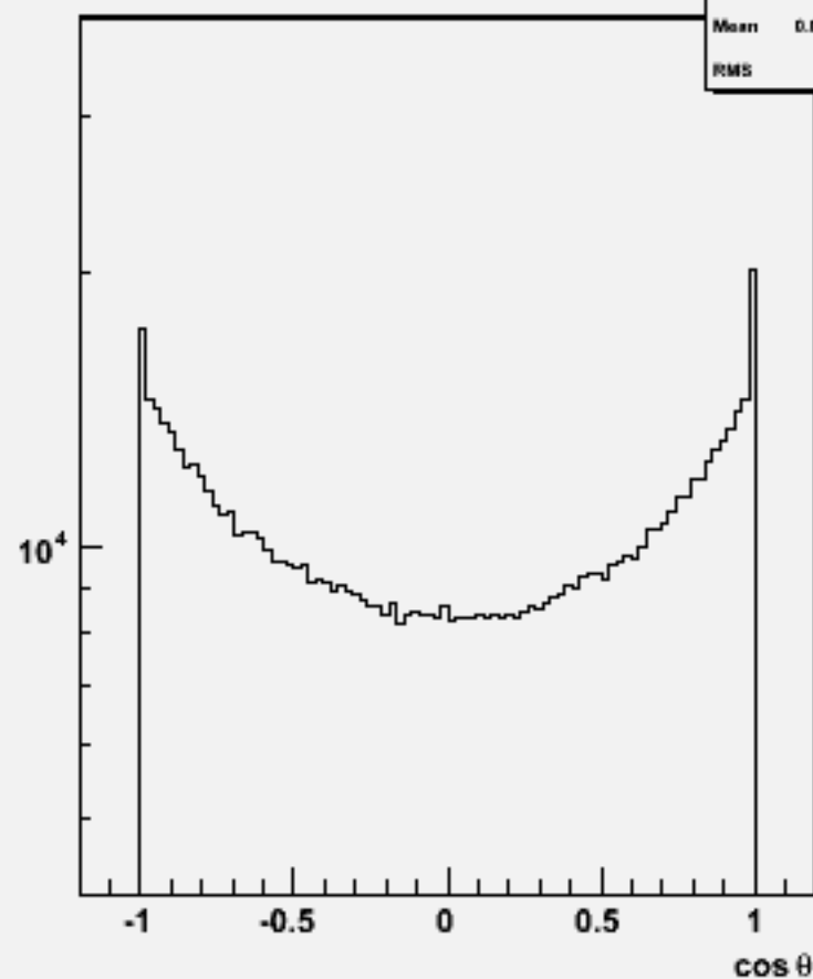
Particle cos \theta : w102520 e1e1ddss_o
