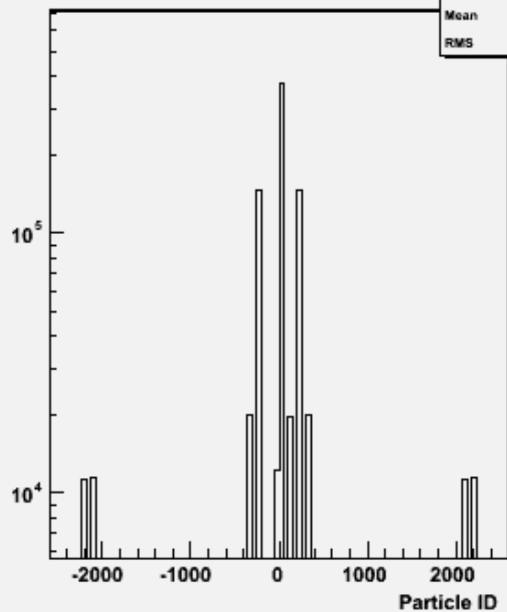
Particle ID : w102519 e1e1ddss_o
