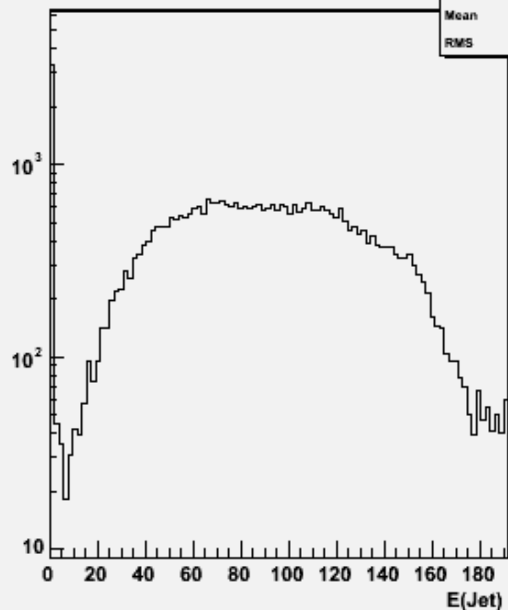
Jet energies(All jets)w102519 e1e1ddss_o
