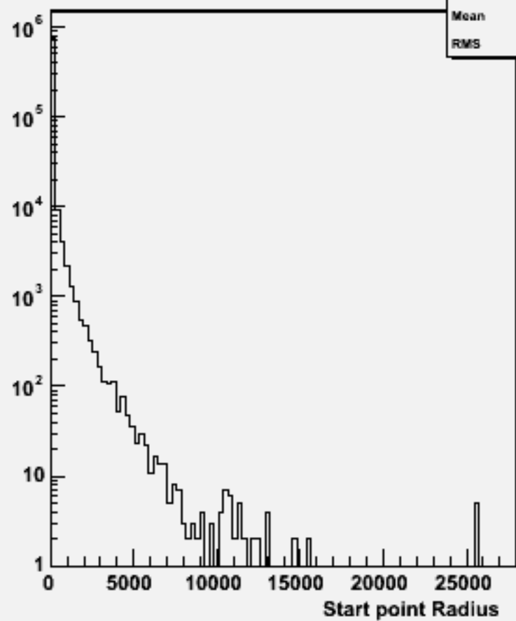
Start point R : w102519 e1e1ddss_o
