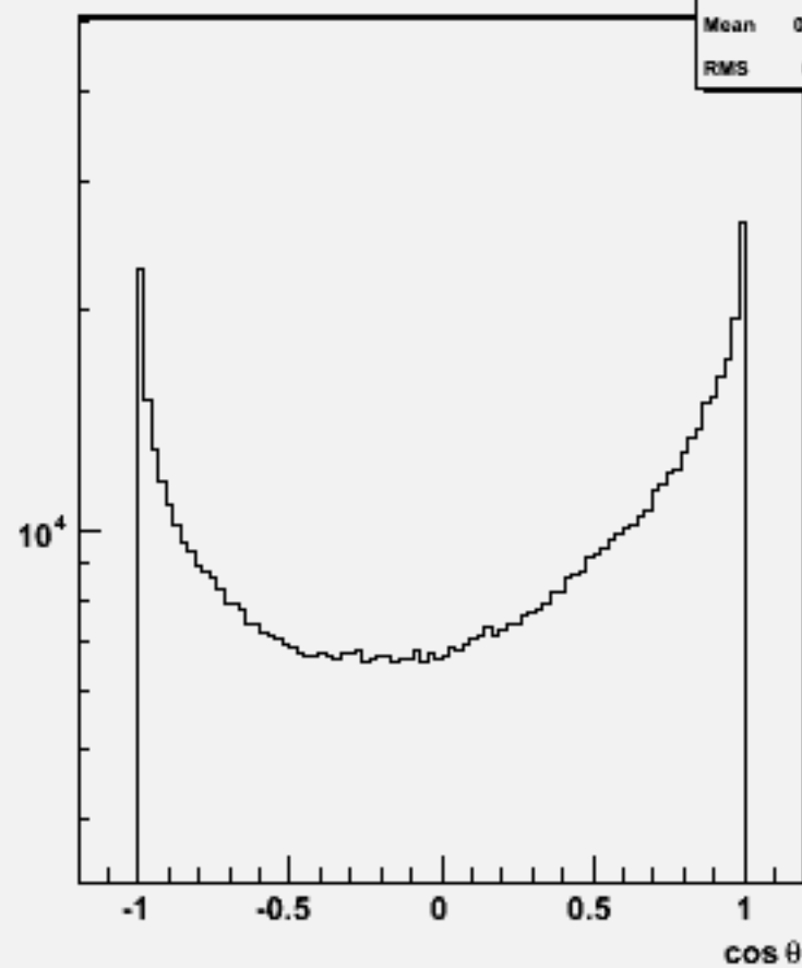
Particle cos \theta : w102519 e1e1ddss_o
