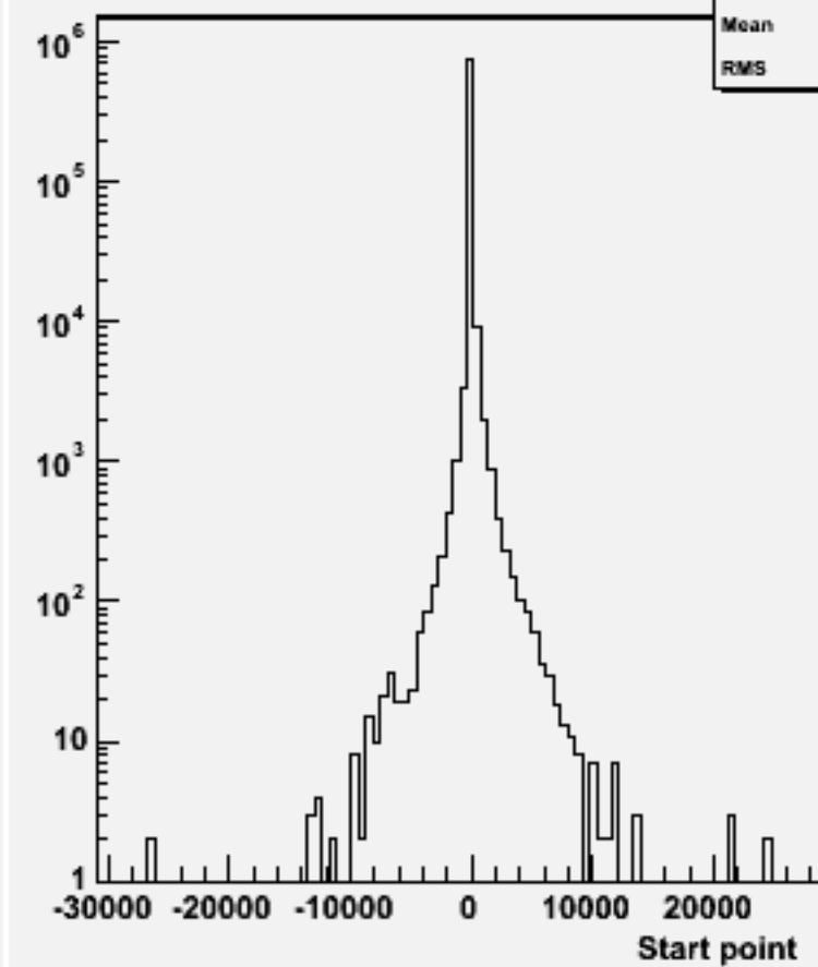
Start point Z : w102519 e1e1ddss_o
