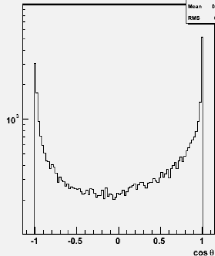
Jet cosθ (All jets)w102519 e1e1ddss_o
