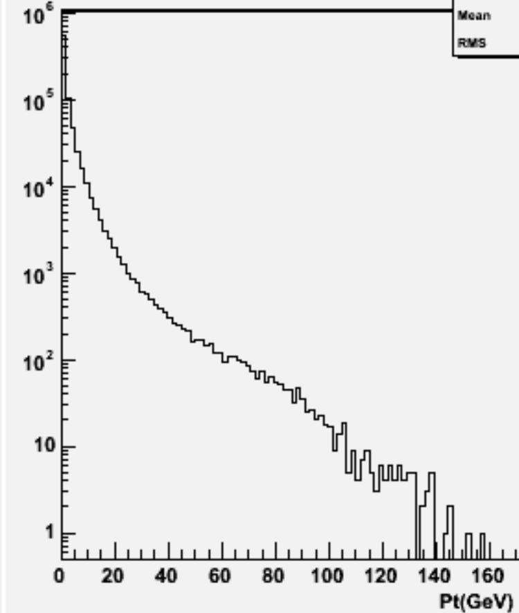
Particle Pt : w102519 e1e1ddss_o
