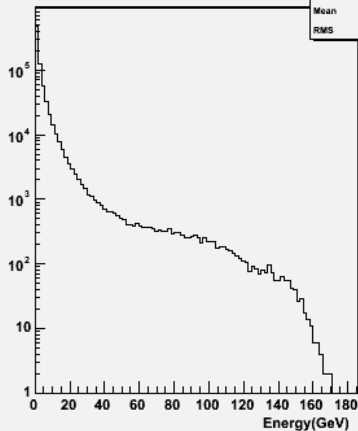
Particle Energy : w102519 e1e1ddss_o
