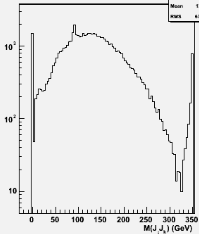
2jets mass(All comb)w102519 e1e1ddss_o
