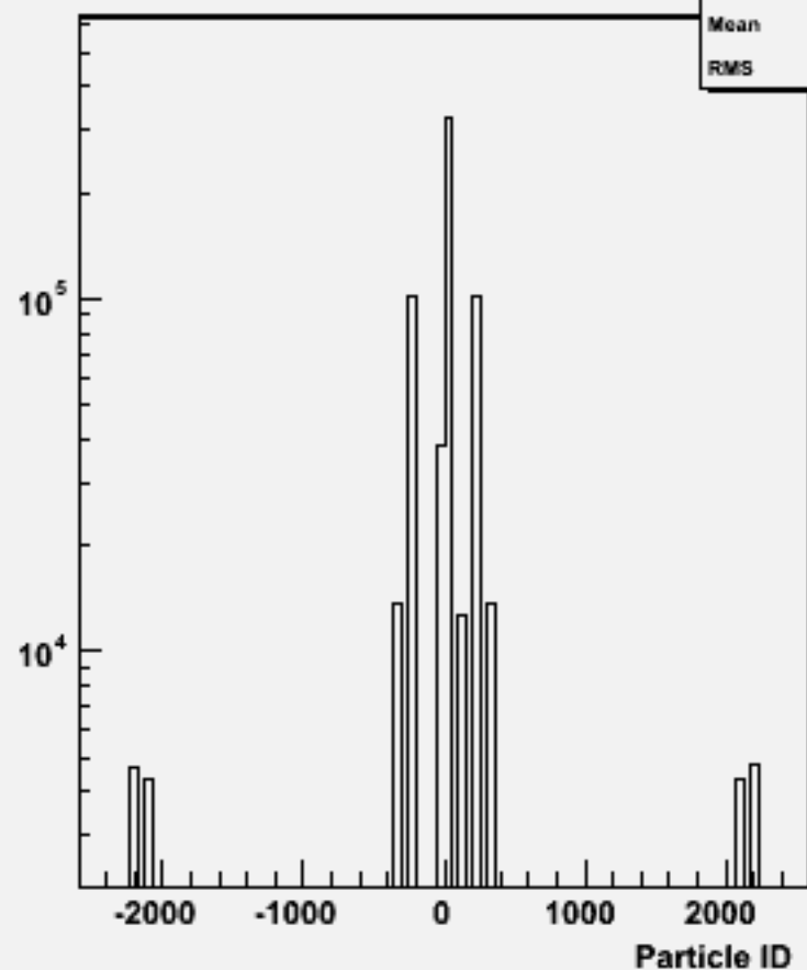
Particle ID : w102512 e1e1e3e3bb_o
