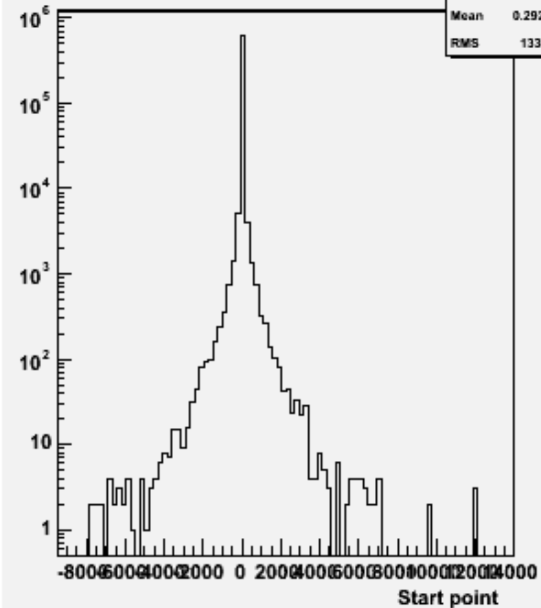
Start point Z : w102512 e1e1e3e3bb_o
