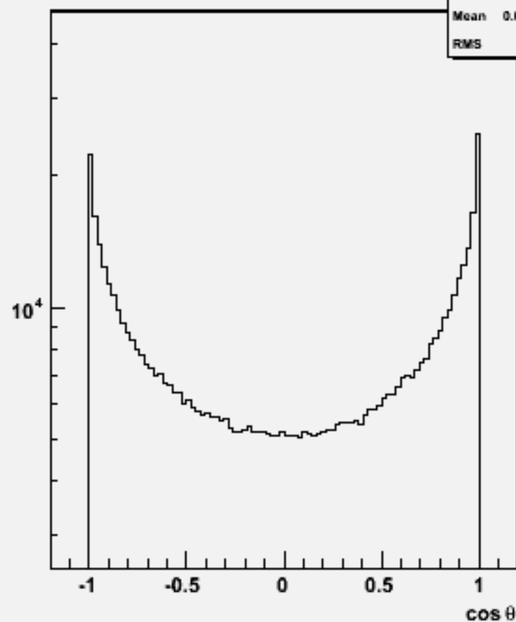
Particle cosθ : w102512 e1e1e3e3bb_o
