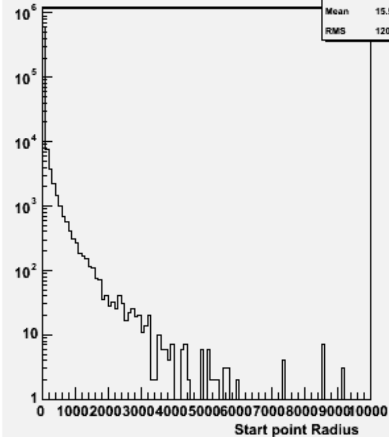
Start point R : w102512 e1e1e3e3bb_o
