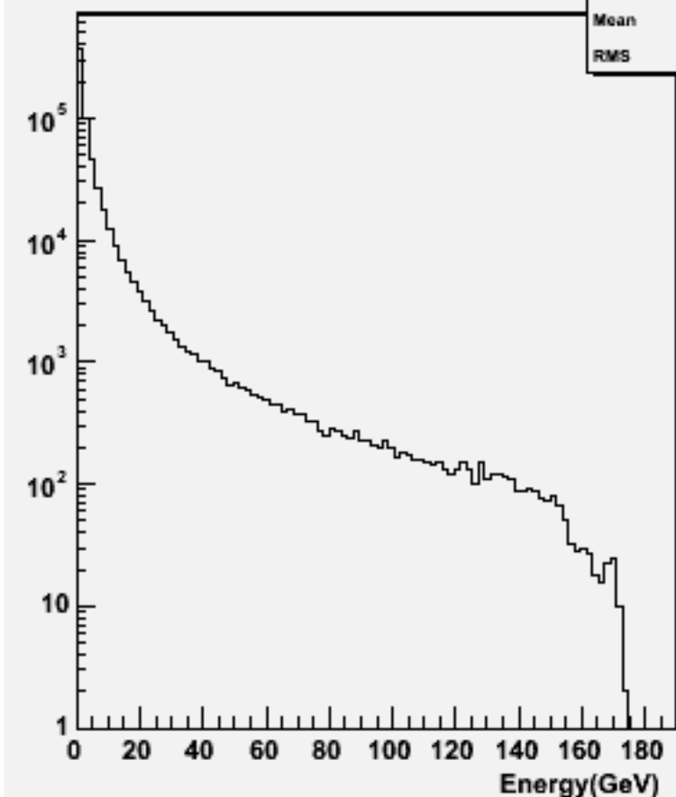
Particle Energy : w102512 e1e1e3e3bb_o
