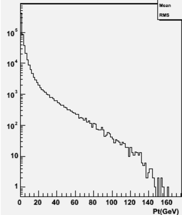
Particle Pt : w102512 e1e1e3e3bb_o
