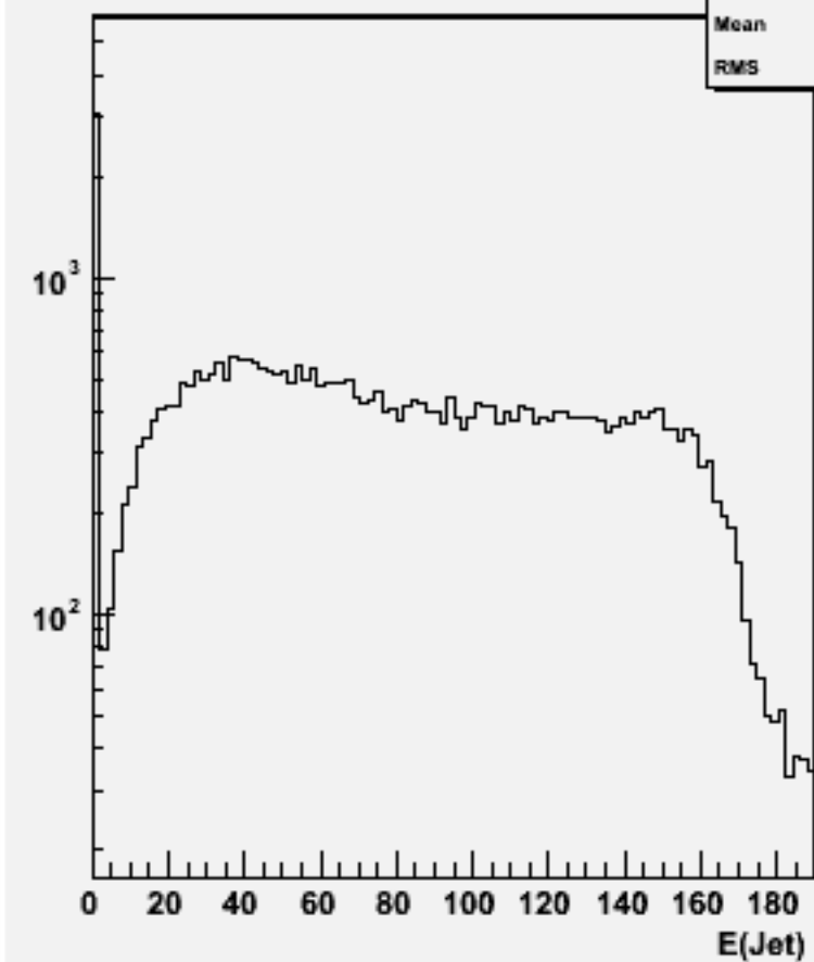
Jet energies(All jets)w102511 e1e1e3e3bb_o
