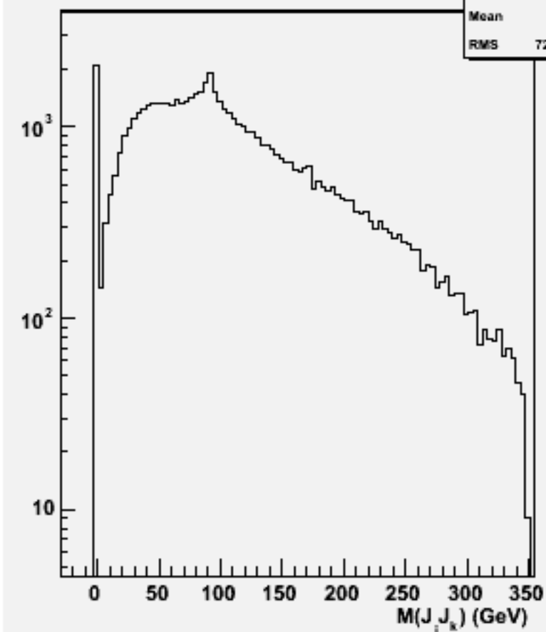
2jets mass(All comb)w102511 e1e1e3e3bb_o
