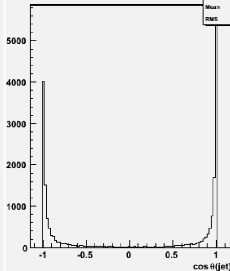
cos \theta for 2-jets :w102511 e1e1e3e3bb_o
