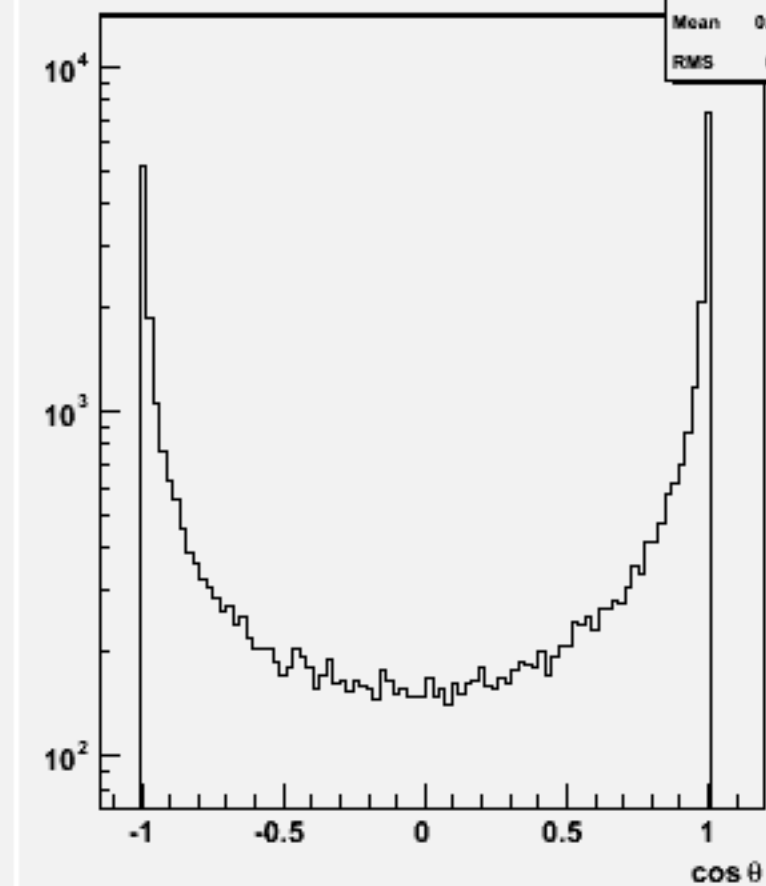
Jet cos \theta (All jets)w102511 e1e1e3e3bb_o
