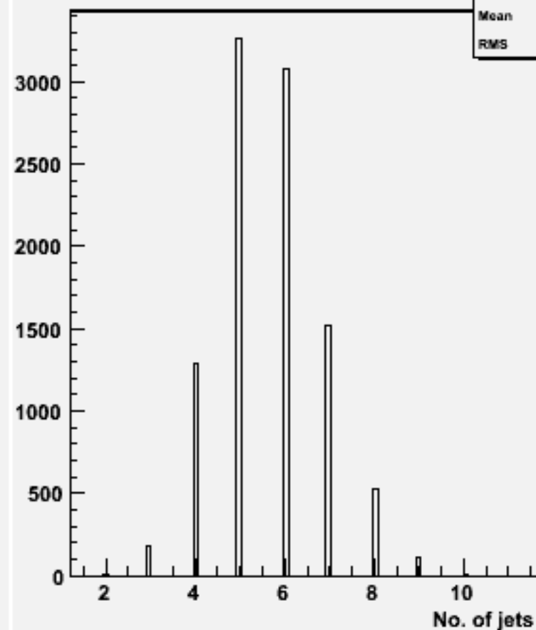
No. jets (ycut=0.001) : w102511 e1e1e3e3bb_o
