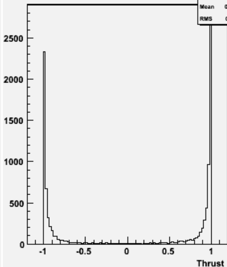
cos \Theta (thrust) w102511 e1e1e3e3bb_o
