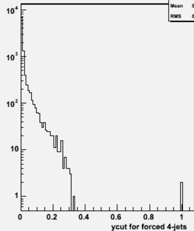
Ycut for 4-jets :w102511 e1e1e3e3bb_o
