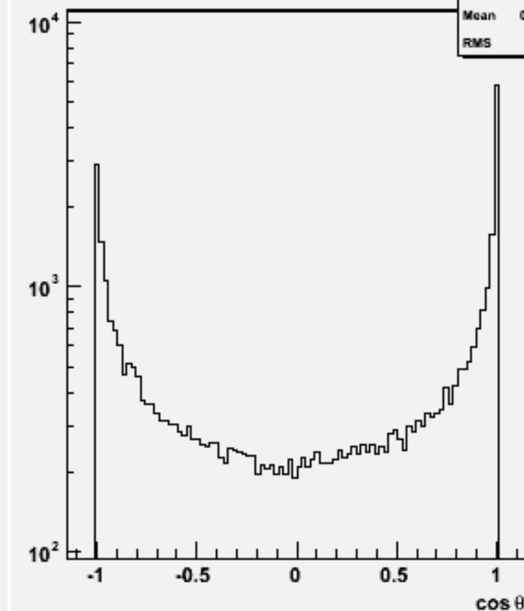
Jet cos \theta (All jets)w102509 e1e1e3e3ss_o
