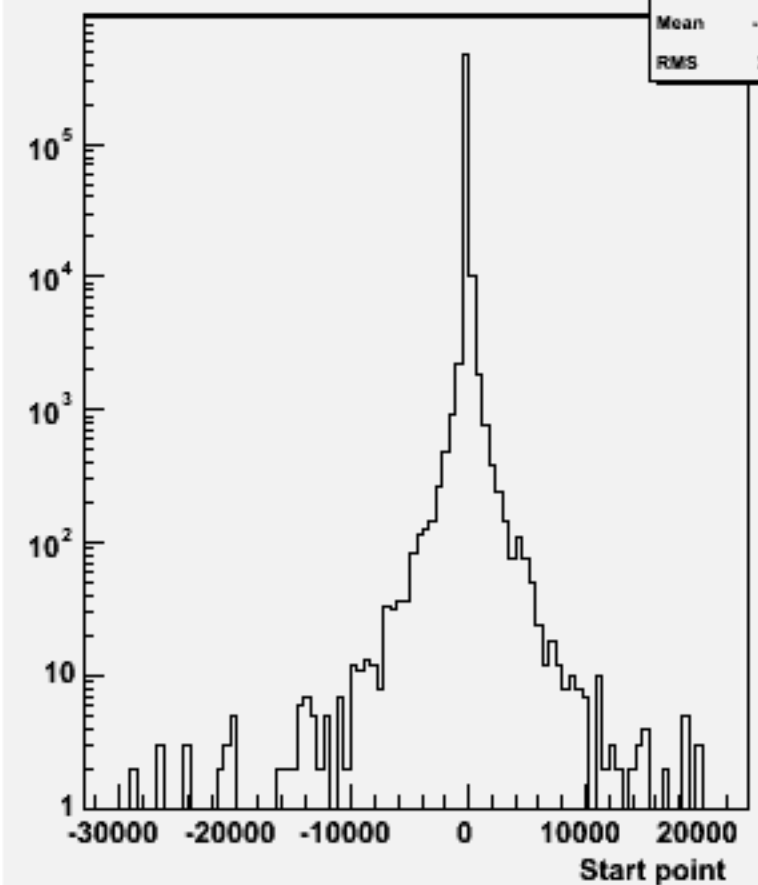
Start point Z : w102509 e1e1e3e3ss_o
