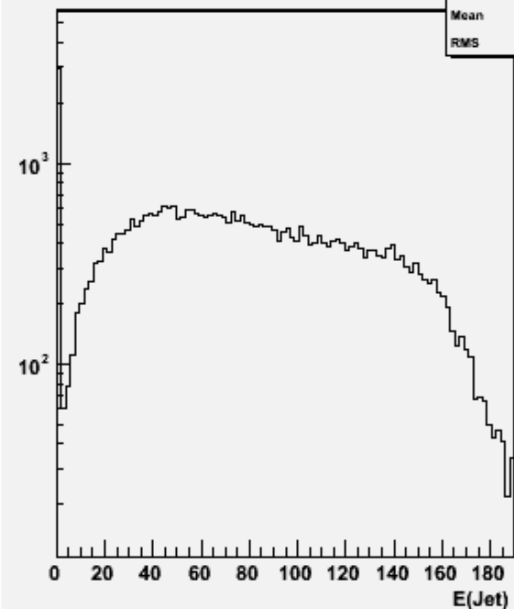
Jet energies(All jets)w102509 e1e1e3e3ss_o
