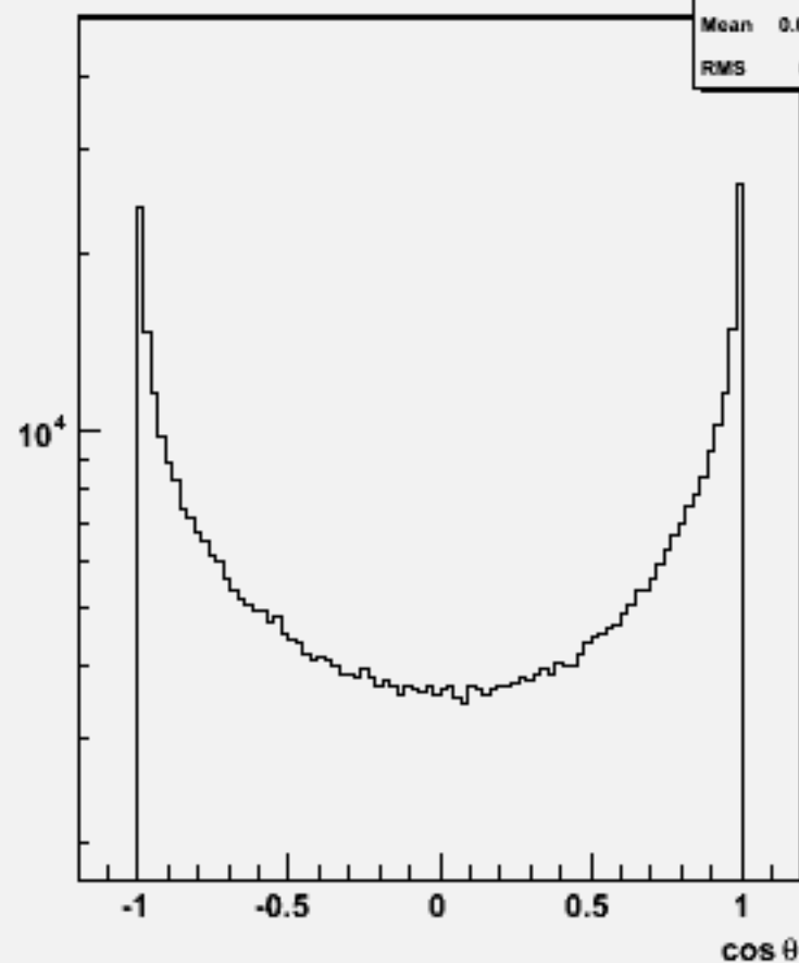
Particle cos \theta : w102509 e1e1e3e3ss_o
