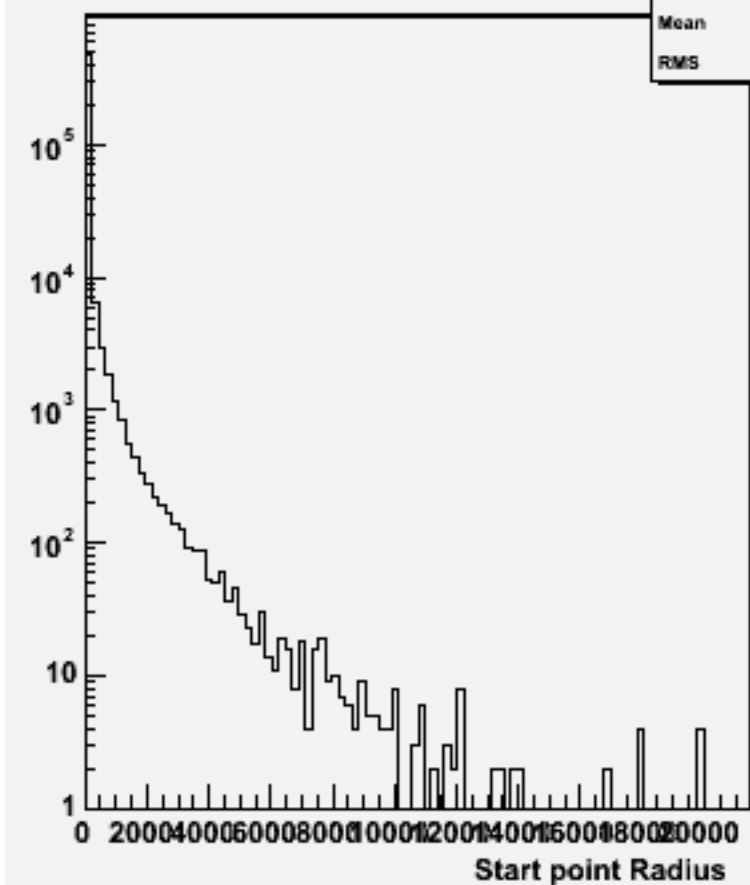
Start point R : w102509 e1e1e3e3ss_o
