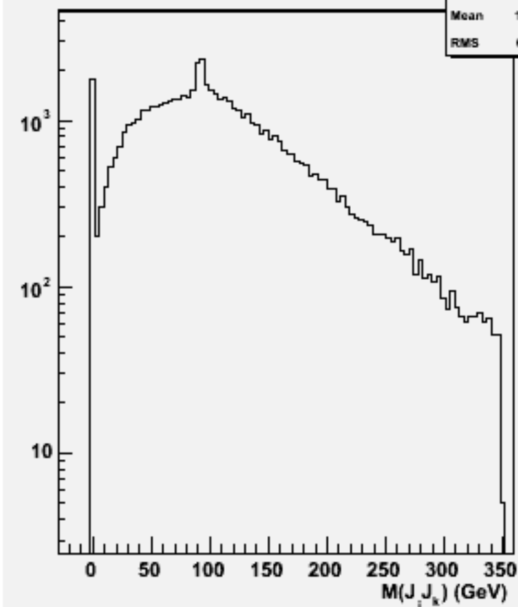
2jets mass(All comb)w102509 e1e1e3e3ss_o
