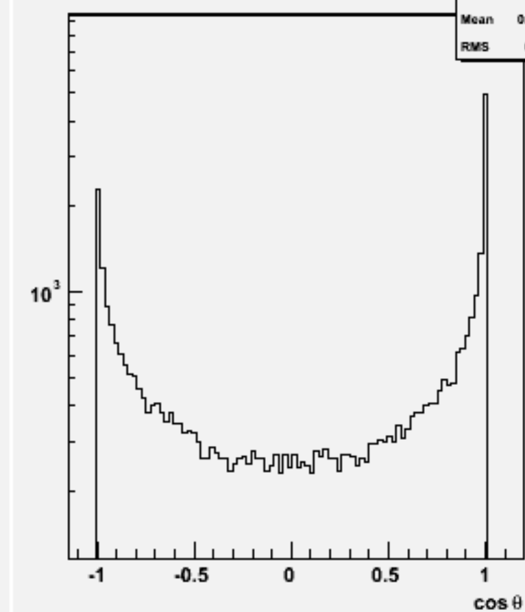
Jet cos \theta (All jets)w102508 e1e1e3e3ss_o
