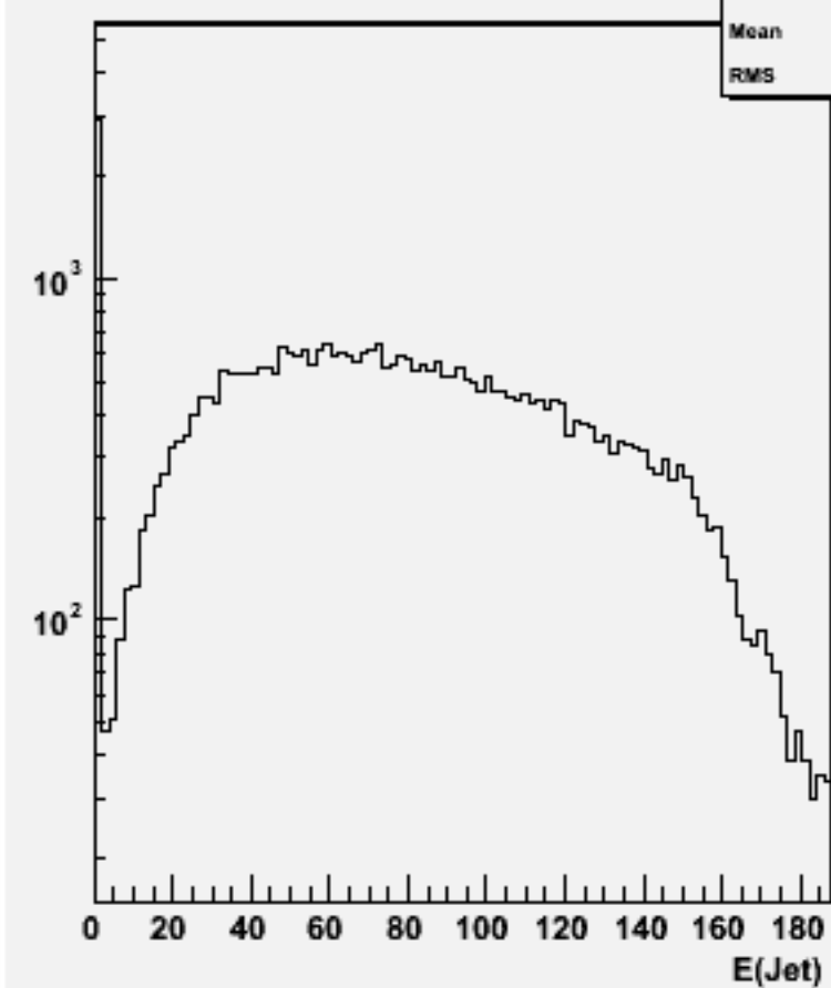
Jet energies(All jets)w102508 e1e1e3e3ss_o
