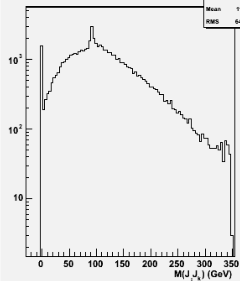
2jets mass(All comb)w102508 e1e1e3e3ss_o
