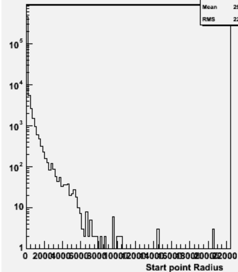
Start point R : w102507 e1e1e3e3ss_o
