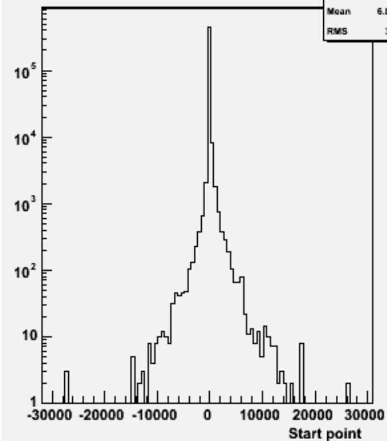
Start point Z : w102507 e1e1e3e3ss_o
