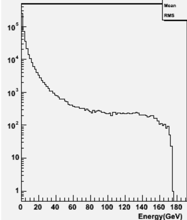
Start point R : w102507 e1e1e3e3ss_o
