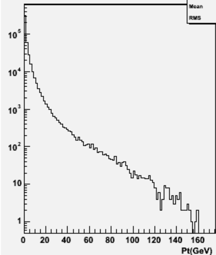
Start point Z : w102507 e1e1e3e3ss_o
