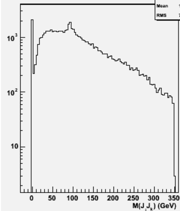
2jets mass(All comb)w102507 e1e1e3e3ss_o
