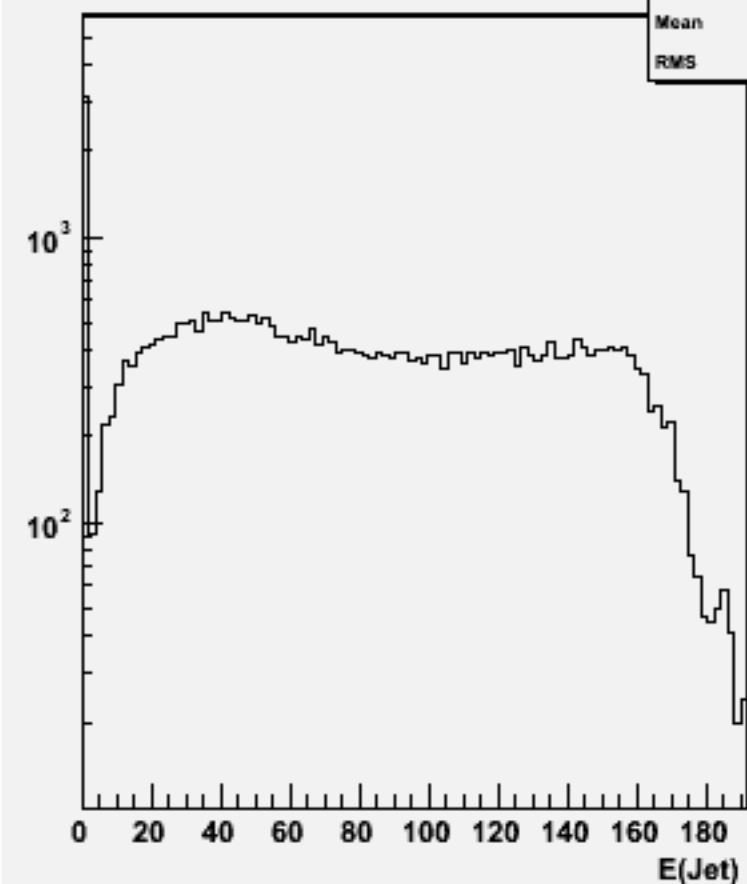
Jet energies(All jets)w102507 e1e1e3e3ss_o
