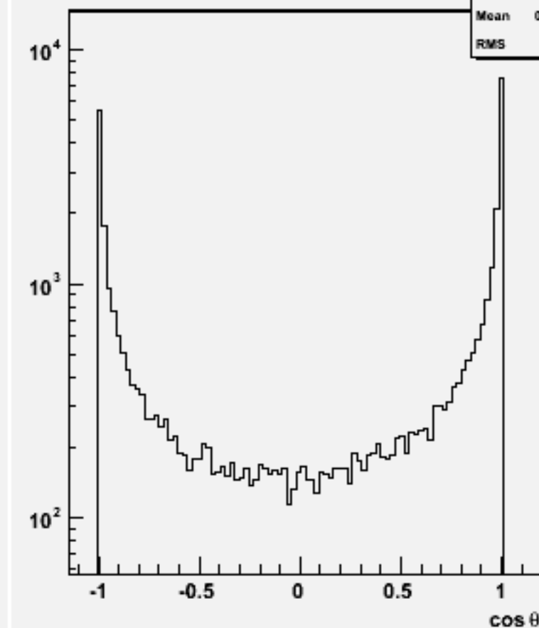
Jet cos \theta (All jets)w102507 e1e1e3e3ss_o
