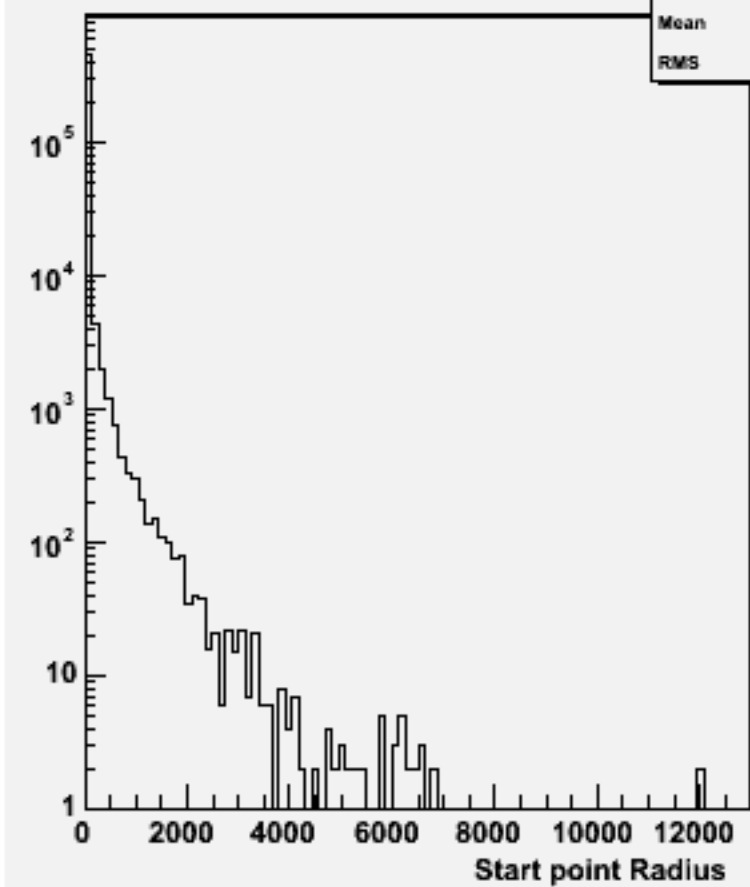
Start point R : w102506 e1e1e3e3dd_o
