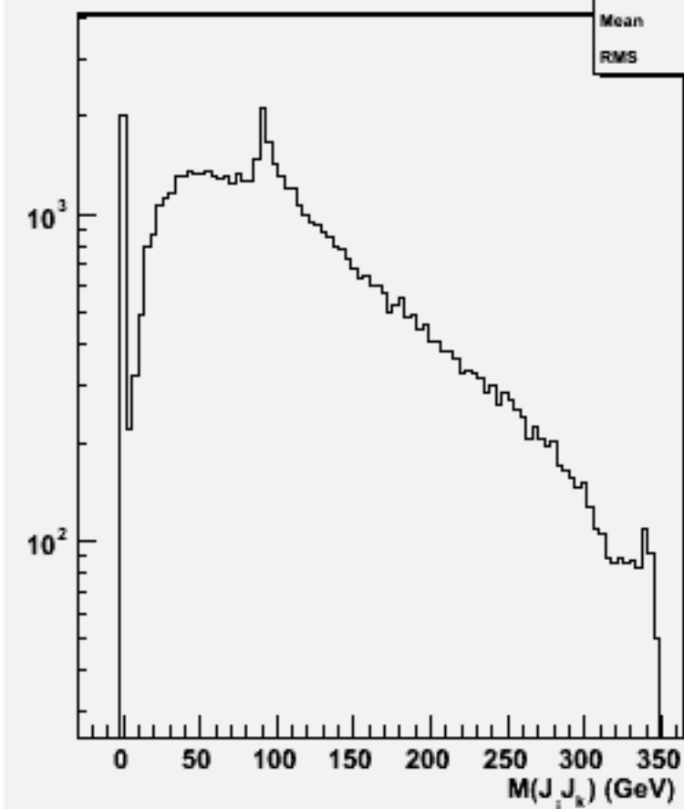
2jets mass(All comb)w102506 e1e1e3e3dd_o
