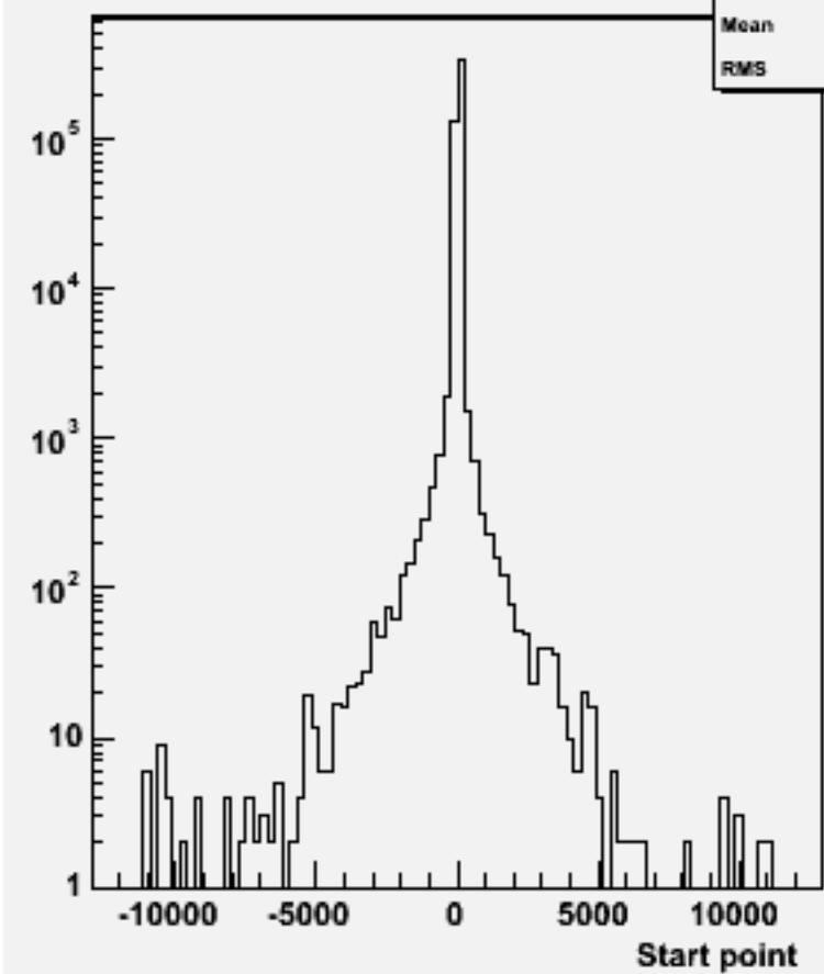
Start point Z : w102506 e1e1e3e3dd_o
