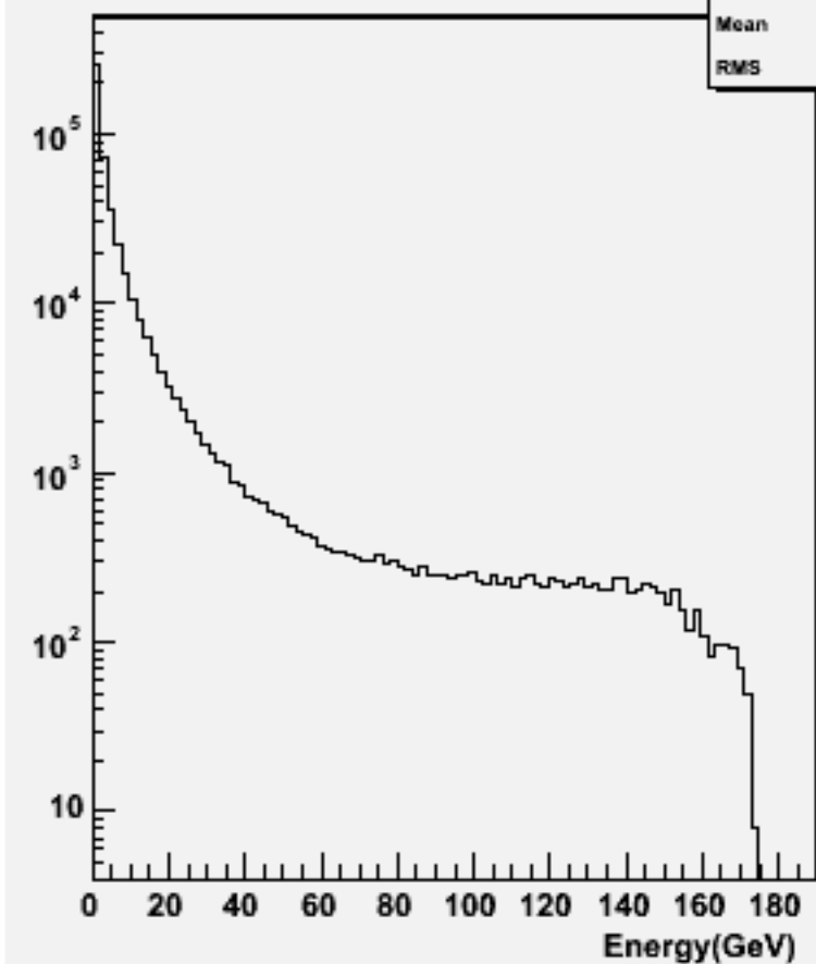
Particle Energy : w102506 e1e1e3e3dd_o
