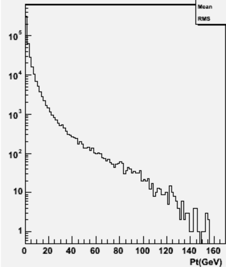
Particle Pt : w102506 e1e1e3e3dd_o
