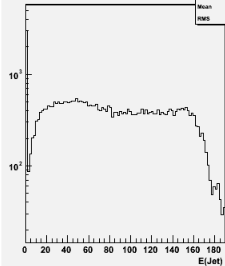
Jet energies(All jets)w102506 e1e1e3e3dd_o
