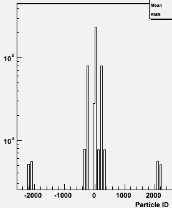
Particle ID : w102506 e1e1e3e3dd_o
