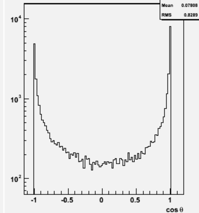
Jet cos \theta (All jets)w102506 e1e1e3e3dd_o
