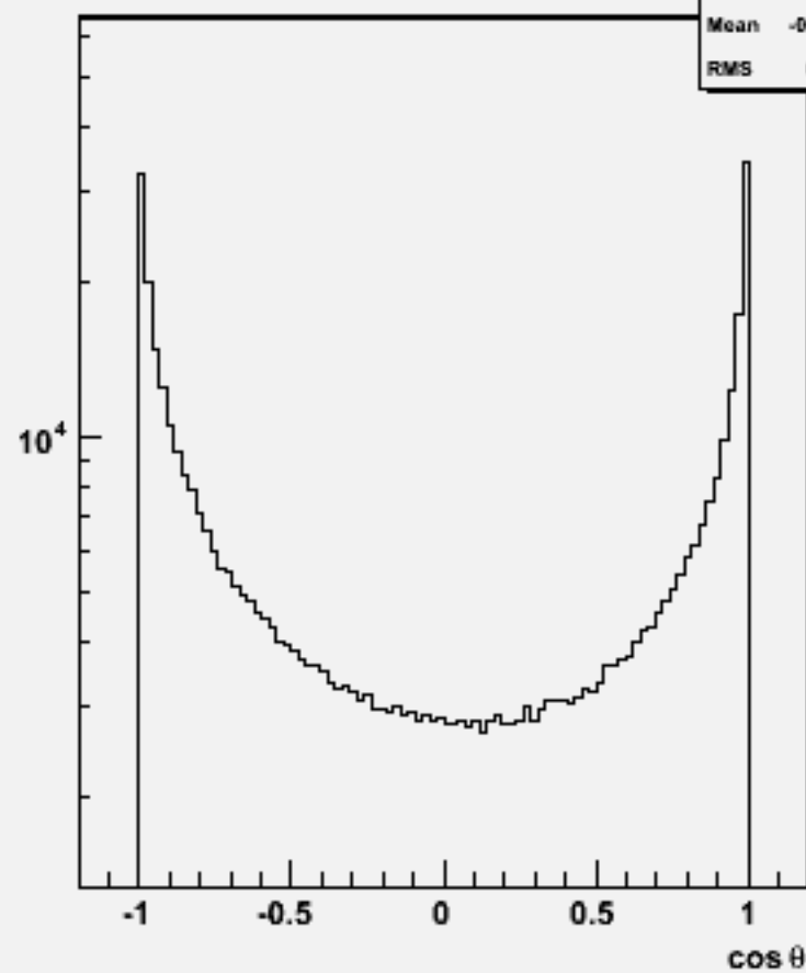
Particle cosθ : w102506 e1e1e3e3dd_o
