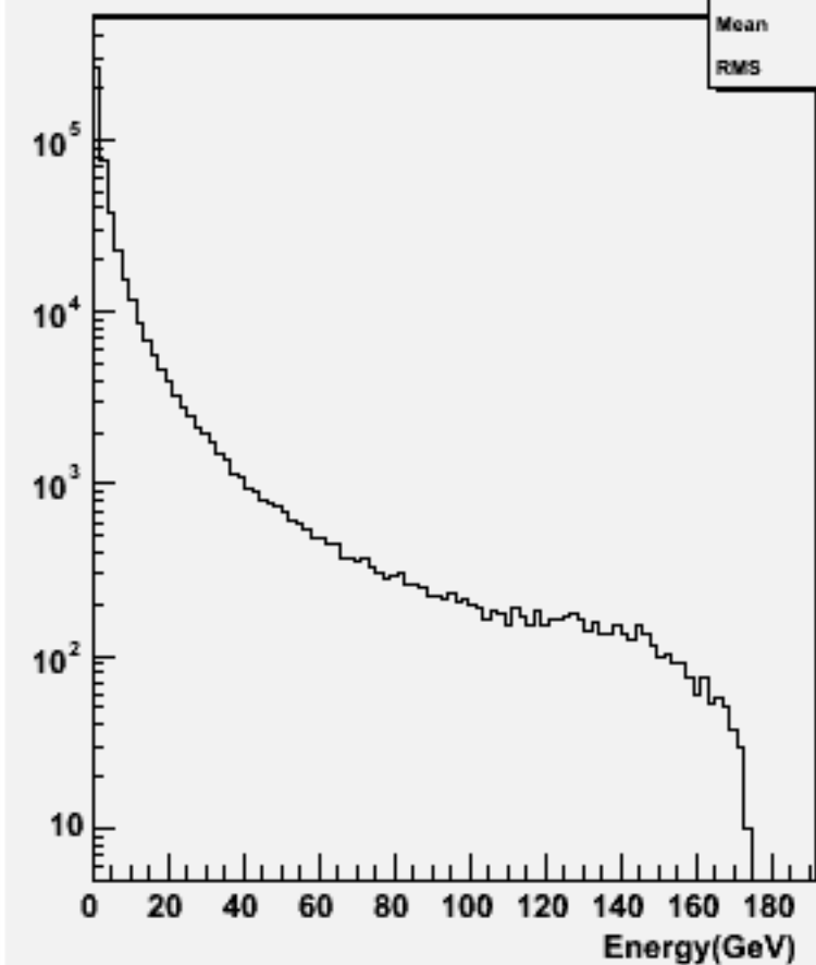
Particle Energy : w102505 e1e1e3e3dd_o
