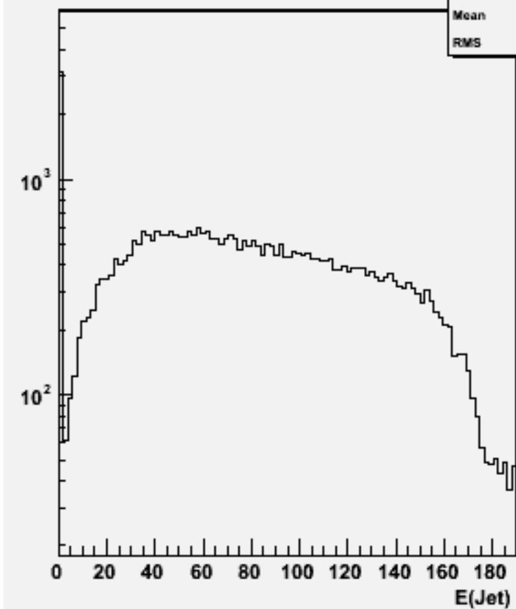
Jet energies(All jets)w102505 e1e1e3e3dd_o
