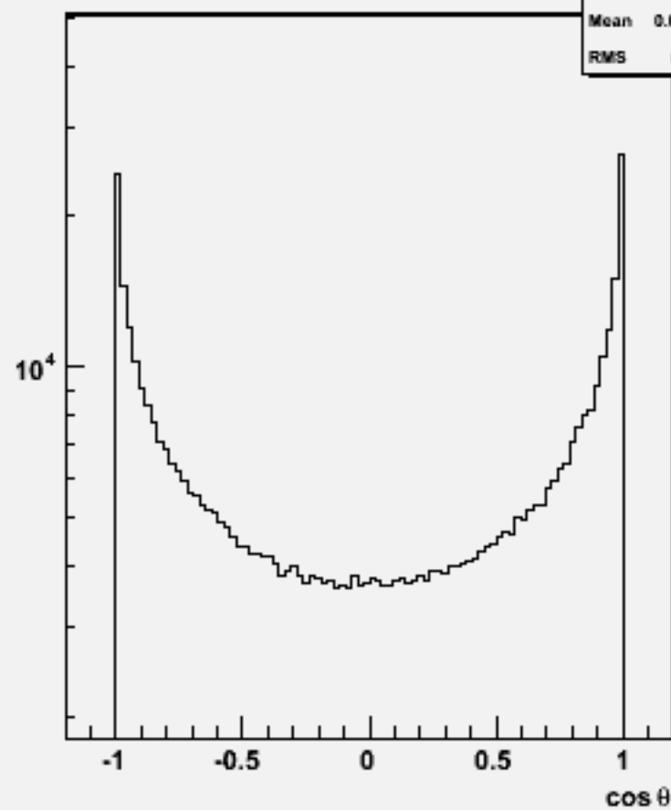
Particle cos \theta : w102505 e1e1e3e3dd_o
