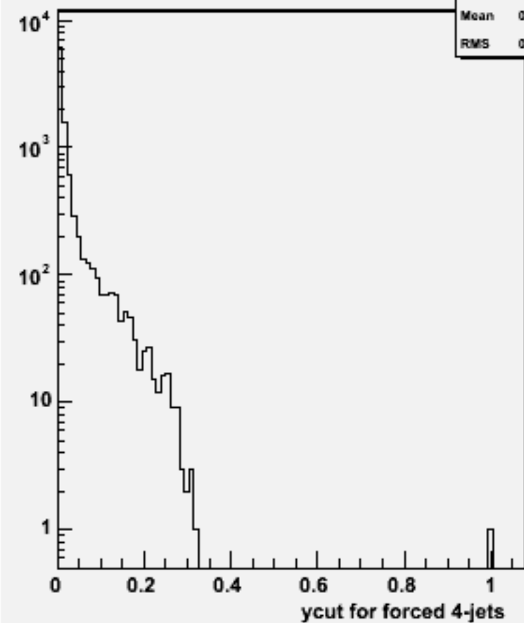
Ycut for 4-jets :w102505 e1e1e3e3dd_o
