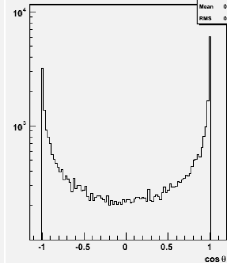
Jet cos \theta (All jets)w102505 e1e1e3e3dd_o
