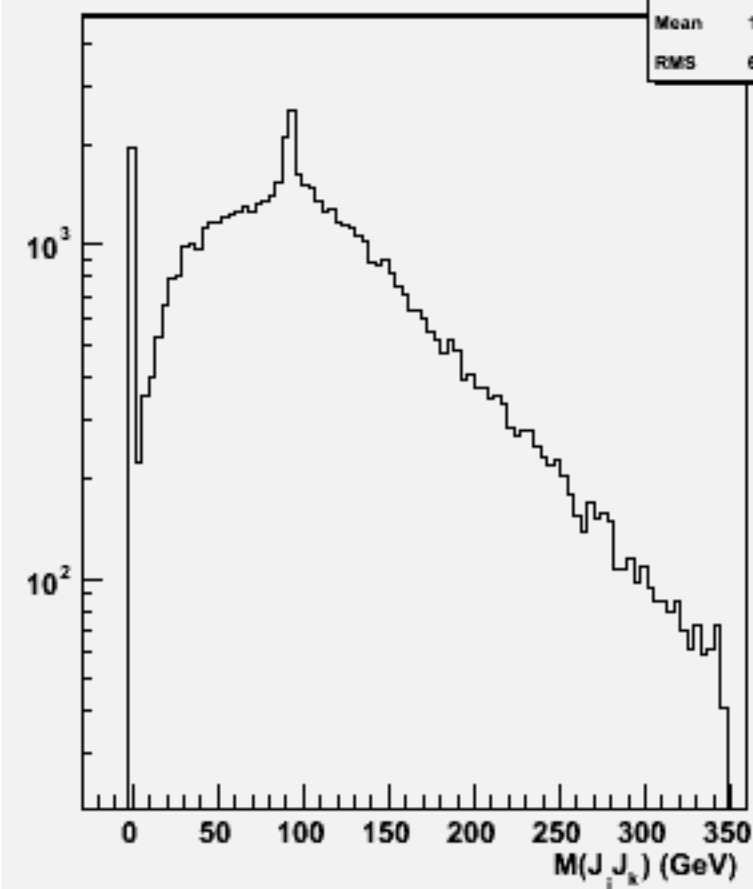
2jets mass(All comb)w102505 e1e1e3e3dd_o
