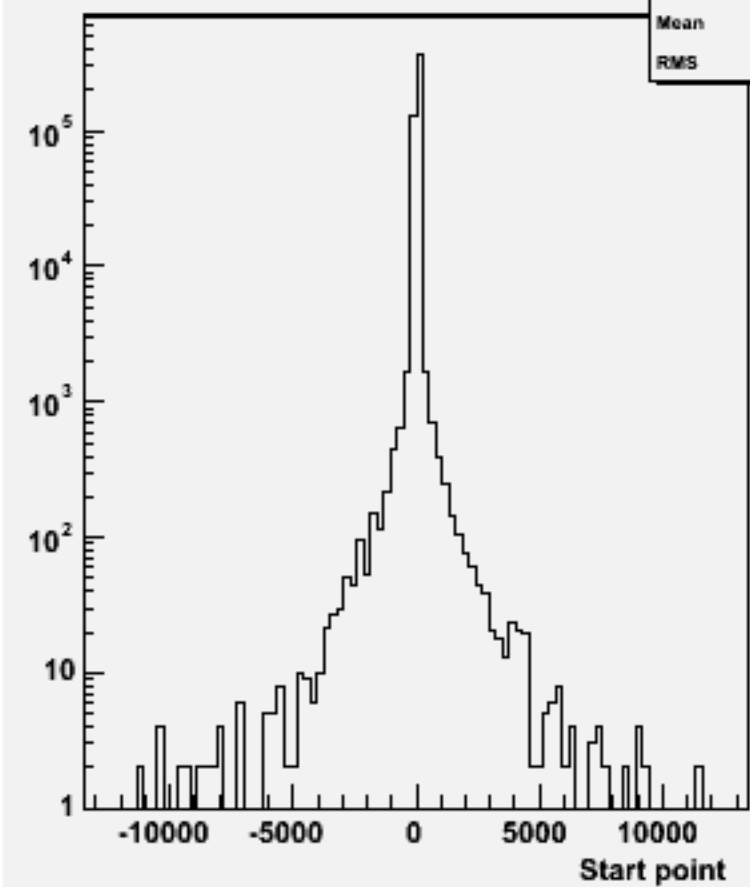
Start point Z : w102505 e1e1e3e3dd_o
