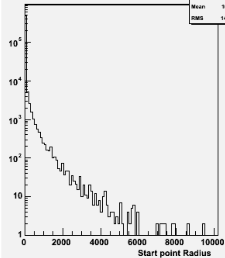
Start point R : w102505 e1e1e3e3dd_o
