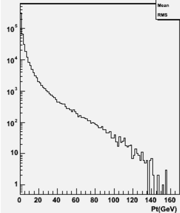
Particle Pt : w102505 e1e1e3e3dd_o
