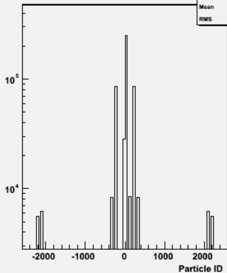
Particle ID : w102505 e1e1e3e3dd_o
