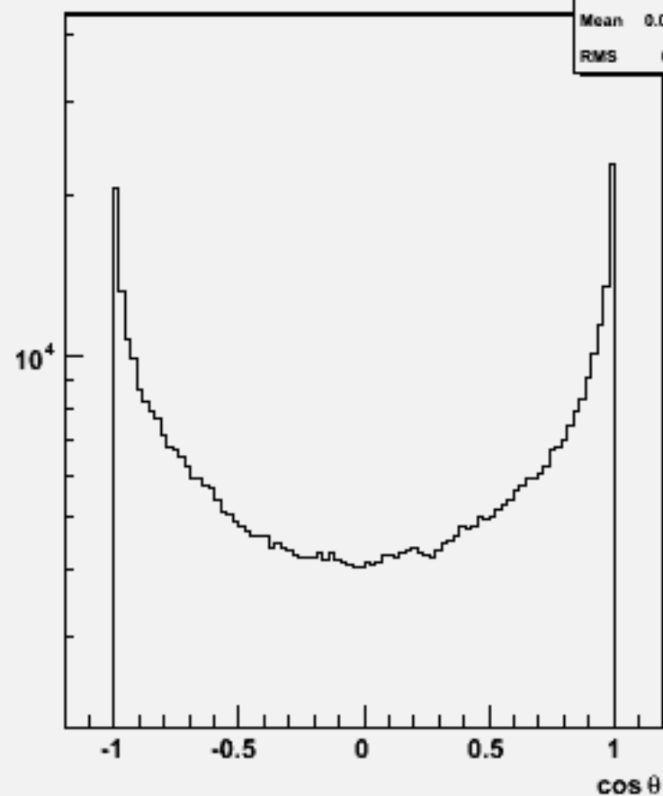
Particle cos \theta : w102504 e1e1e3e3dd_o
