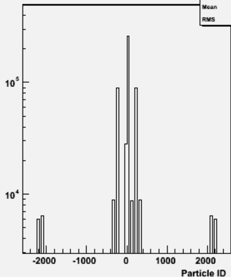
Particle ID : w102504 e1e1e3e3dd_o
