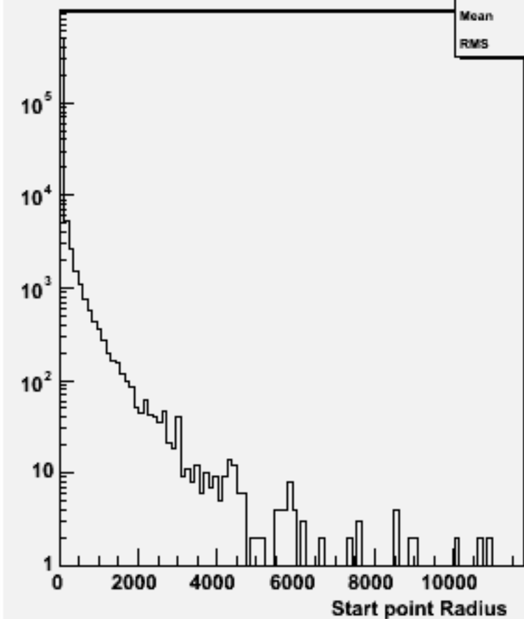
Start point R : w102504 e1e1e3e3dd_o
