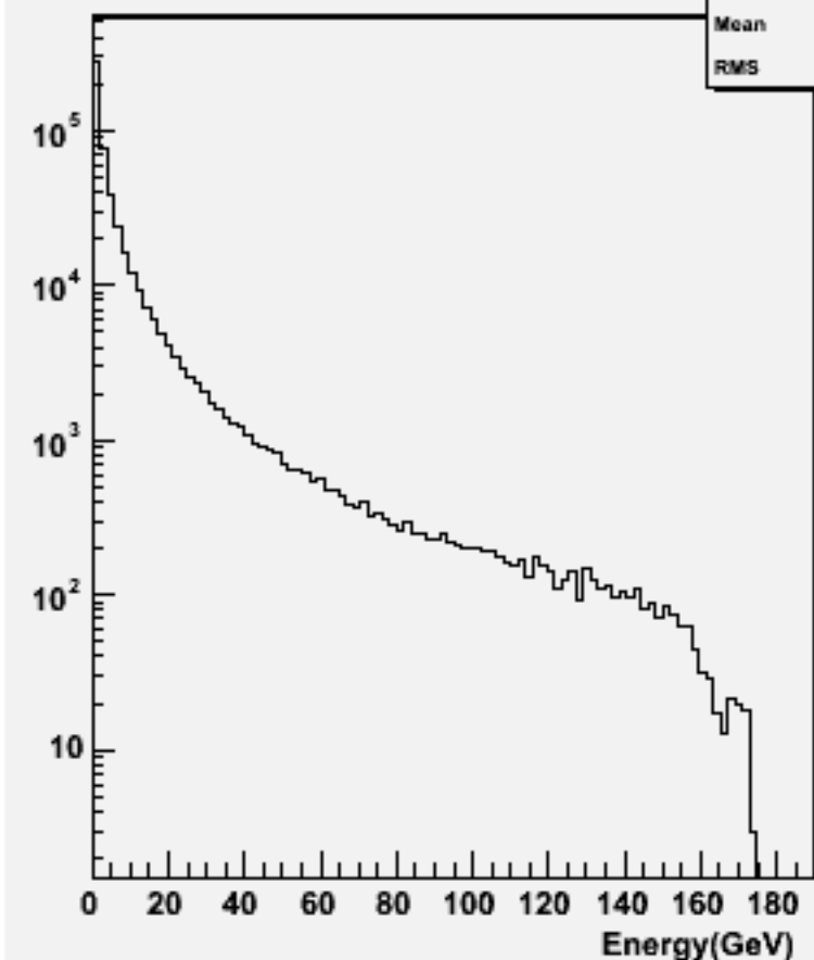
Particle Energy : w102504 e1e1e3e3dd_o
