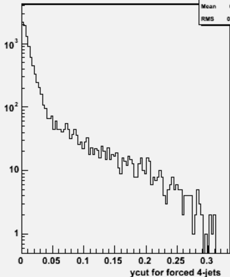
Ycut for 4-jets :w102504 e1e1e3e3dd_o
