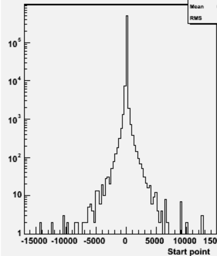
Start point Z : w102504 e1e1e3e3dd_o
