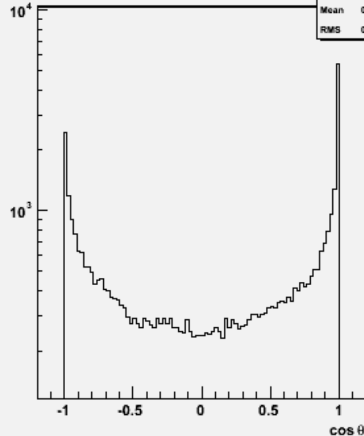
Jet cos \theta (All jets)w102504 e1e1e3e3dd_o
