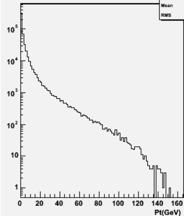
Particle Pt : w102504 e1e1e3e3dd_o
