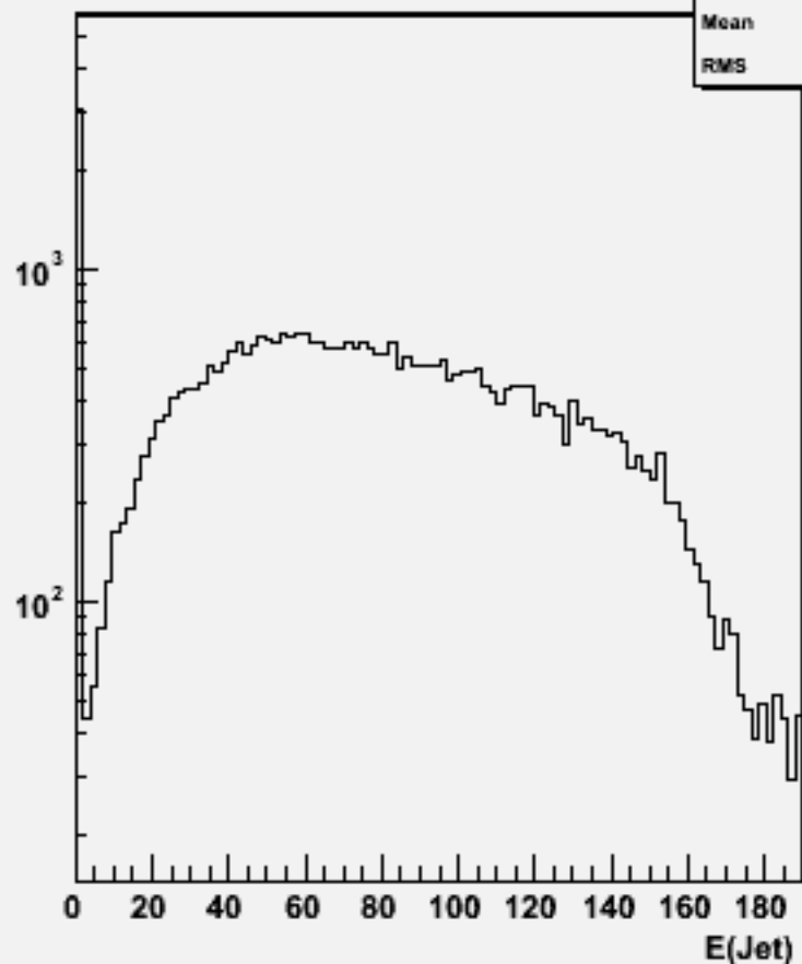
Jet energies(All jets)w102504 e1e1e3e3dd_o
