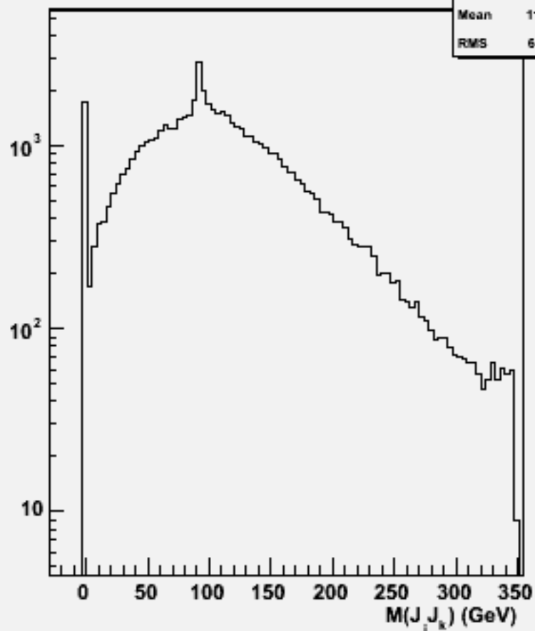
2jets mass(All comb)w102504 e1e1e3e3dd_o
