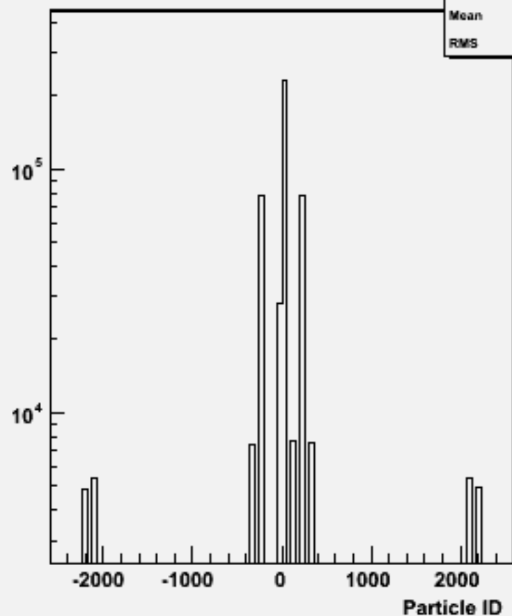
Particle ID : w102503 e1e1e3e3dd_o
