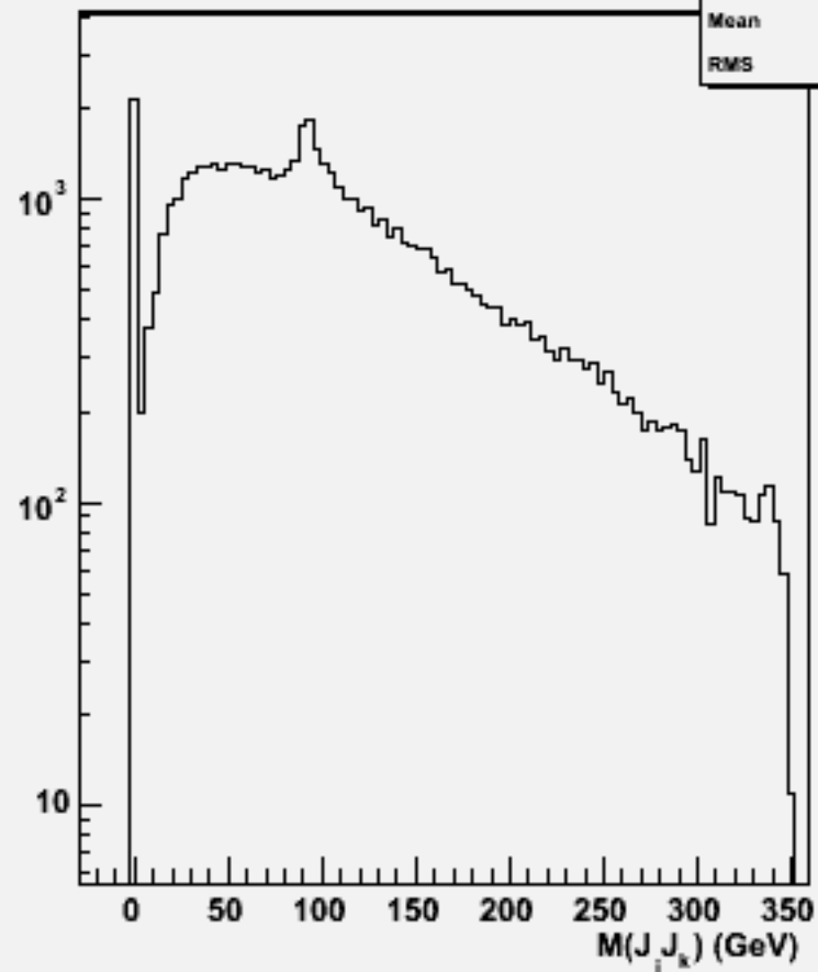
2jets mass(All comb)w102503 e1e1e3e3dd_o
