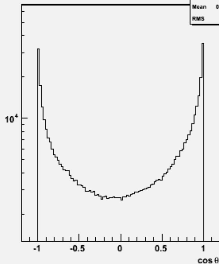
Particle cosθ : w102503 e1e1e3e3dd_o
