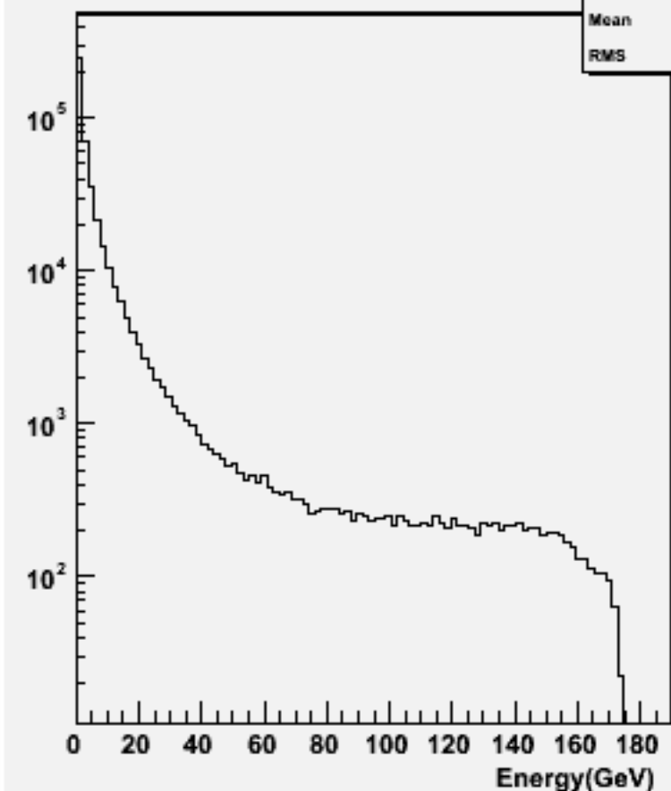
Particle Energy : w102503 e1e1e3e3dd_o
