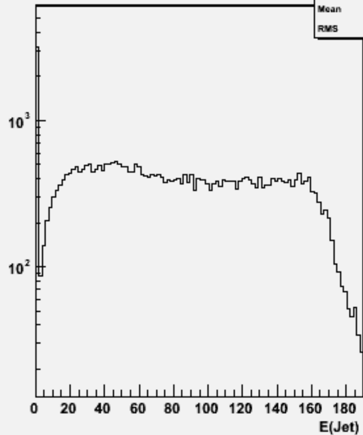
Jet energies(All jets)w102503 e1e1e3e3dd_o
