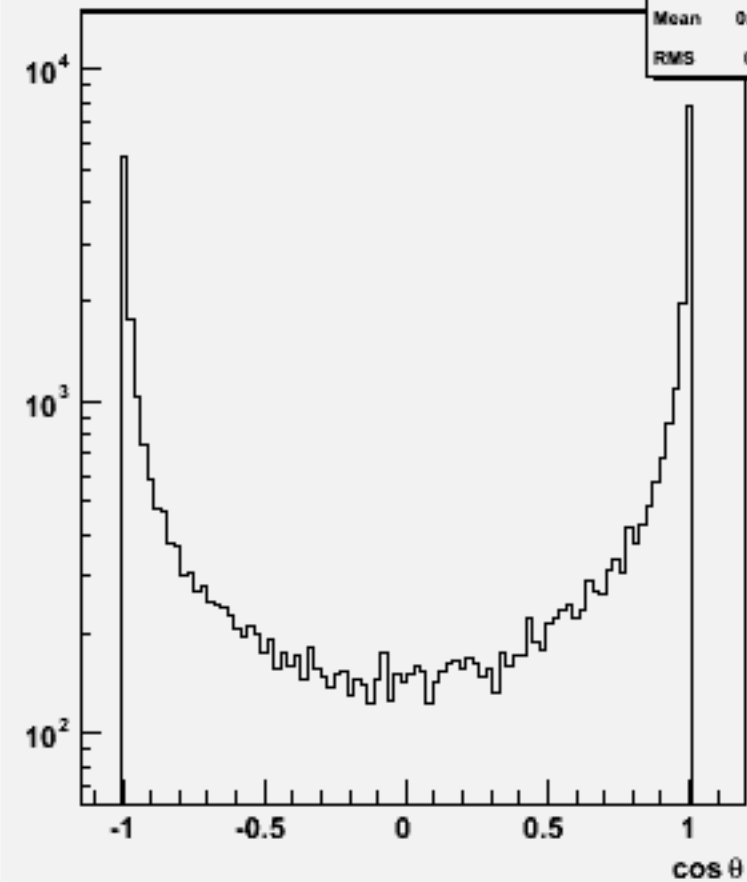
Jet cos \theta (All jets)w102503 e1e1e3e3dd_o
