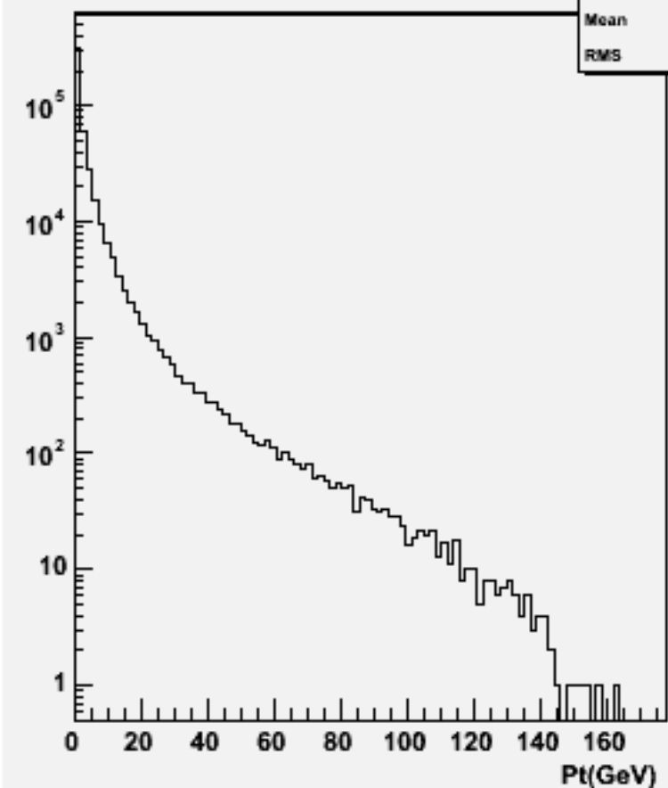
Particle Pt : w102503 e1e1e3e3dd_o
