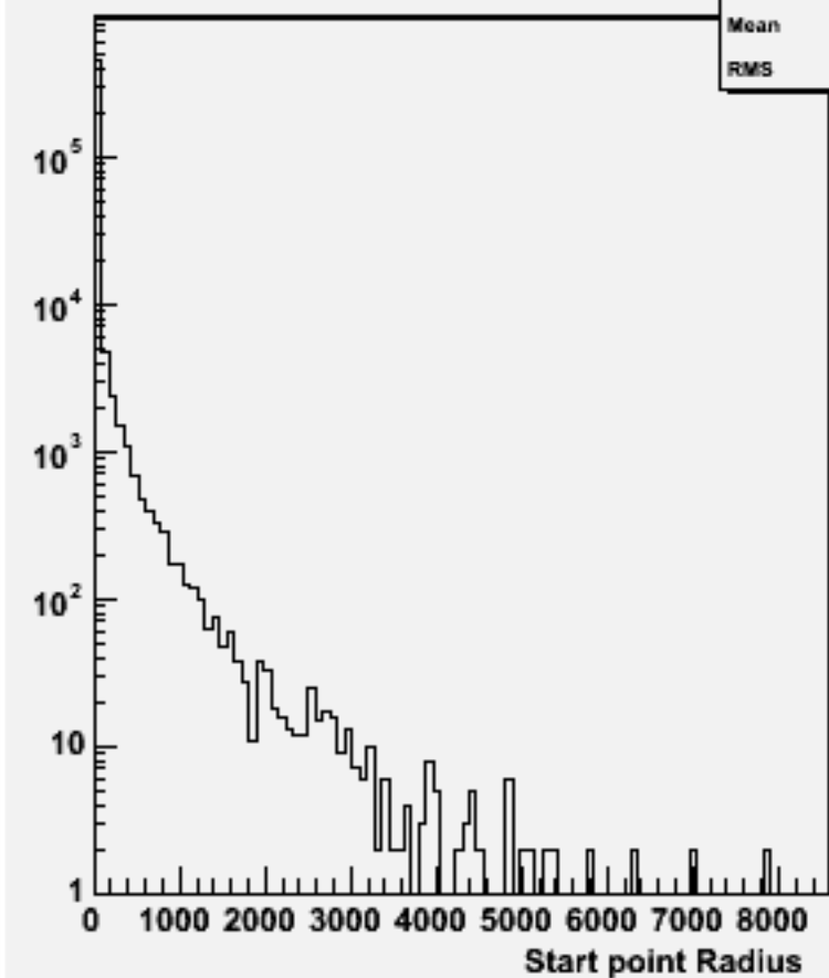
Start point R : w102503 e1e1e3e3dd_o
