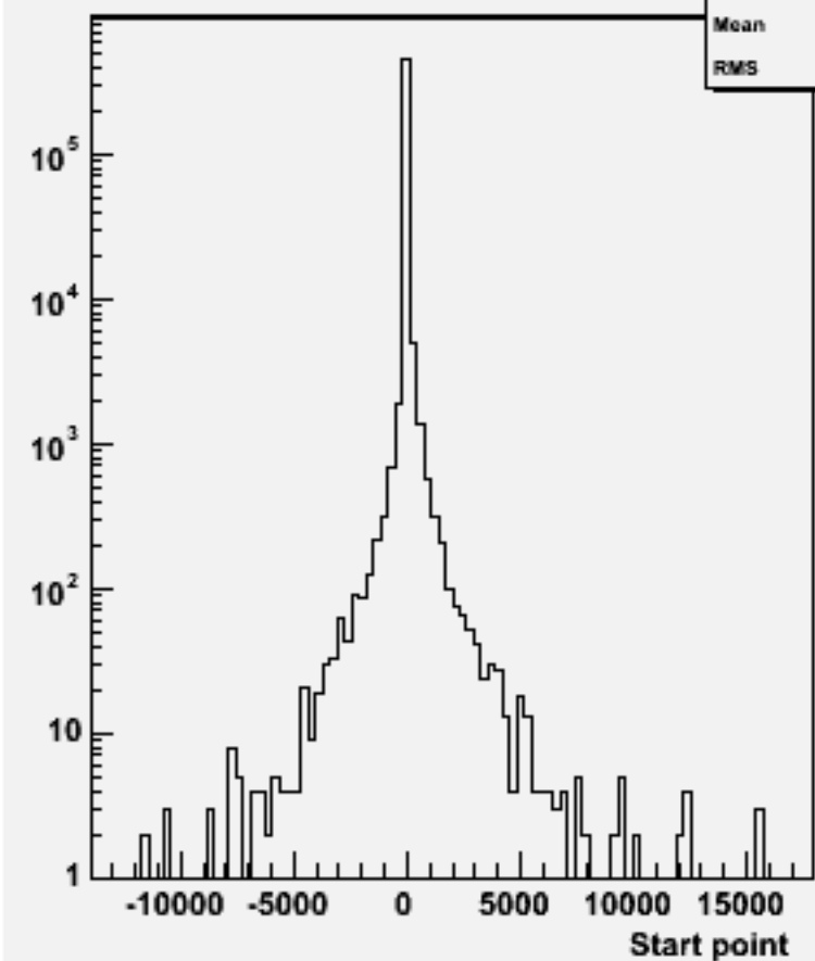
Start point Z : w102503 e1e1e3e3dd_o
