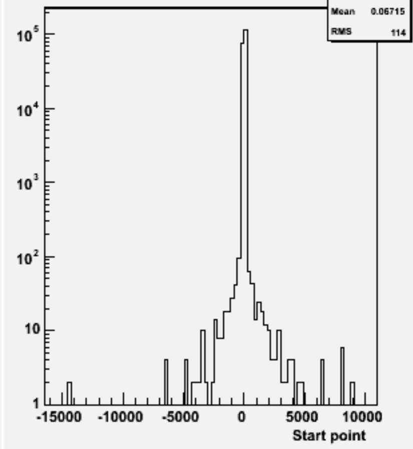
Start point Z : w102502 e1e1e3e3e3e3_o
