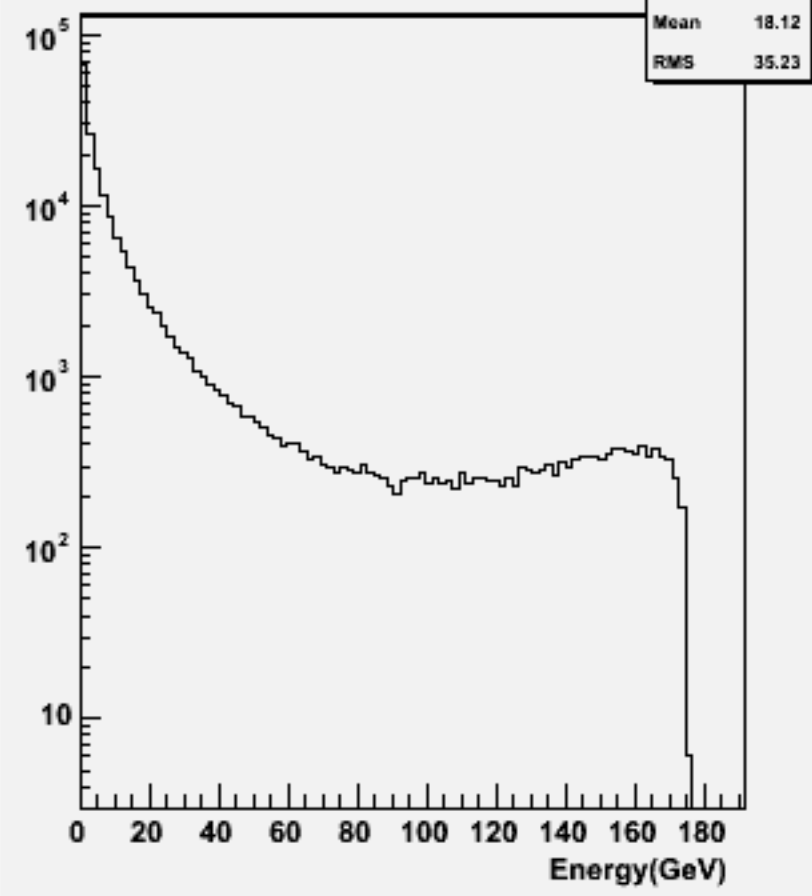
Start point R : w102502 e1e1e3e3e3e3_o
