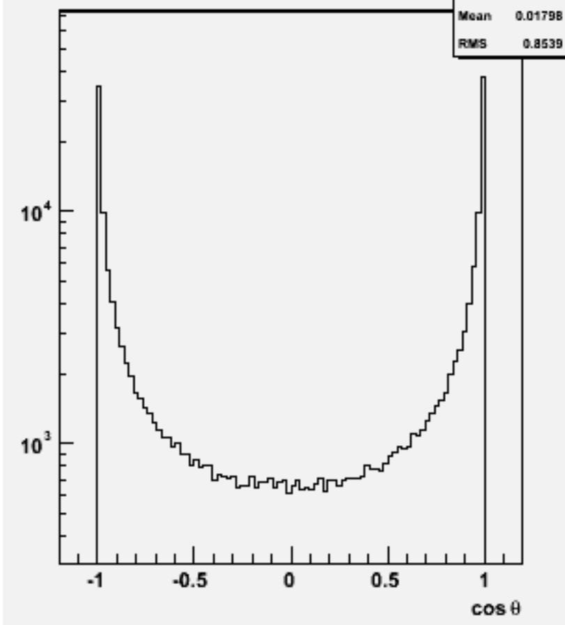
Particle cos \theta : w102502 e1e1e3e3e3e3_o
