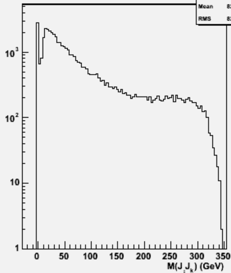
2jets mass(All comb)w102502 e1e1e3e3e3e3_o
