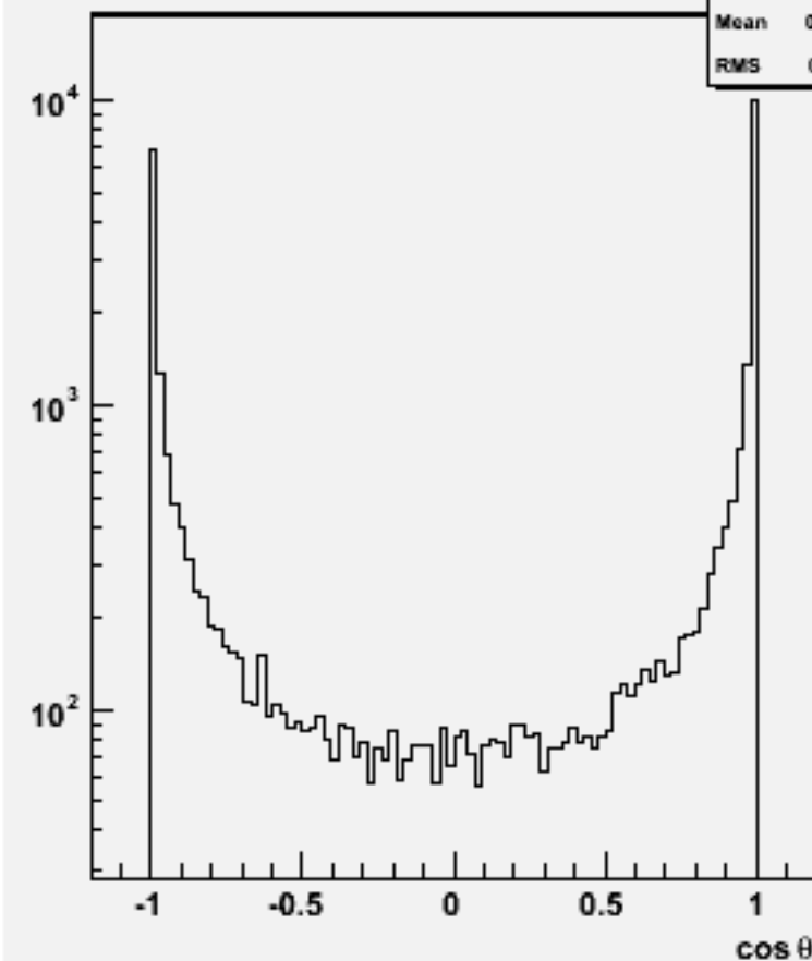
Jet cos \theta (All jets)w102502 e1e1e3e3e3e3_o
