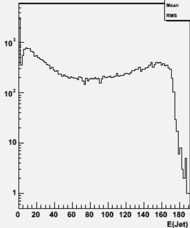
Jet energies(All jets)w102502 e1e1e3e3e3e3_o
