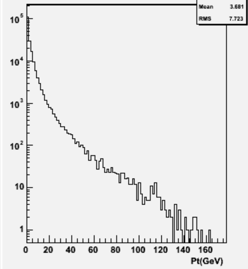
Start point Z : w102501 e1e1e3e3e3e3_o
