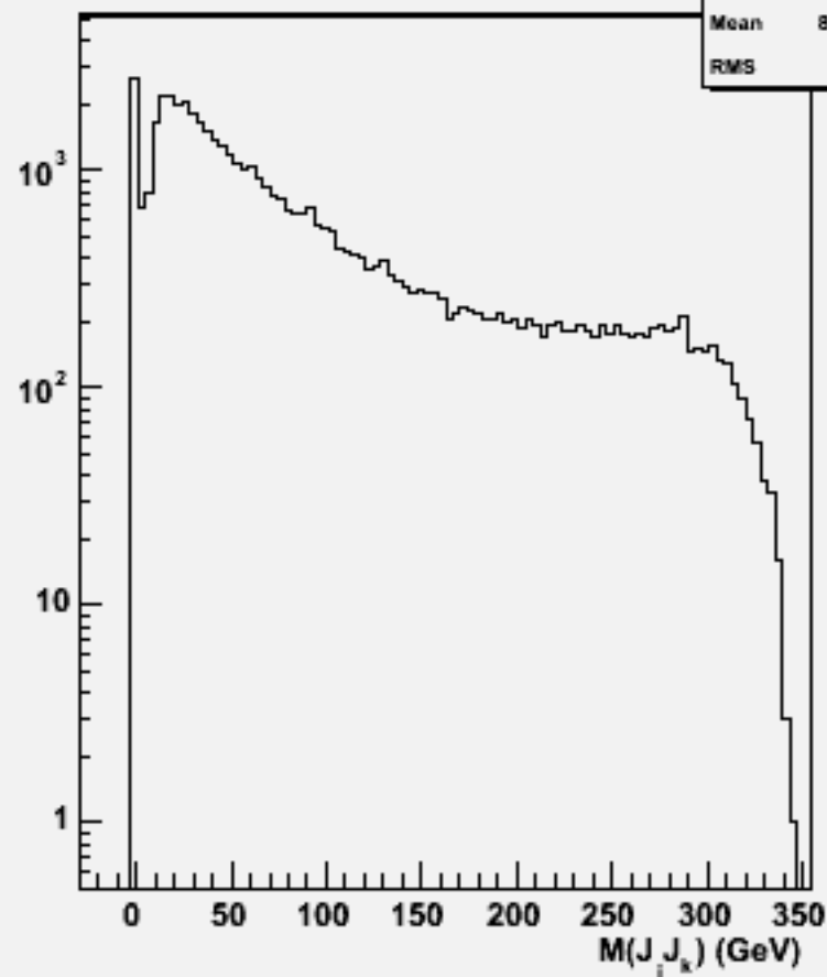
2jets mass(All comb)w102501 e1e1e3e3e3e3_o
