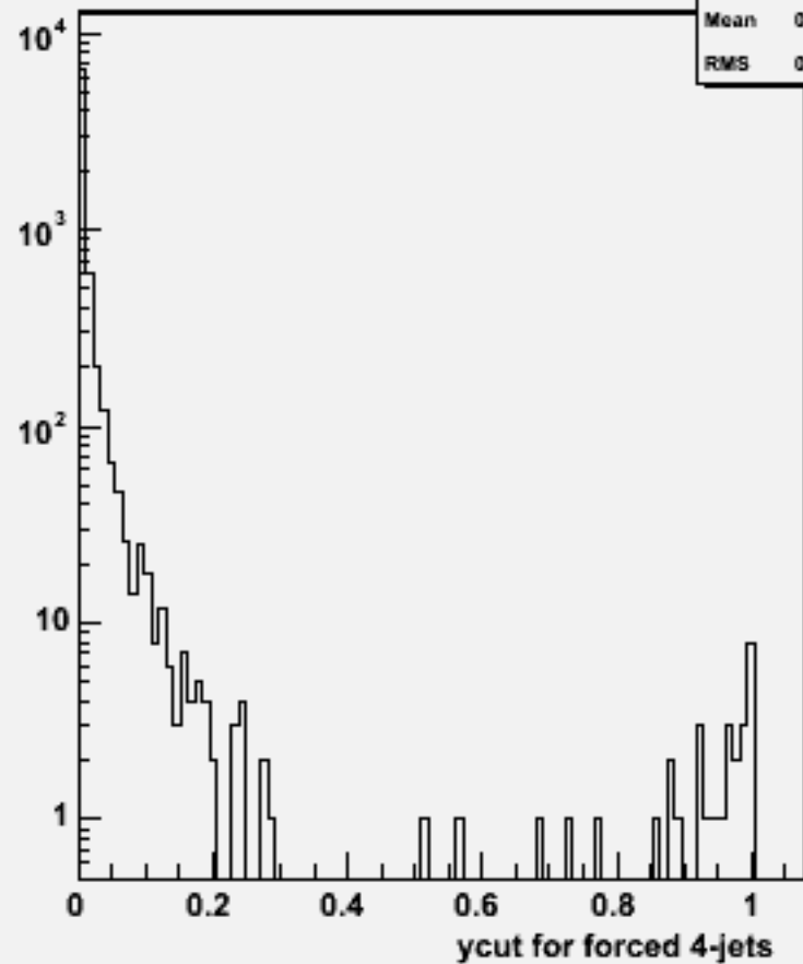
Ycut for 4-jets :w102501 e1e1e3e3e3e3_o
