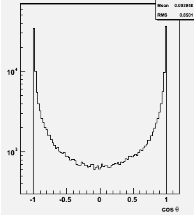
Particle cos \theta : w102501 e1e1e3e3e3e3_o
