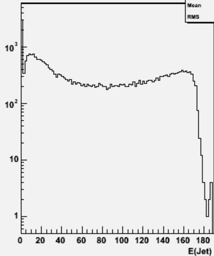
Jet energies(All jets)w102501 e1e1e3e3e3e3_o
