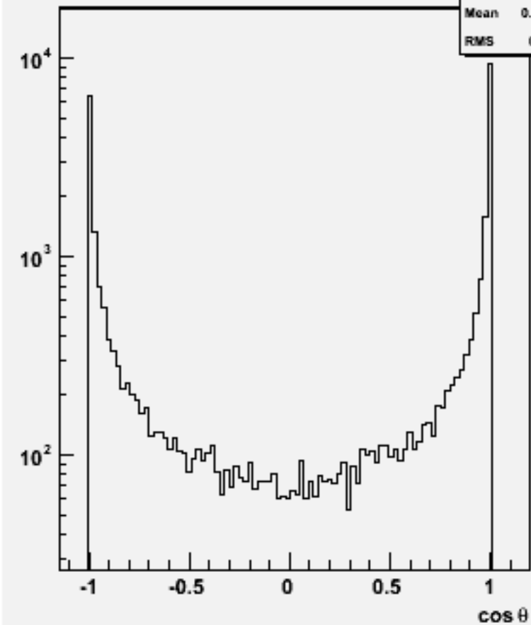
Jet cos \theta (All jets)w102501 e1e1e3e3e3e3_o
