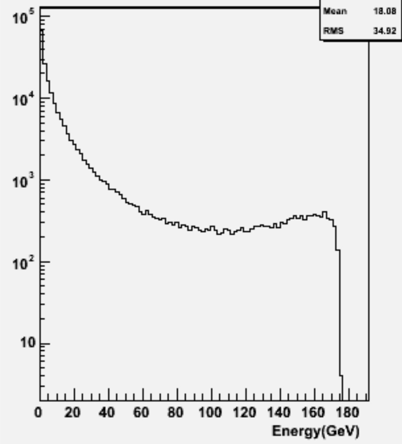
Start point R : w102501 e1e1e3e3e3e3_o
