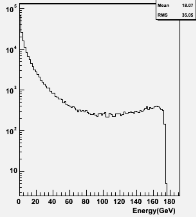
Start point R : w102499 e1e1e3e3e3e3_o
