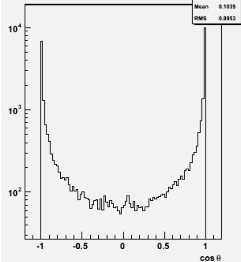
Jet cos \theta (All jets)w102499 e1e1e3e3e3e3_o
