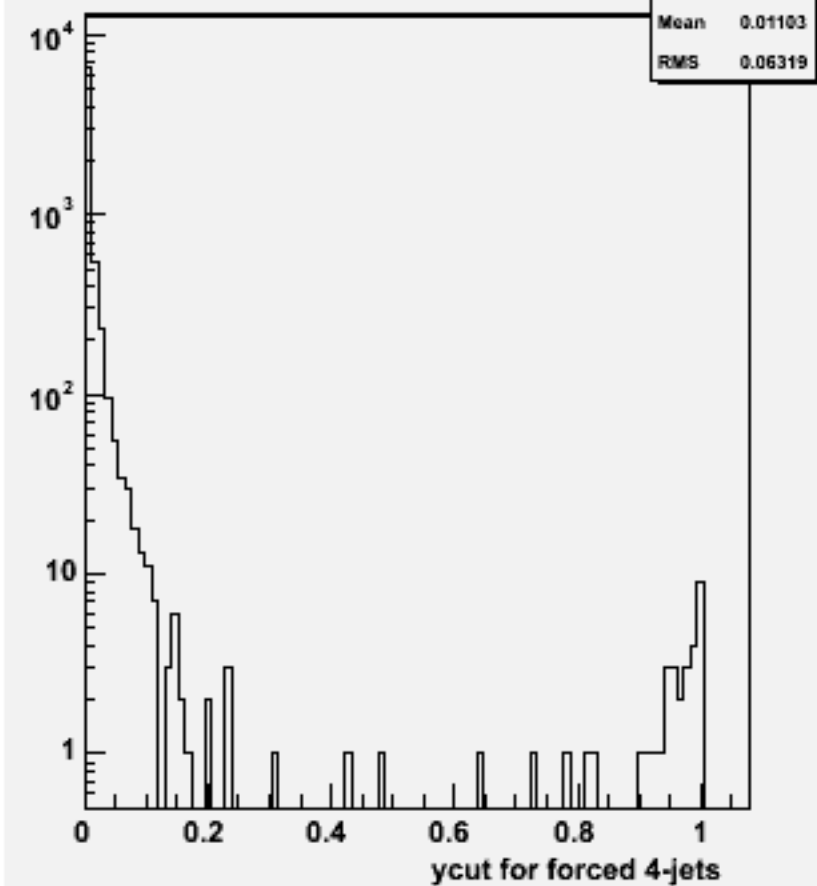
Ycut for 4-jets :w102499 e1e1e3e3e3e3_o
