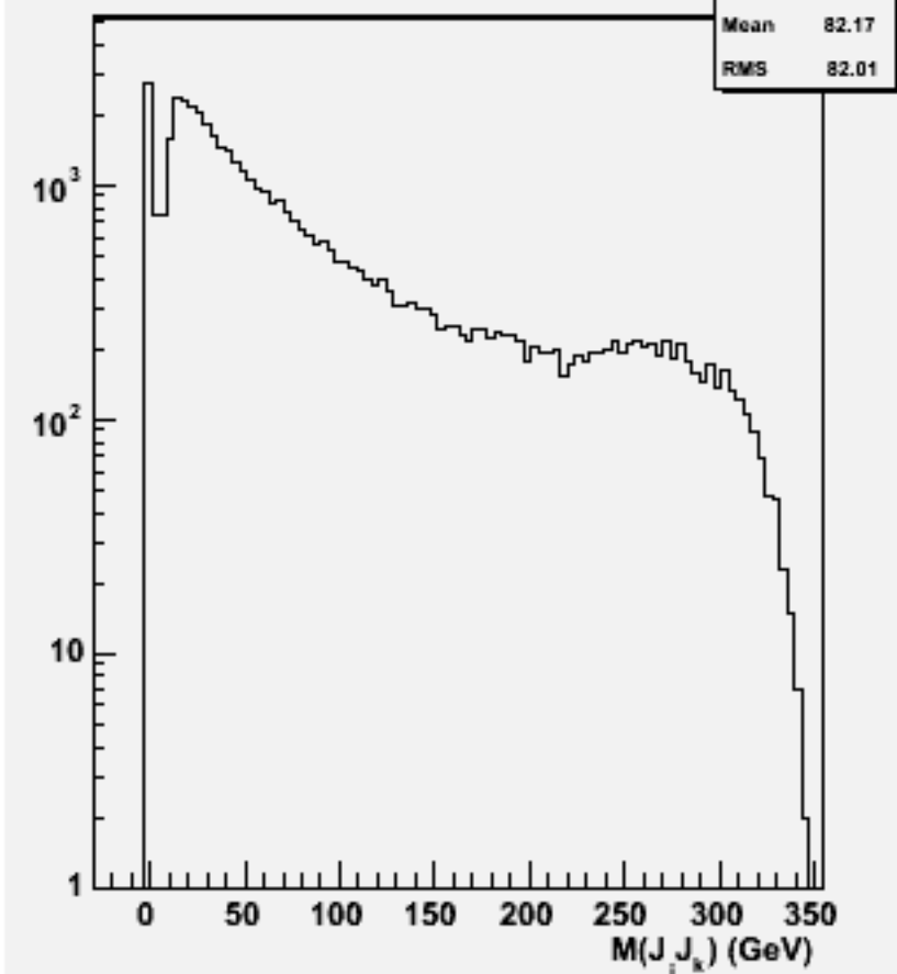
2jets mass(All comb)w102499 e1e1e3e3e3e3_o
