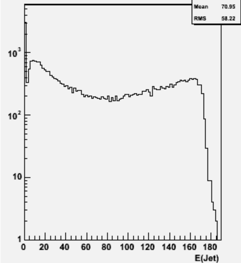
Jet energies(All jets)w102499 e1e1e3e3e3e3_o
