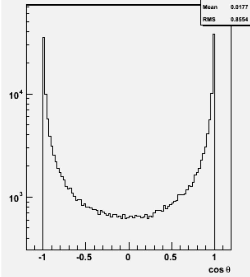
Particle cos \theta : w102499 e1e1e3e3e3e3_o
