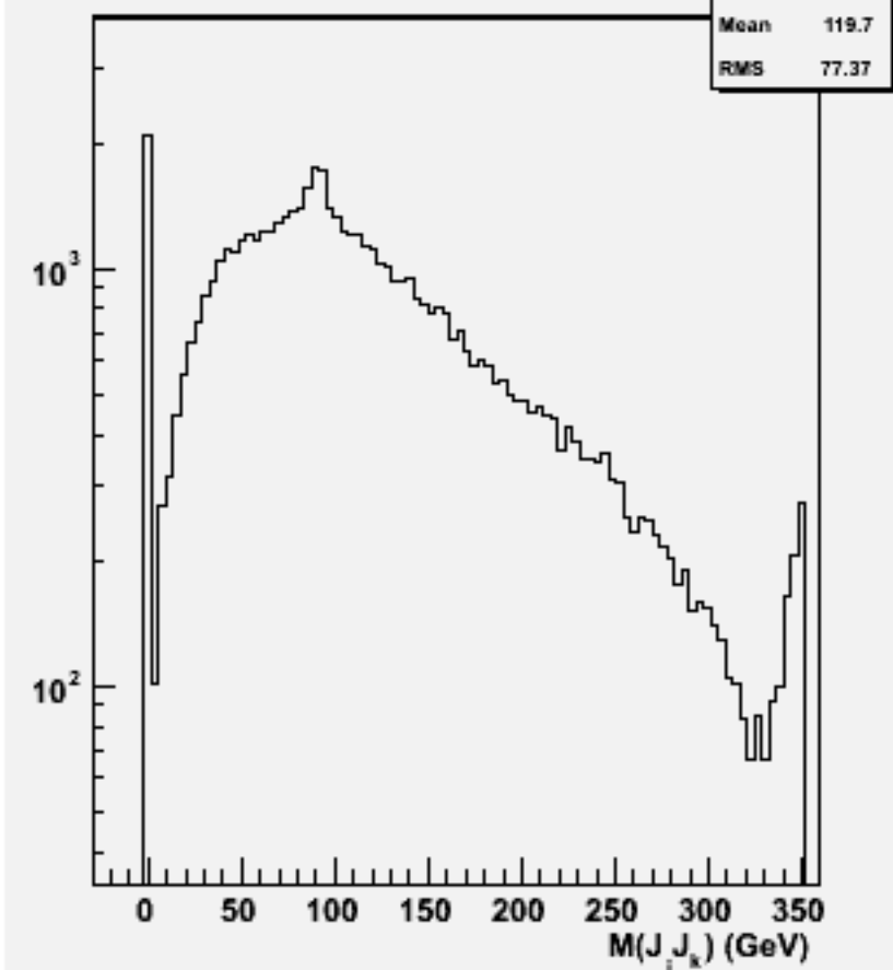
2jets mass(All comb)w102498 e1e1e2e2bb_o
