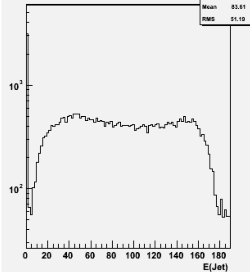
Jet energies(All jets)w102498 e1e1e2e2bb_o
