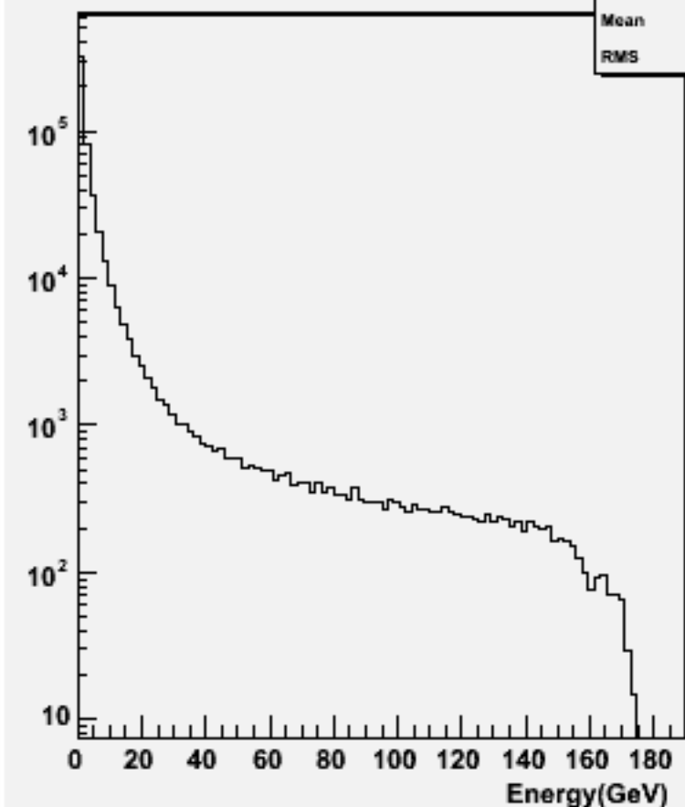
Particle Energy : w102498 e1e1e2e2bb_o
