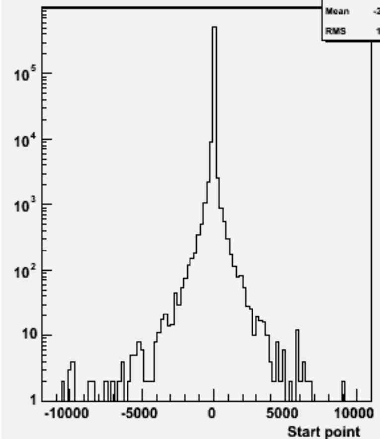
Start point Z : w102498 e1e1e2e2bb_o
