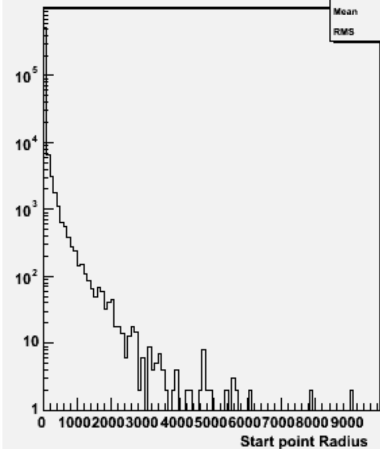
Start point R : w102498 e1e1e2e2bb_o
