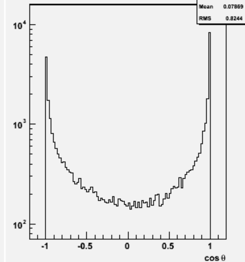
Jet cos \theta (All jets)w102498 e1e1e2e2bb_o
