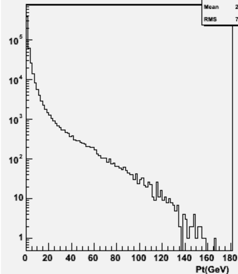
Particle Pt : w102498 e1e1e2e2bb_o
