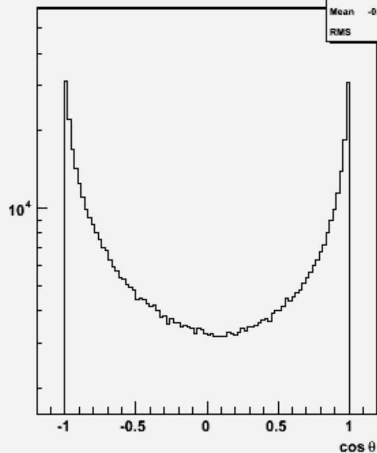
Particle cos \theta : w102498 e1e1e2e2bb_o
