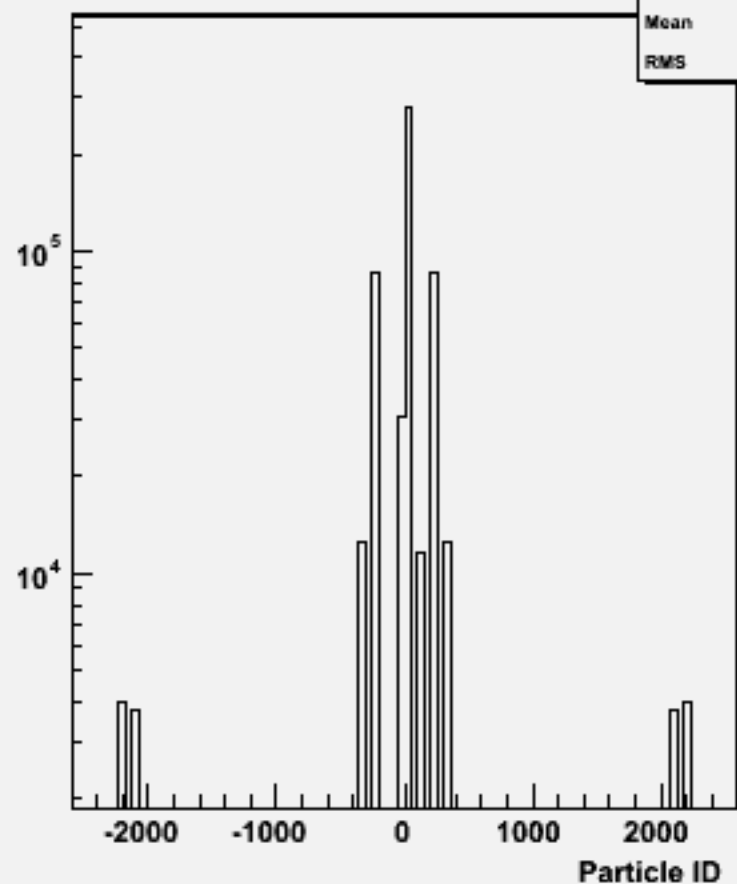
Particle ID : w102498 e1e1e2e2bb_o
