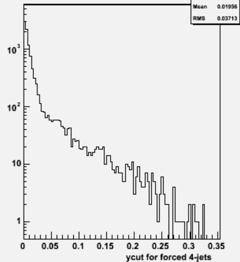
Ycut for 4-jets :w102498 e1e1e2e2bb_o
