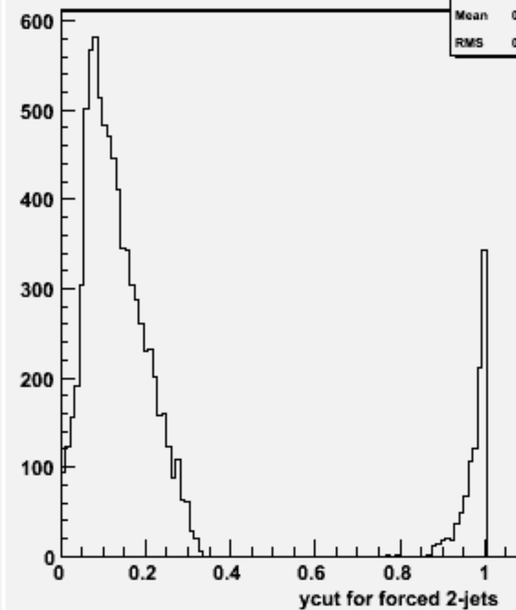
Ycut for 2-jets :w102496 e1e1e2e2bb_o
