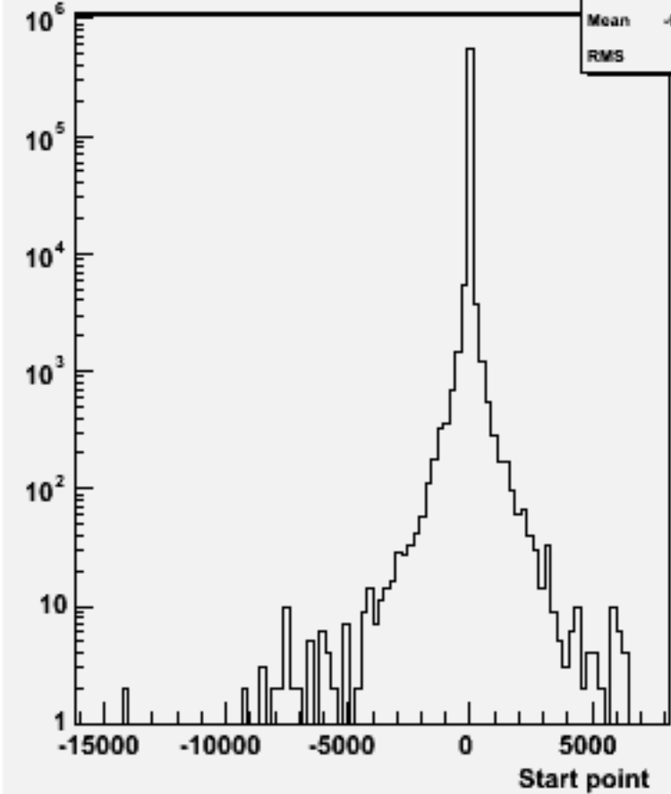
Start point Z : w102496 e1e1e2e2bb_o
