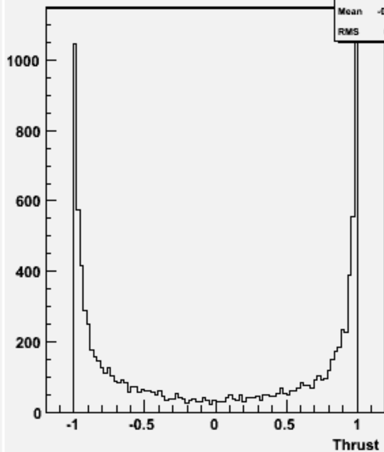
cos \Theta (thrust) w102496 e1e1e2e2bb_o
