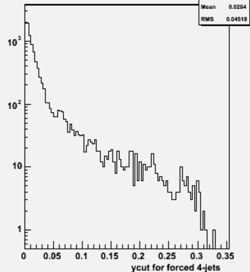
Ycut for 4-jets :w102496 e1e1e2e2bb_o
