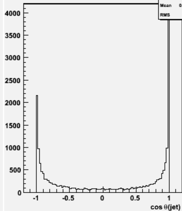
cos \theta for 2-jets :w102496 e1e1e2e2bb_o
