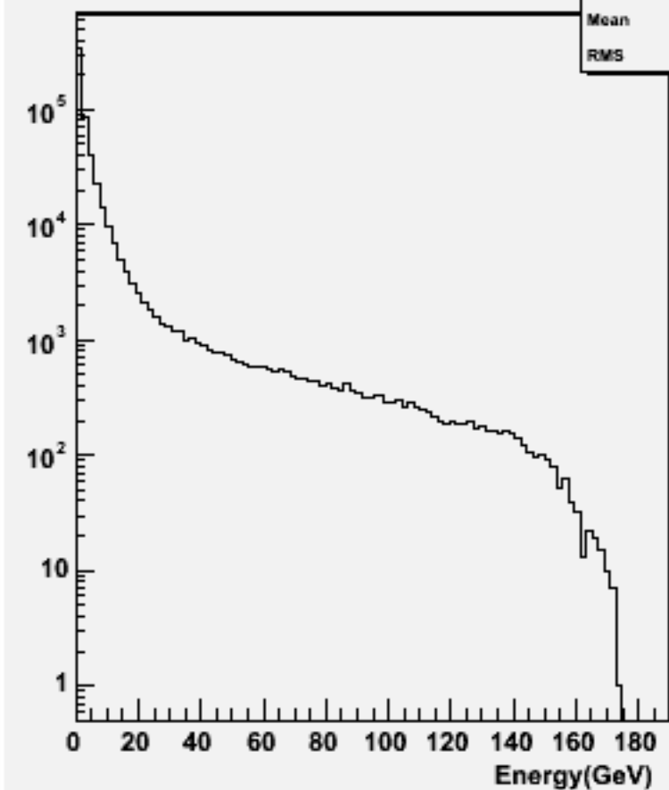
Particle Energy : w102496 e1e1e2e2bb_o
