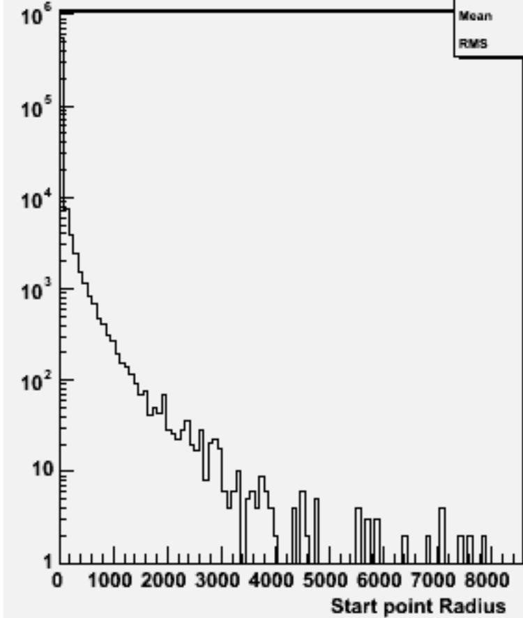
Start point R : w102496 e1e1e2e2bb_o
