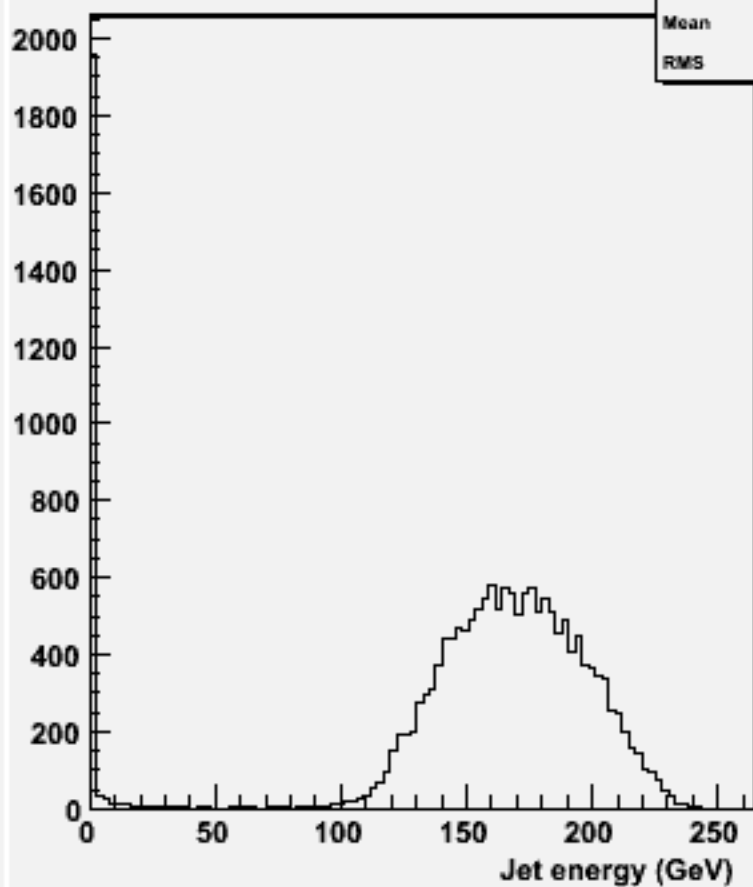
energy for 2-jets :w102496 e1e1e2e2bb_o
