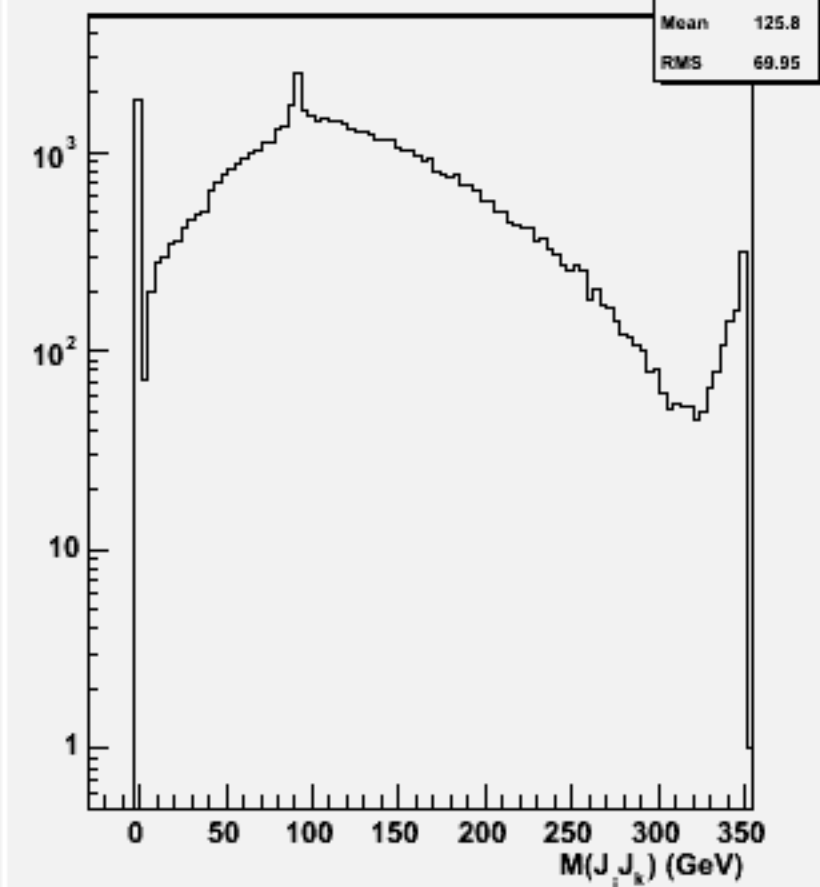
2jets mass(All comb)w102496 e1e1e2e2bb_o
