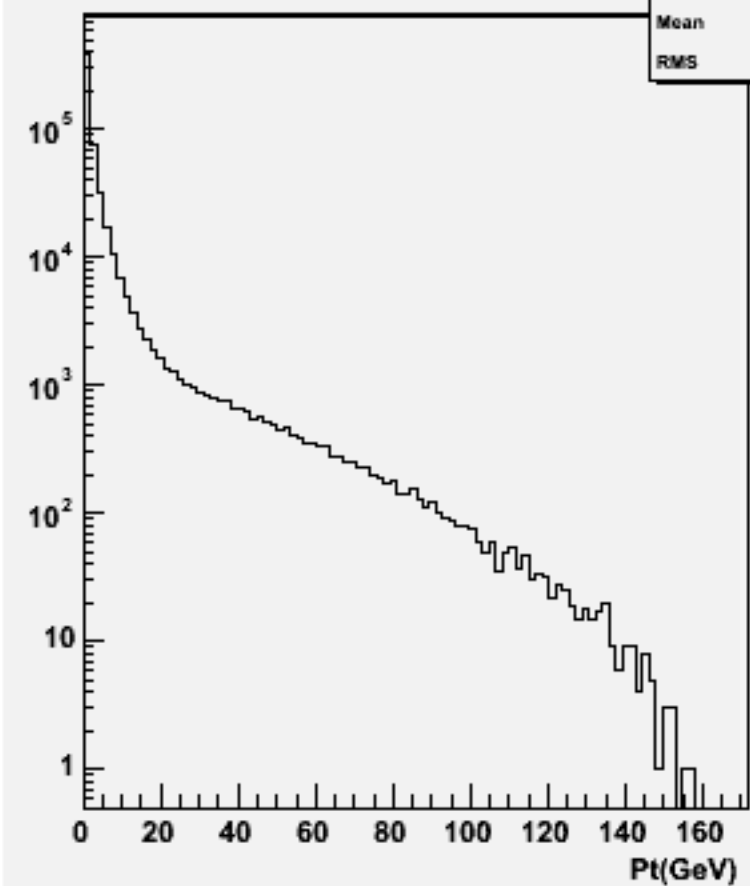
Particle Pt : w102496 e1e1e2e2bb_o
