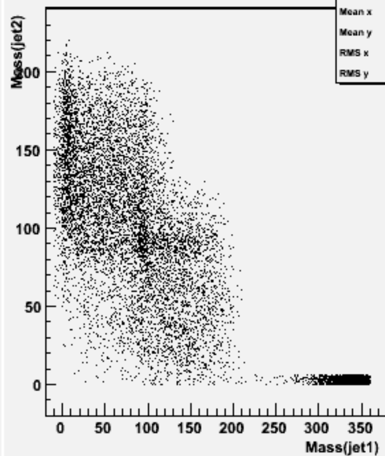
Jet mass for forced 2-jets : w102496 e1e1e2e2bb_o
