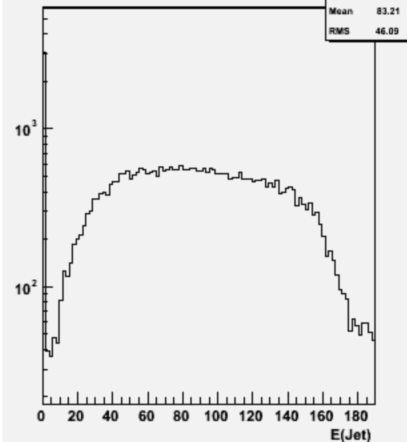
Jet energies(All jets)w102496 e1e1e2e2bb_o
