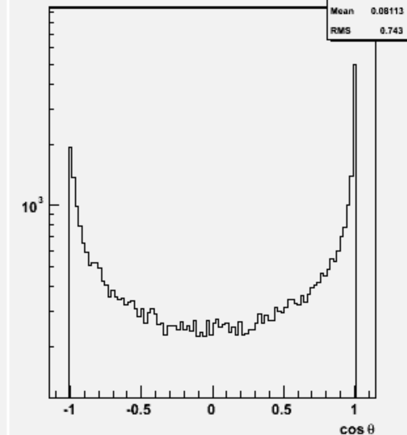
Jet cos \theta (All jets)w102496 e1e1e2e2bb_o
