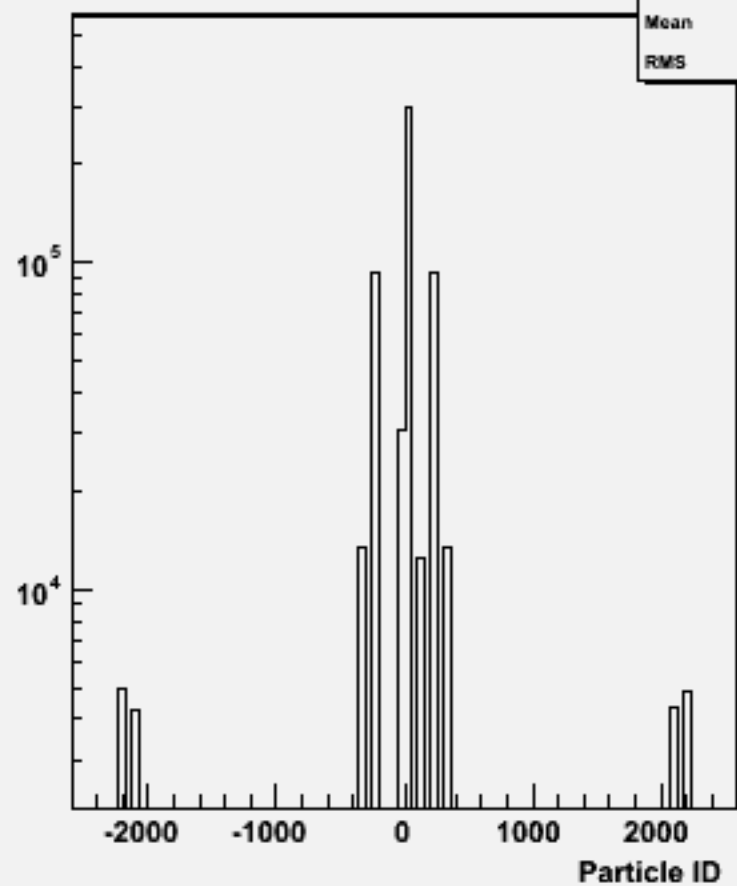
Particle ID : w102496 e1e1e2e2bb_o
