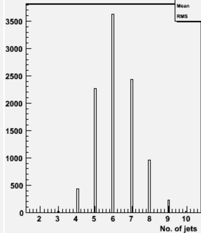
No. jets (ycut=0.001) : w102496 e1e1e2e2bb_o
