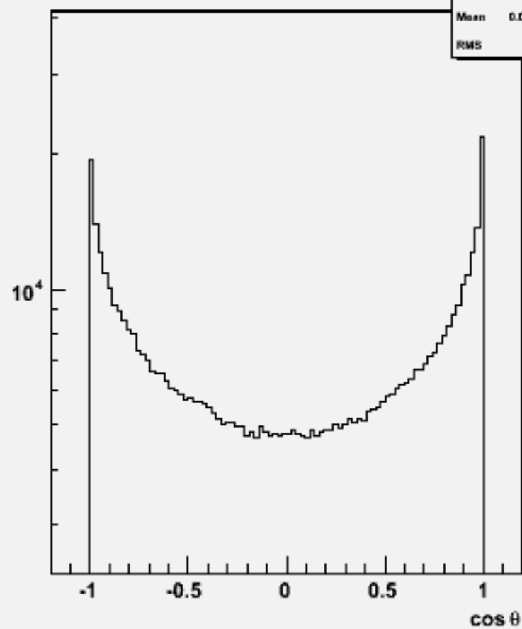
Particle cos \theta : w102496 e1e1e2e2bb_o
