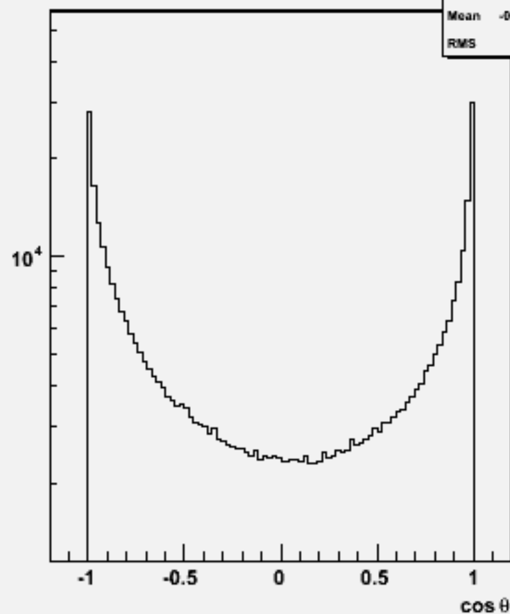
Particle cosθ : w102494 e1e1e2e2ss_o
