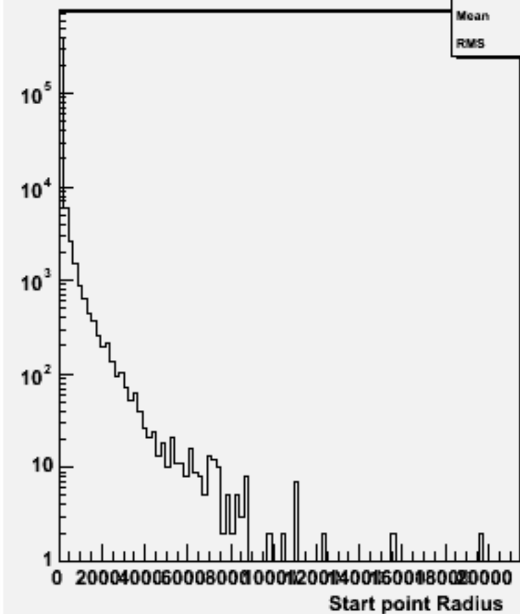
Start point R : w102494 e1e1e2e2ss_o
