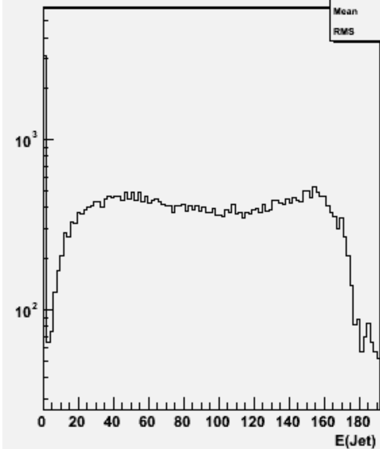
Jet energies(All jets)w102494 e1e1e2e2ss_o
