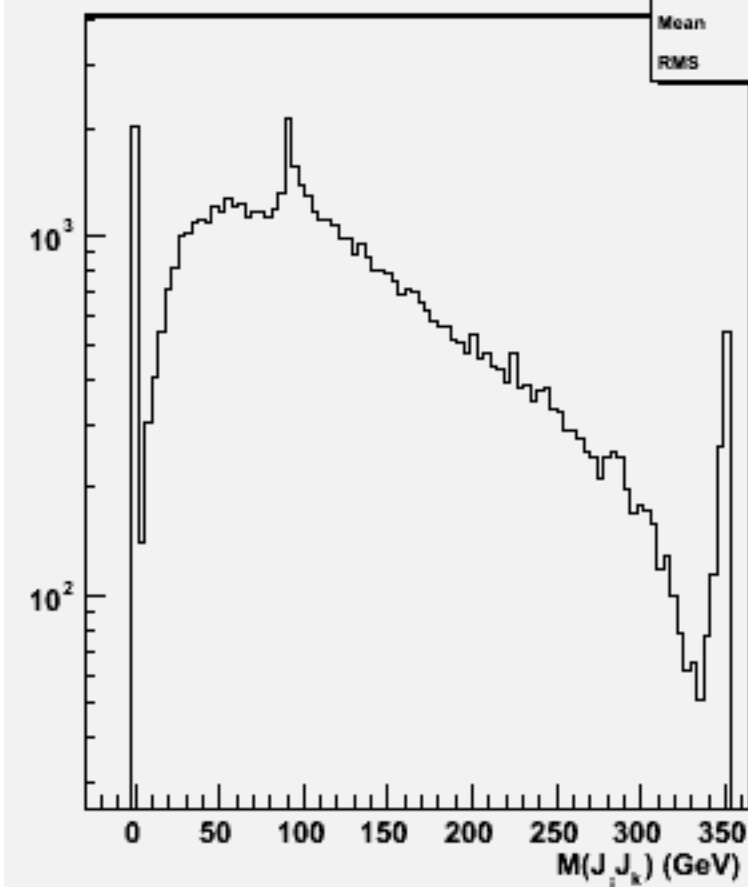
2jets mass(All comb)w102494 e1e1e2e2ss_o
