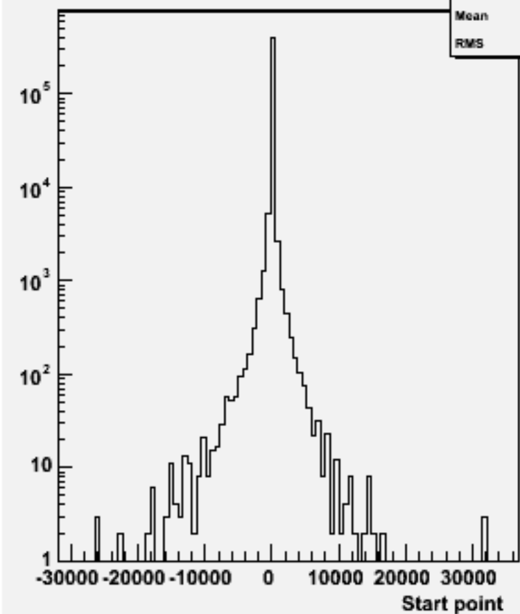
Start point Z : w102494 e1e1e2e2ss_o
