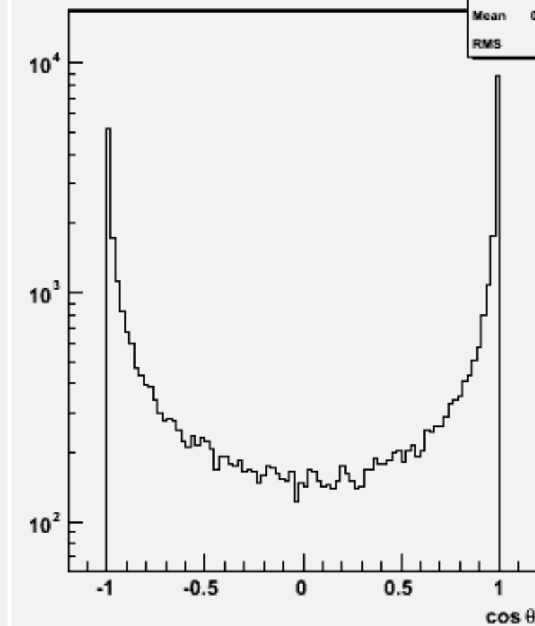
Jet cos θ (All jets)w102494 e1e1e2e2ss_o
