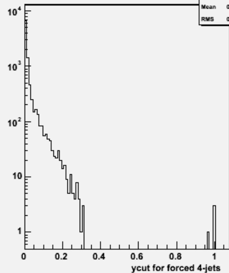
Ycut for 4-jets :w102494 e1e1e2e2ss_o
