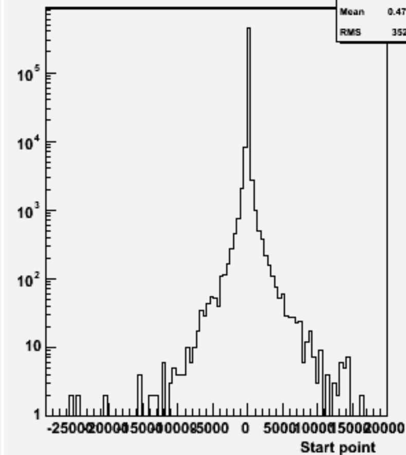
Start point Z : w102492 e1e1e2e2ss_o
