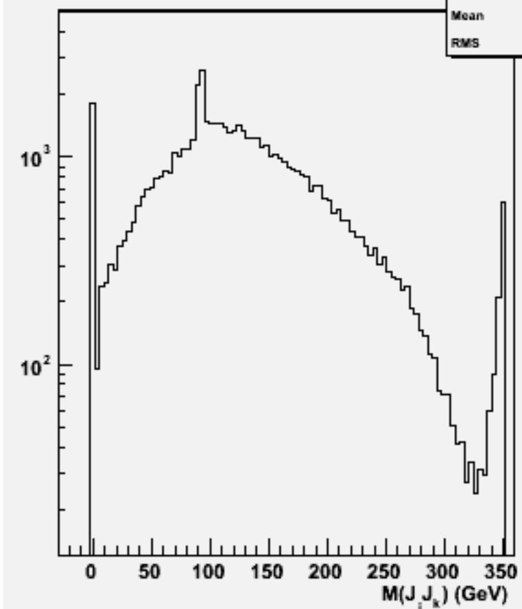
2jets mass(All comb)w102492 e1e1e2e2ss_o
