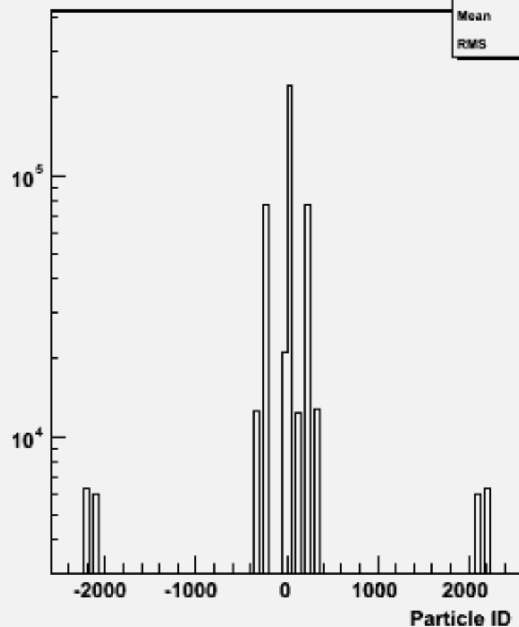
Particle ID : w102492 e1e1e2e2ss_o
