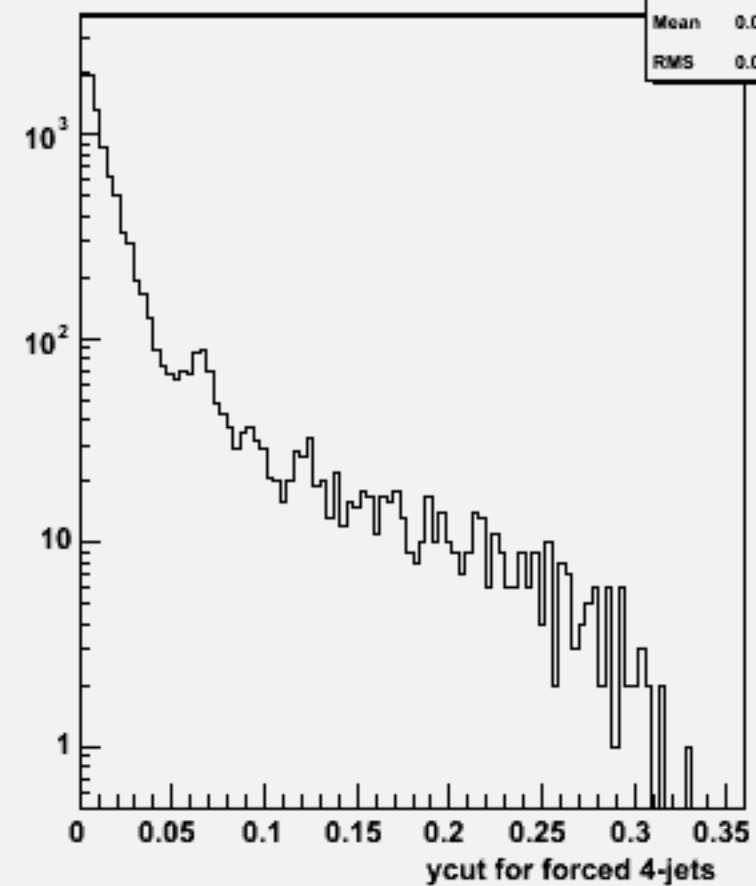
Ycut for 4-jets :w102492 e1e1e2e2ss_o
