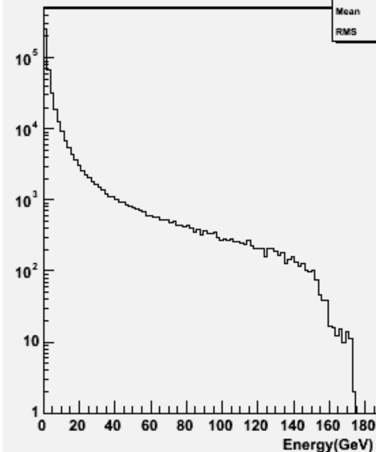
Particle Energy : w102492 e1e1e2e2ss_o
