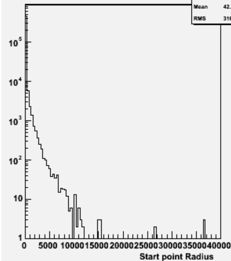
Start point R : w102492 e1e1e2e2ss_o
