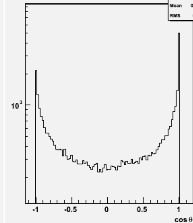
Jet cos \theta (All jets)w102492 e1e1e2e2ss_o
