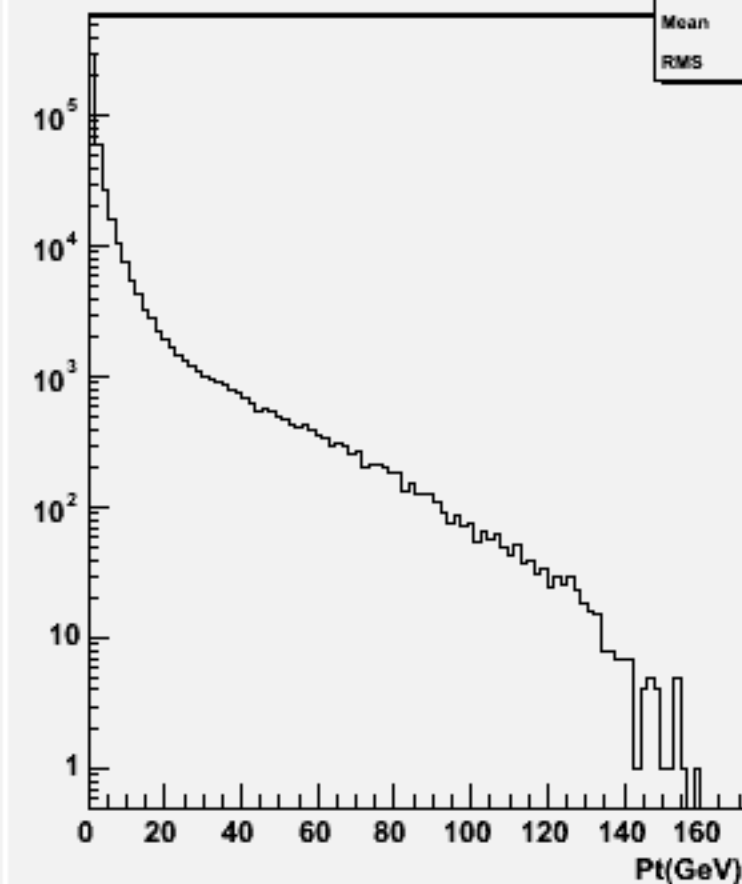
Particle Pt : w102492 e1e1e2e2ss_o
