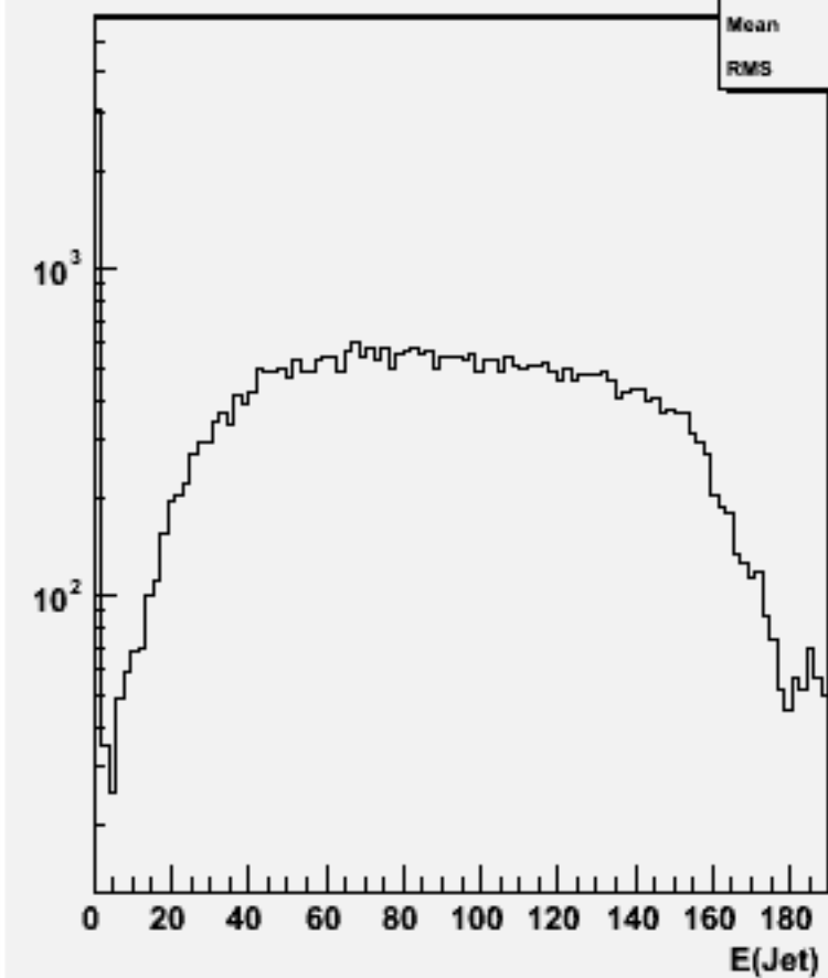
Jet energies(All jets)w102492 e1e1e2e2ss_o
