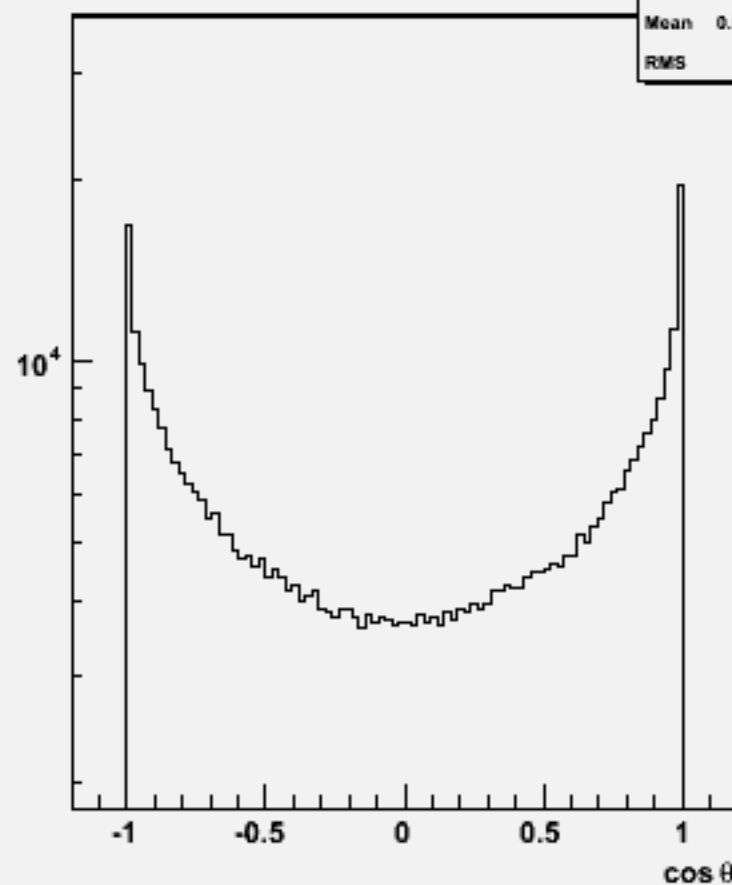
Particle cosθ : w102492 e1e1e2e2ss_o
