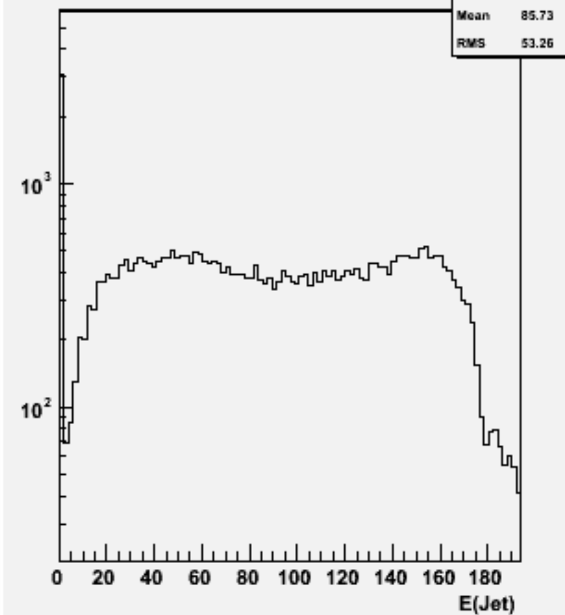
Jet energies(All jets)w102491 e1e1e2e2ss_o
