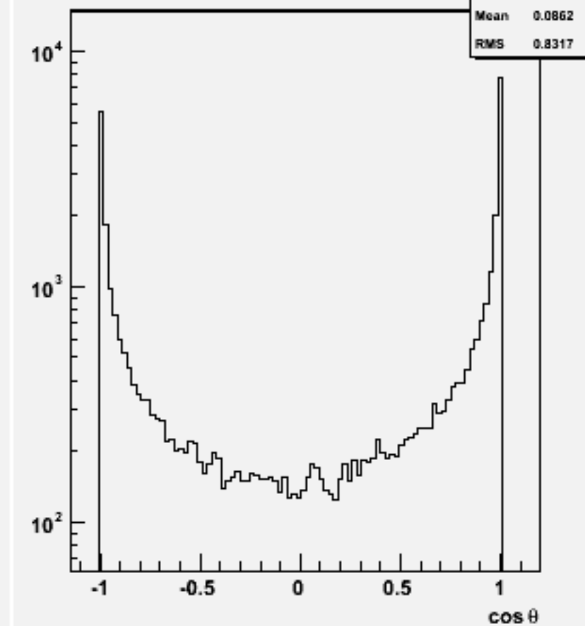
Jet cos \theta (All jets)w102491 e1e1e2e2ss_o
