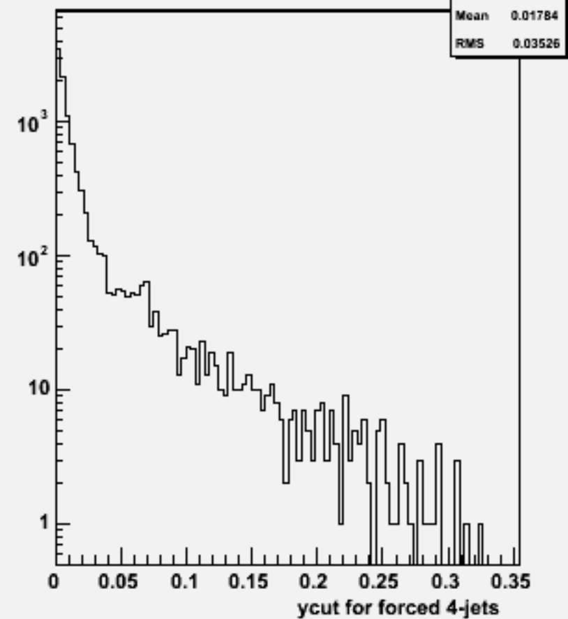
Ycut for 4-jets :w102491 e1e1e2e2ss_o
