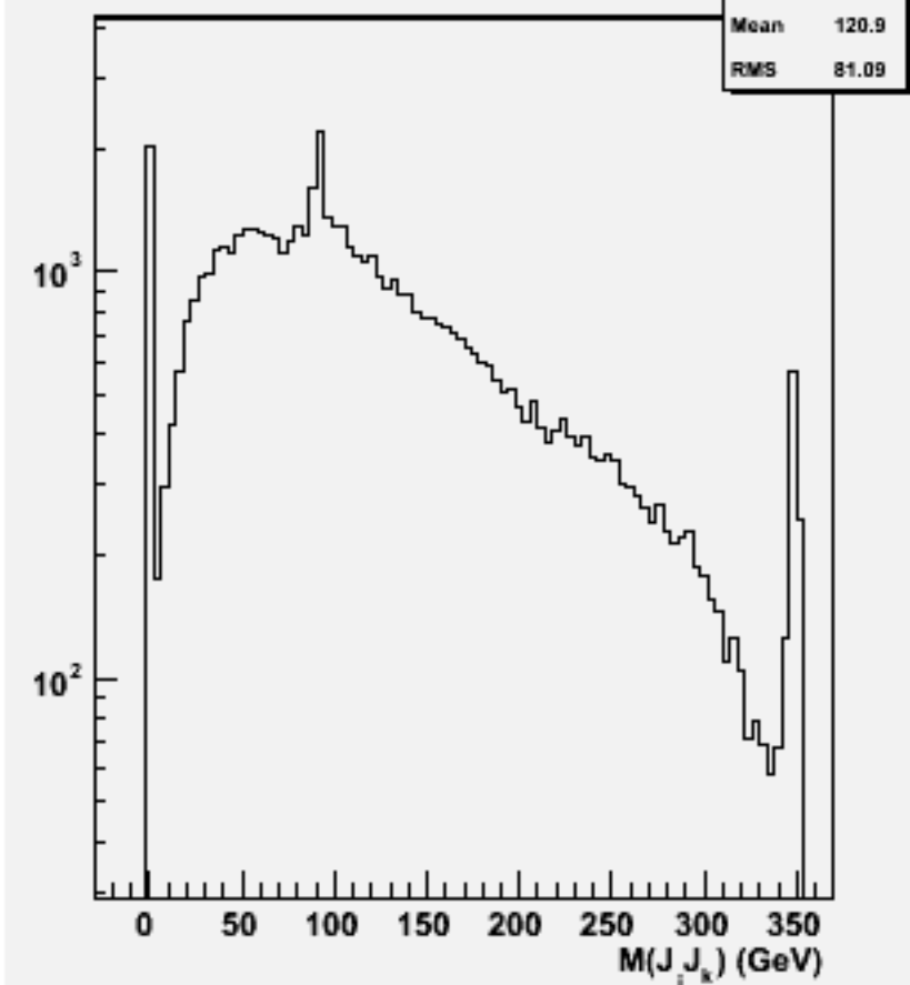
2jets mass(All comb)w102491 e1e1e2e2ss_o
