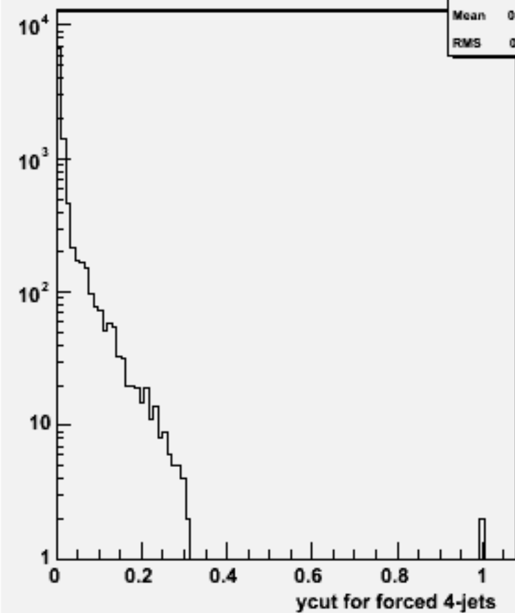
Ycut for 4-jets :w102490 e1e1e2e2dd_o
