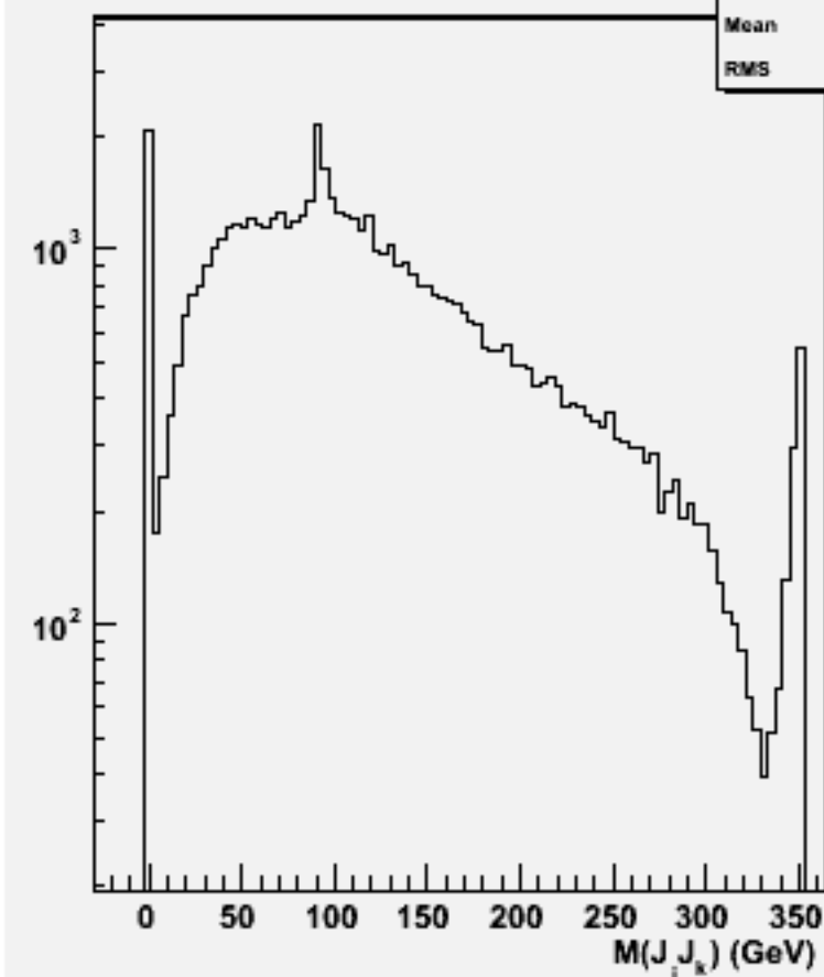
2jets mass(All comb)w102490 e1e1e2e2dd_o
