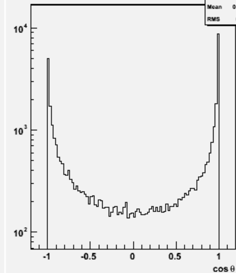
Jet cos \theta (All jets)w102490 e1e1e2e2dd_o
