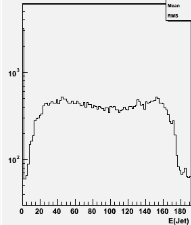
Jet energies(All jets)w102490 e1e1e2e2dd_o
