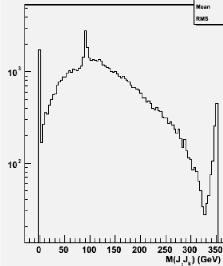
2jets mass(All comb)w102489 e1e1e2e2dd_o
