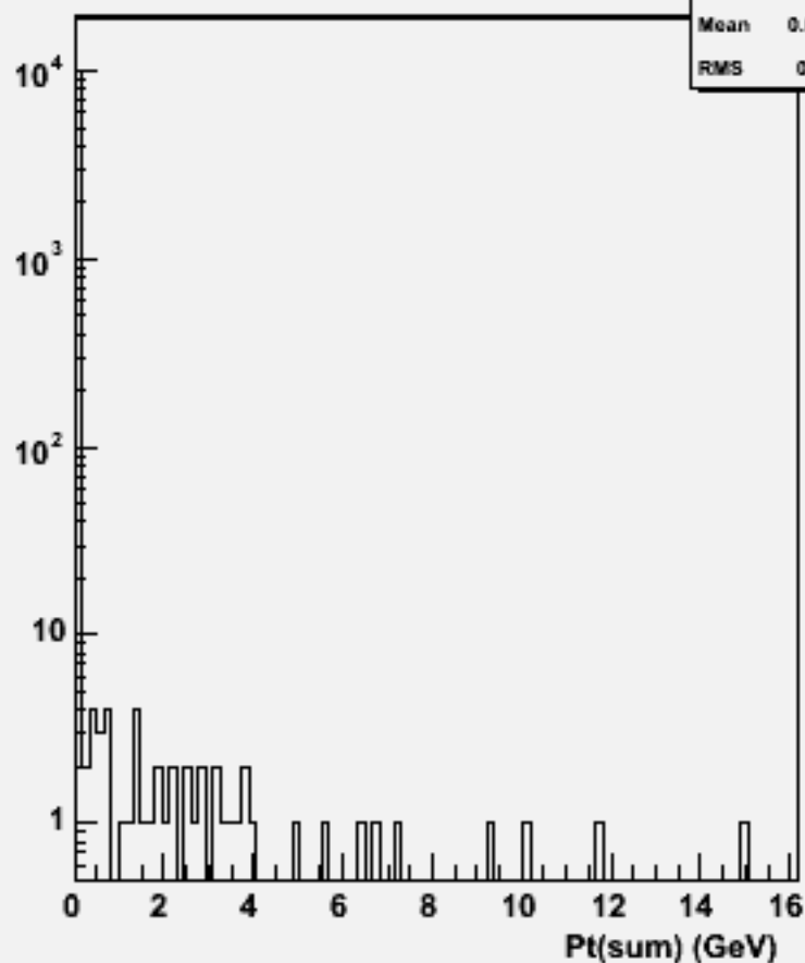
Pt Sum: w102489 e1e1e2e2dd_o
