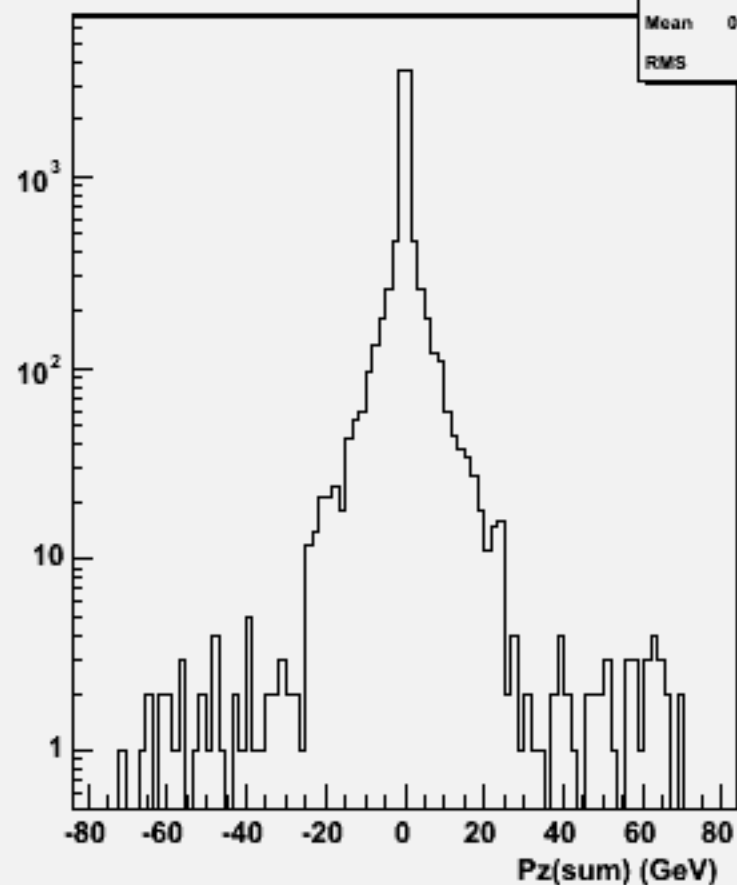
Pz Sum: w102489 e1e1e2e2dd_o
