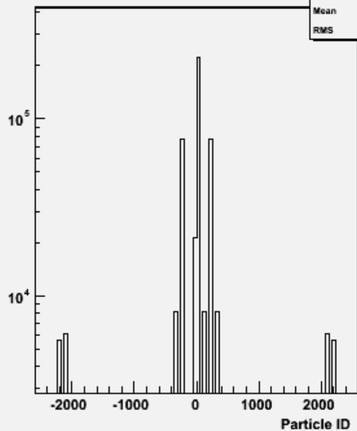
Particle ID : w102489 e1e1e2e2dd_o
