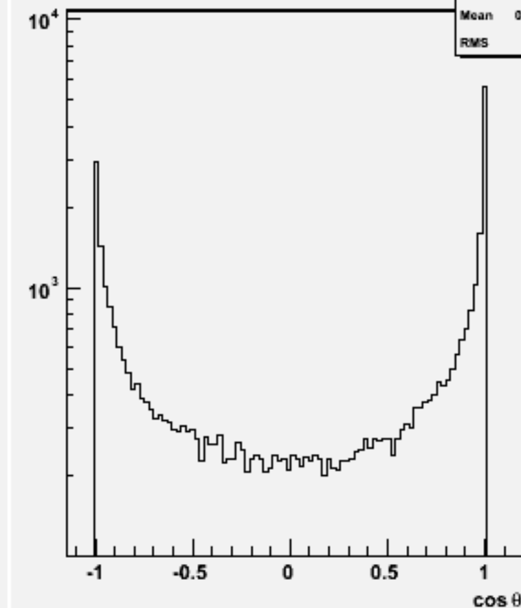
Jet cos \theta (All jets)w102489 e1e1e2e2dd_o
