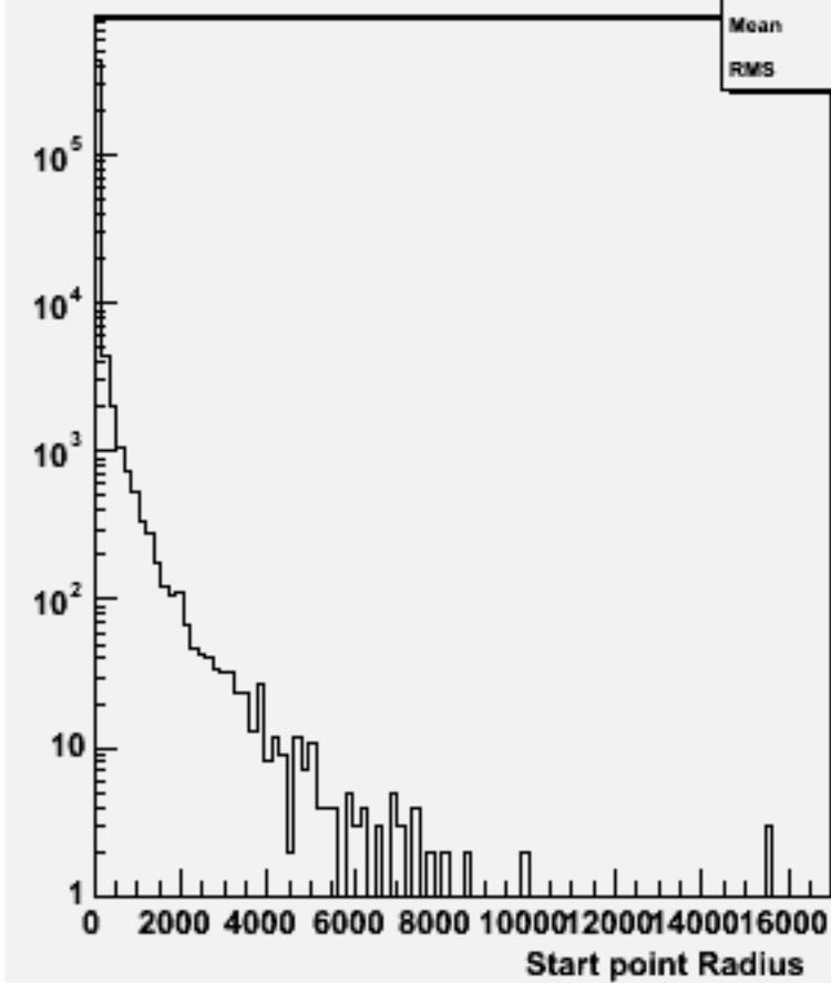
Start point R : w102489 e1e1e2e2dd_o
