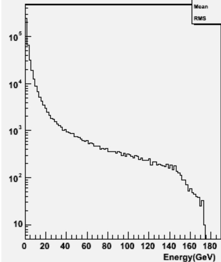
Particle Energy : w102489 e1e1e2e2dd_o
