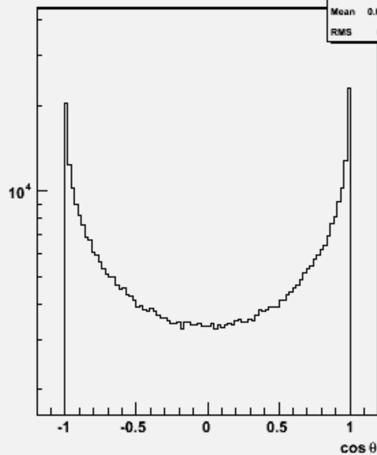
Particle \cos\theta : w102489 e1e1e2e2dd_o
