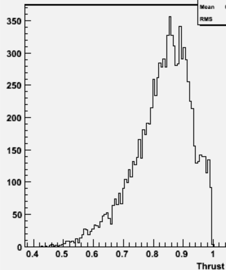
Thrust w102489 e1e1e2e2dd_o
