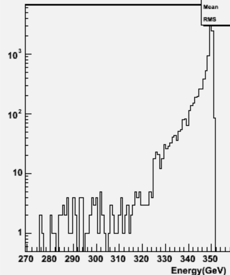
Thrust w102489 e1e1e2e2dd_o
