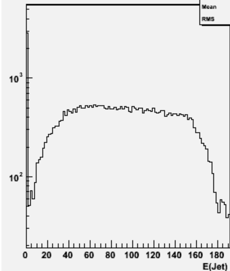
Jet energies(All jets)w102489 e1e1e2e2dd_o
