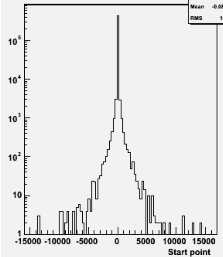
Start point Z : w102489 e1e1e2e2dd_o
