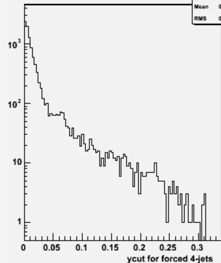
Ycut for 4-jets :w102489 e1e1e2e2dd_o
