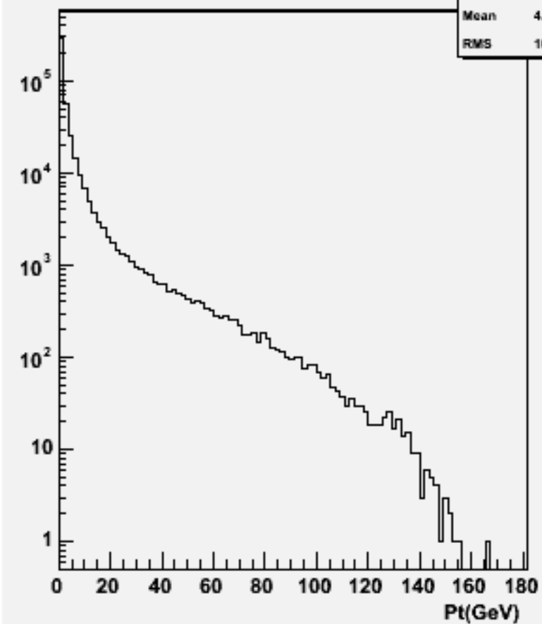
Particle Pt : w102489 e1e1e2e2dd_o
