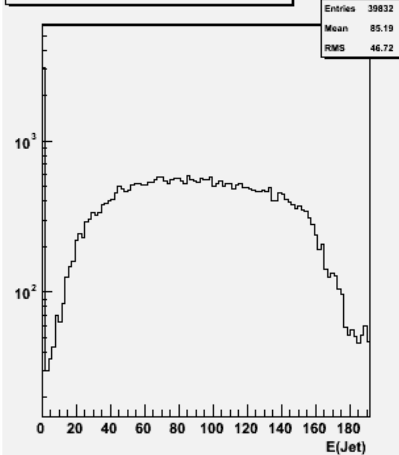
Jet energies(All jets)w102488 e1e1e2e2dd_o
