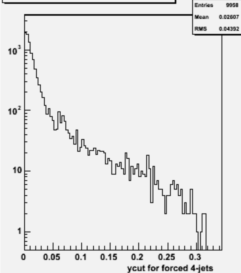
Ycut for 4-jets :w102488 e1e1e2e2dd_o
