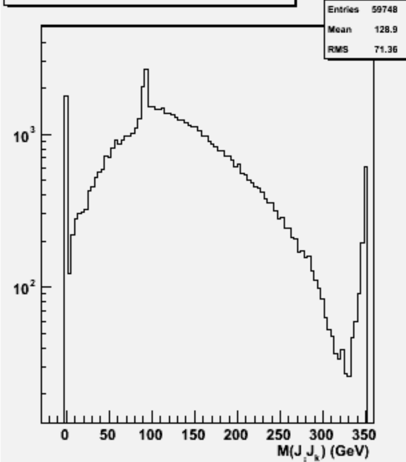
2jets mass(All comb)w102488 e1e1e2e2dd_o
