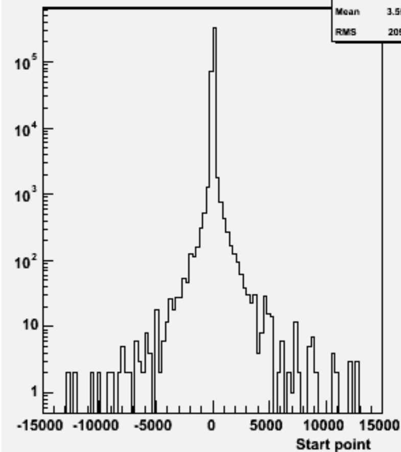
Start point Z : w102487 e1e1e2e2dd_o
