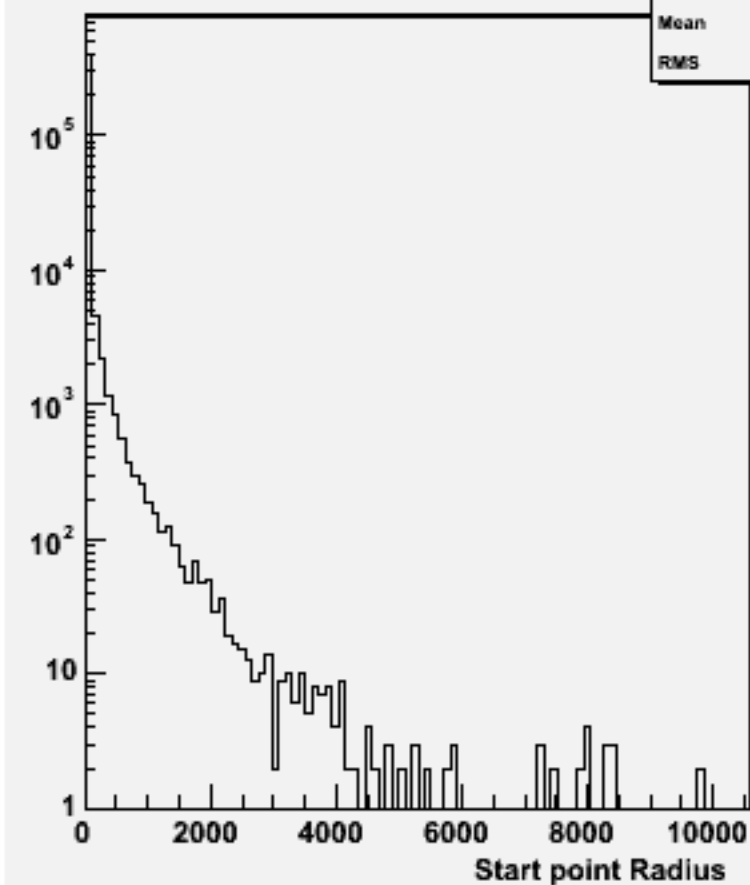
Start point R : w102487 e1e1e2e2dd_o
