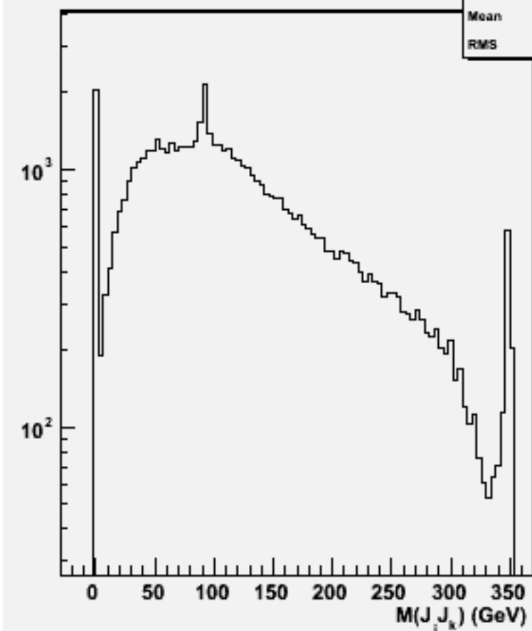
2jets mass(All comb)w102487 e1e1e2e2dd_o
