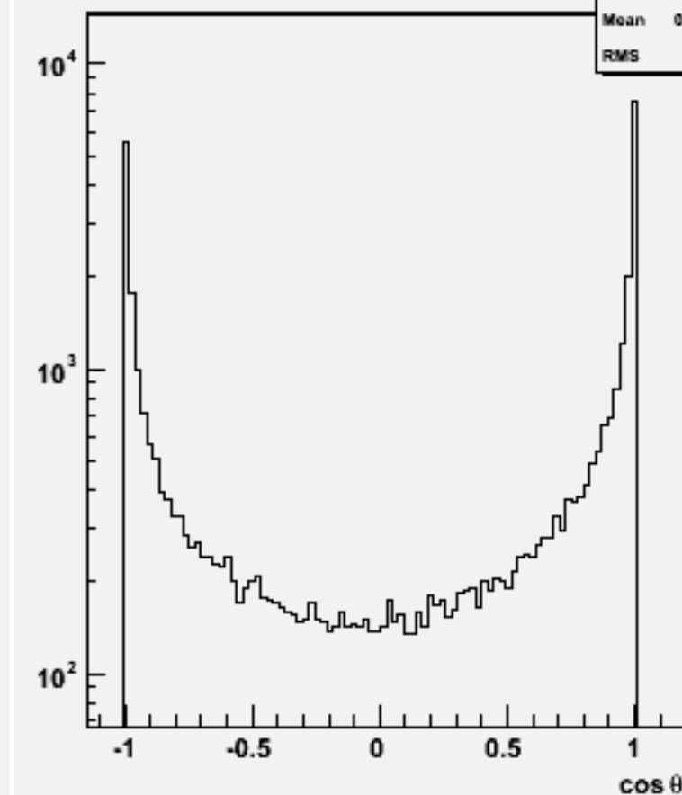
Jet cos \theta (All jets)w102487 e1e1e2e2dd_o
