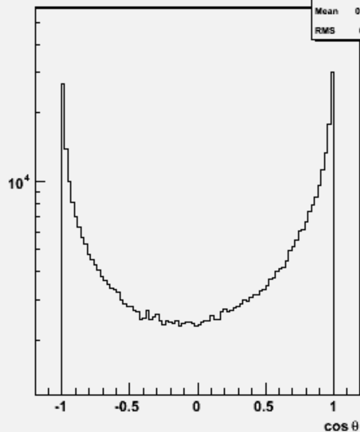
Particle cosθ : w102487 e1e1e2e2dd_o
