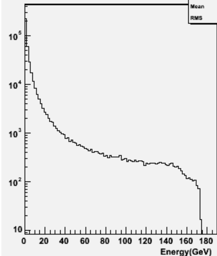
Particle Energy : w102487 e1e1e2e2dd_o
