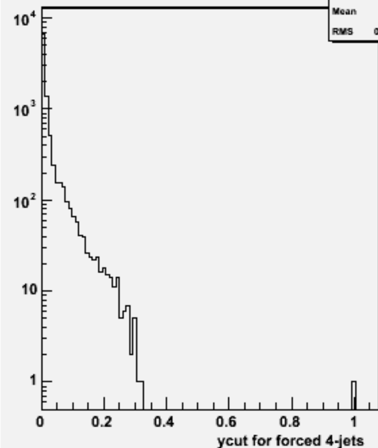
Ycut for 4-jets :w102487 e1e1e2e2dd_o
