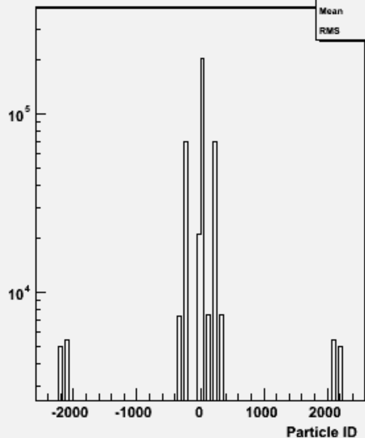
Particle ID : w102487 e1e1e2e2dd_o
