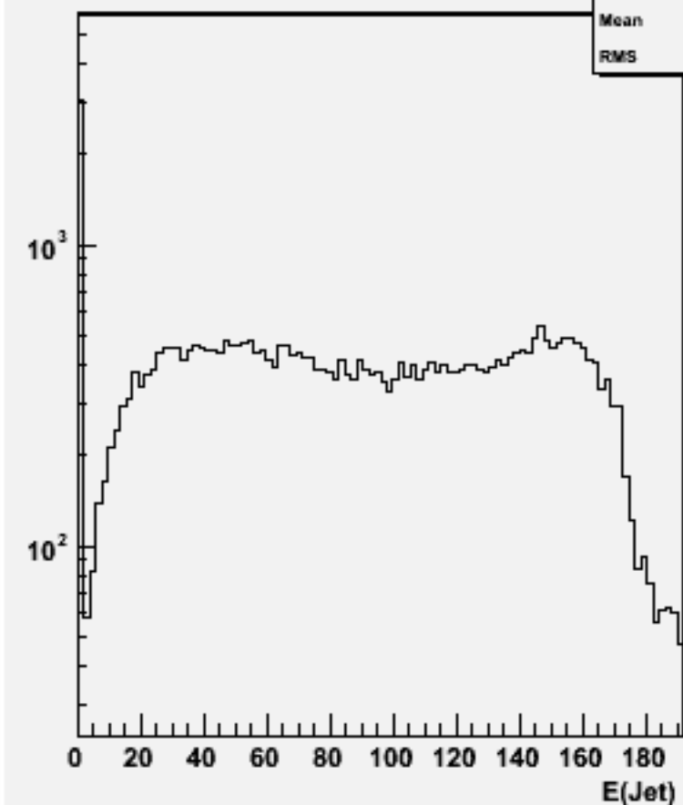
Jet energies(All jets)w102487 e1e1e2e2dd_o
