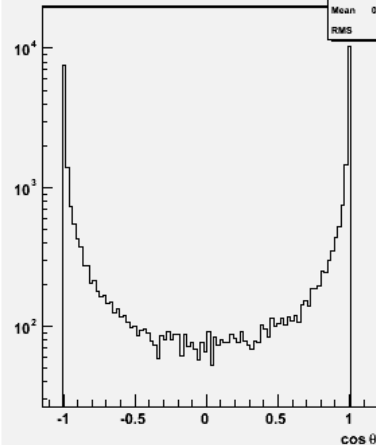
Jet cos \theta (All jets)w102486 e1e1e2e2e3e3_o
