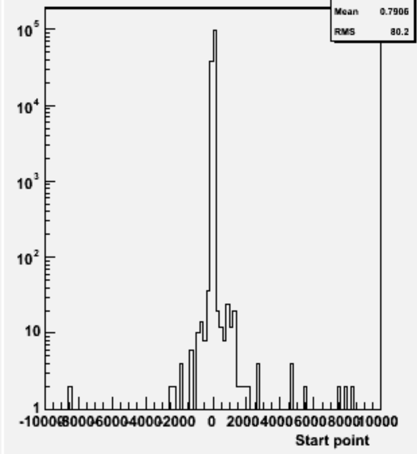
Start point Z : w102486 e1e1e2e2e3e3_o
