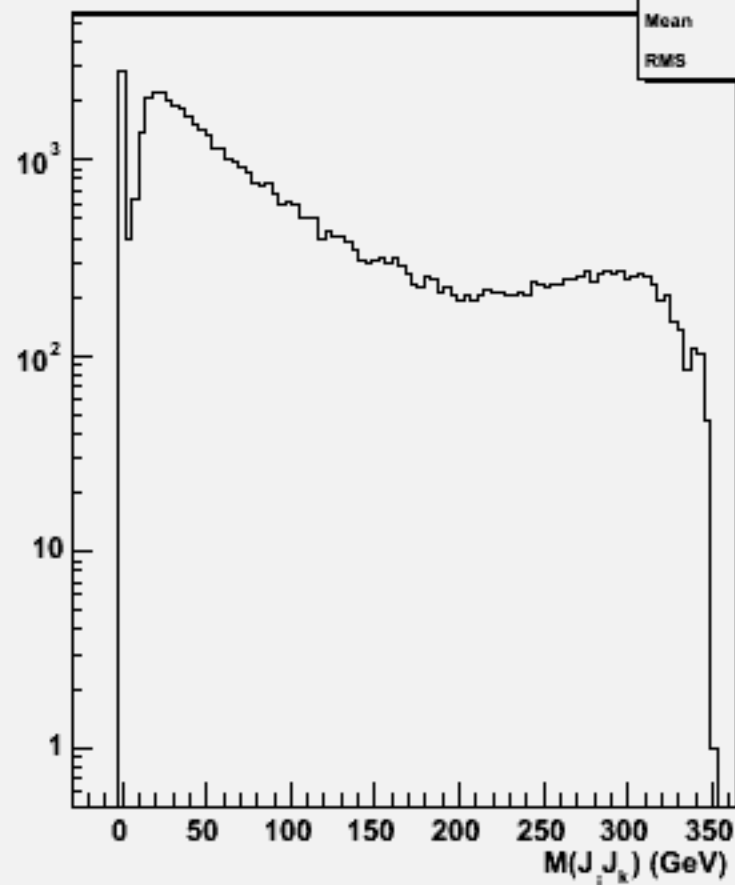
2jets mass(All comb)w102486 e1e1e2e2e3e3_o
