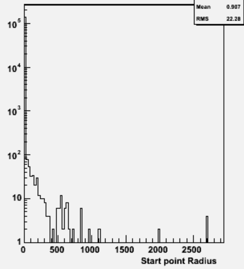
Start point R : w102486 e1e1e2e2e3e3_o
