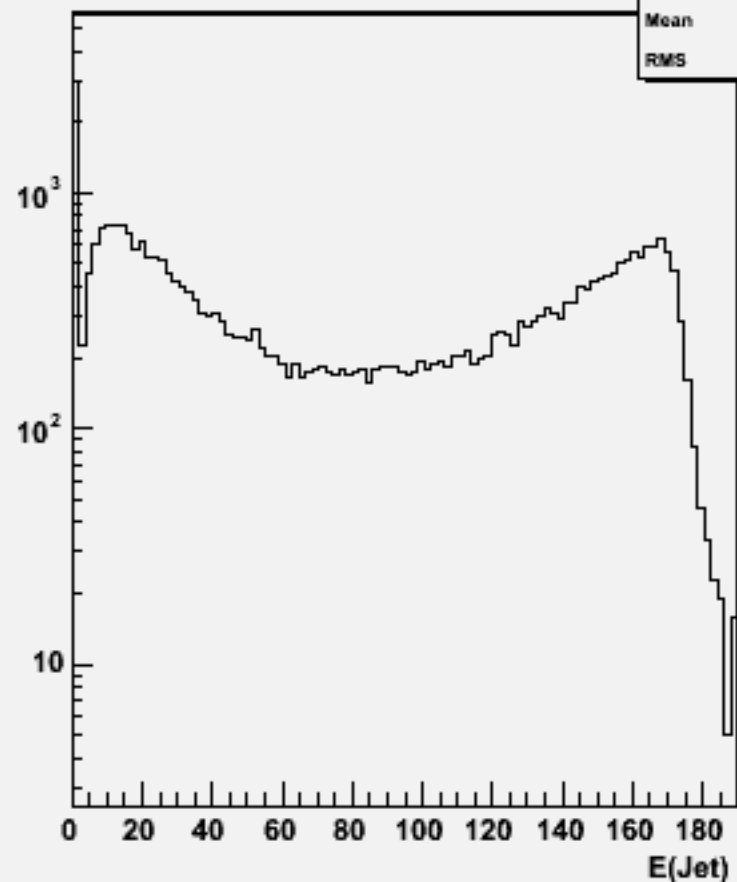
Jet energies(All jets)w102486 e1e1e2e2e3e3_o
