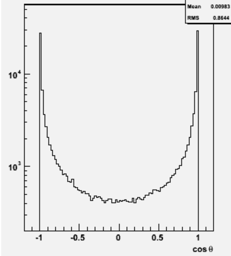
Particle cos θ : w102486 e1e1e2e2e3e3_o
