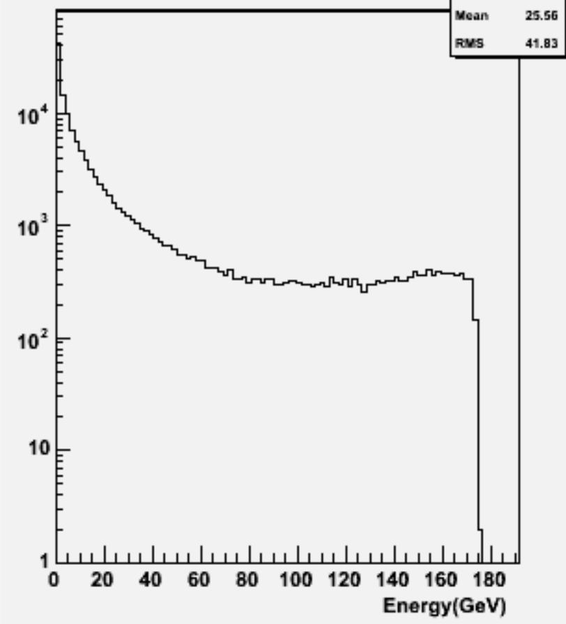
Start point R : w102485 e1e1e2e2e3e3_o
