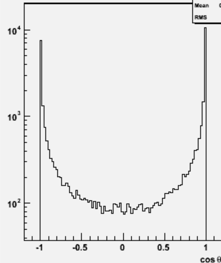
Jet cos \theta (All jets)w102485 e1e1e2e2e3e3_o
