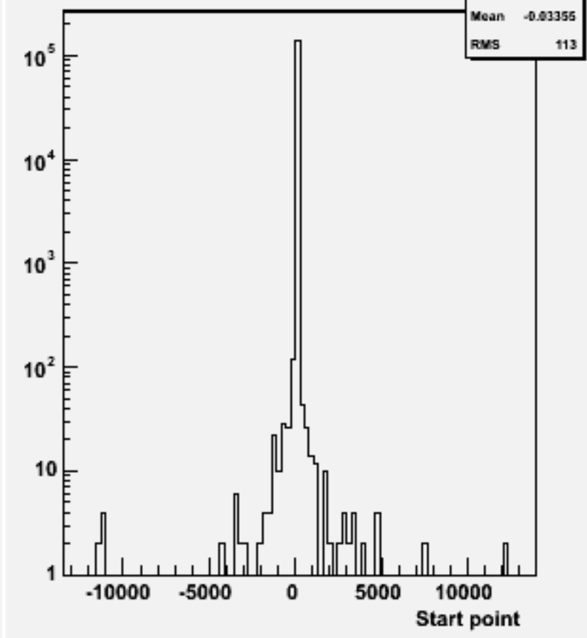
Start point Z : w102485 e1e1e2e2e3e3_o
