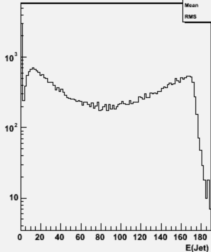
Jet energies(All jets)w102485 e1e1e2e2e3e3_o
