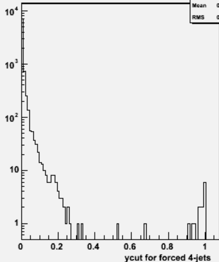
Ycut for 4-jets :w102485 e1e1e2e2e3e3_o
