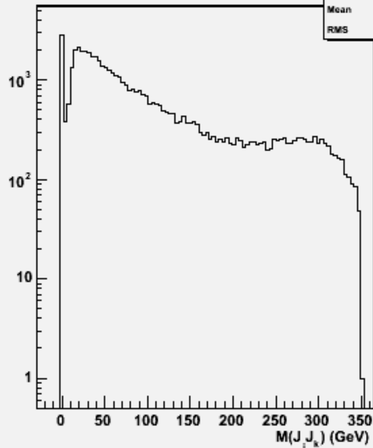
2jets mass(All comb)w102485 e1e1e2e2e3e3_o
