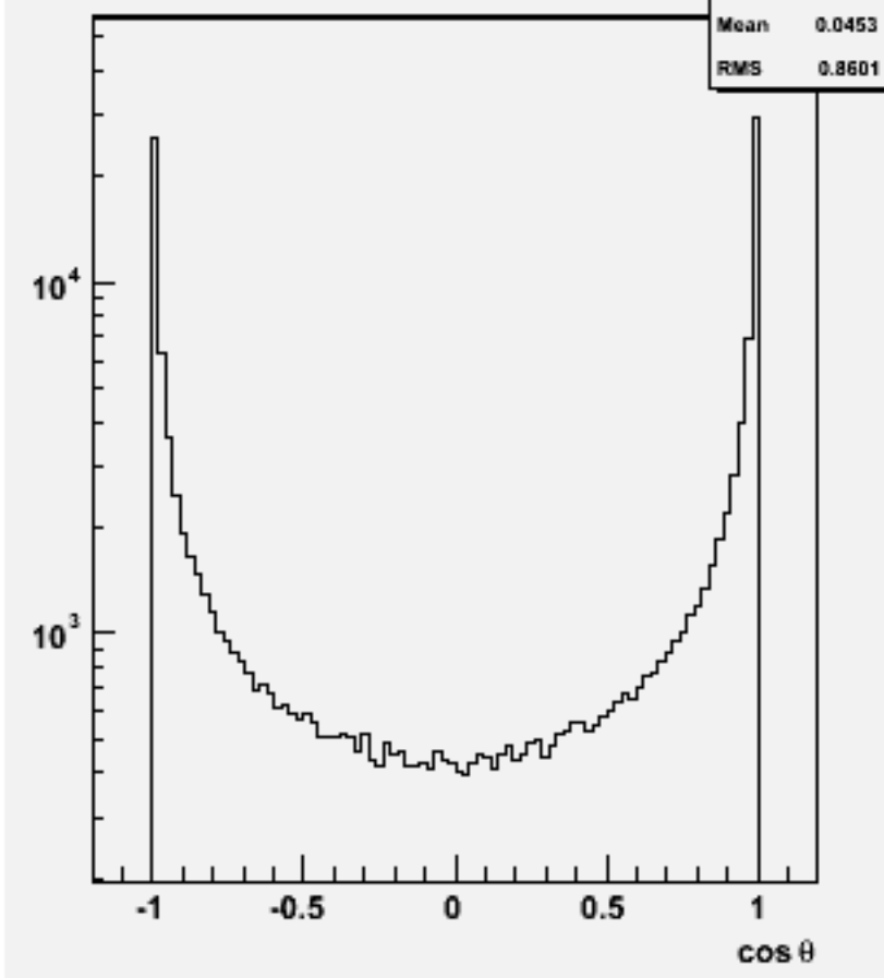
Particle cos \theta : w102485 e1e1e2e2e3e3_o
