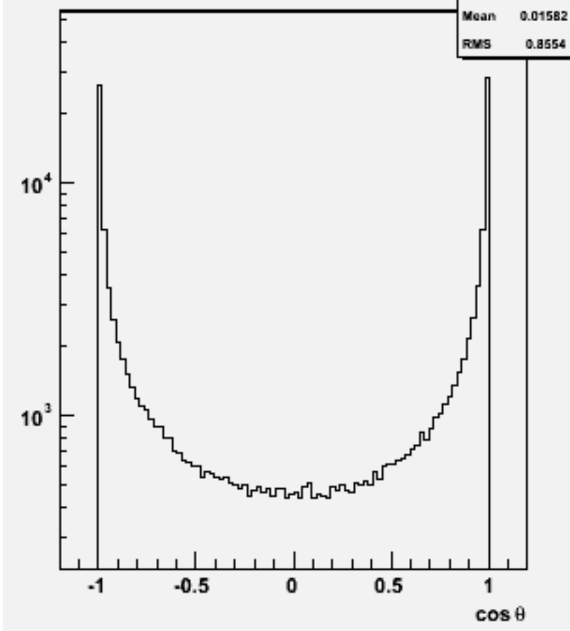
Particle cos \theta : w102484 e1e1e2e2e3e3_o
