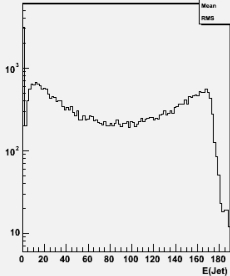
Jet energies(All jets)w102484 e1e1e2e2e3e3_o
