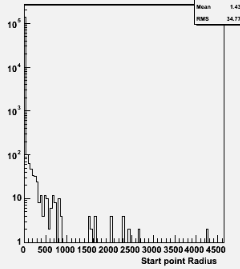
Start point R : w102484 e1e1e2e2e3e3_o
