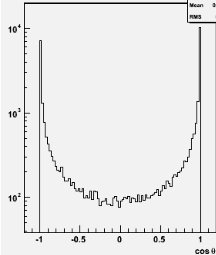
Jet cos \theta (All jets)w102484 e1e1e2e2e3e3_o
