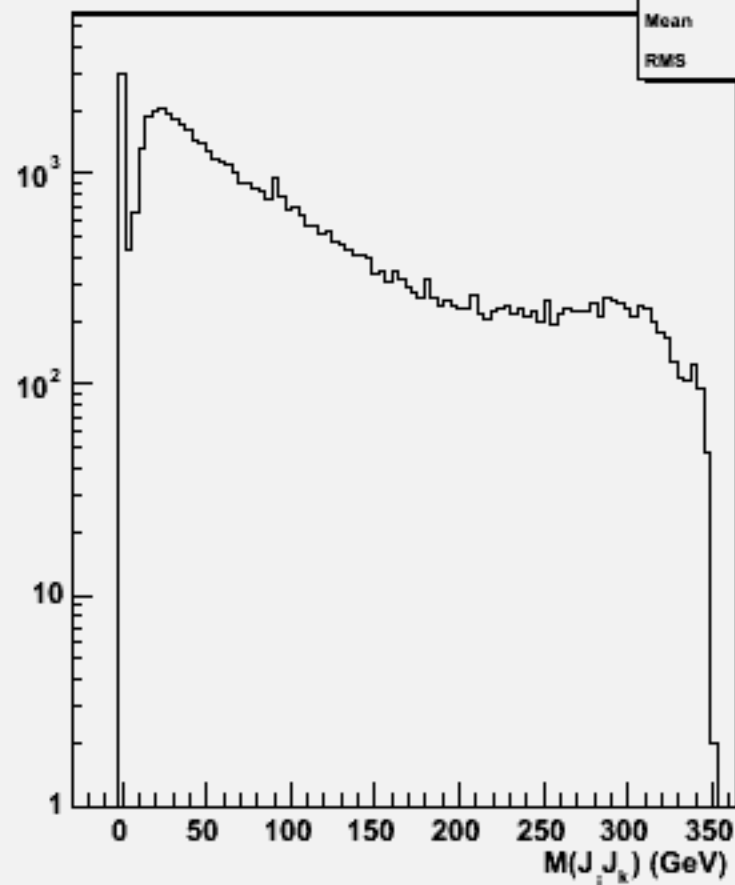
2jets mass(All comb)w102484 e1e1e2e2e3e3_o
