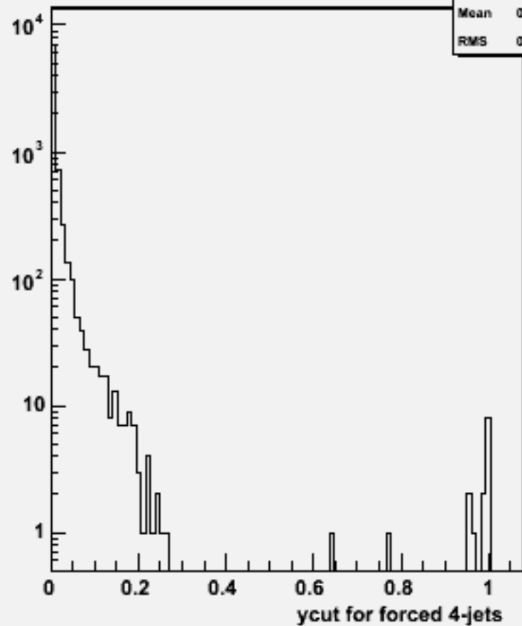
Ycut for 4-jets :w102484 e1e1e2e2e3e3_o
