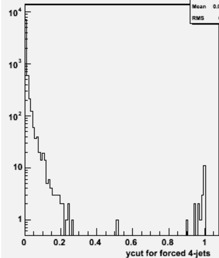
Ycut for 4-jets :w102483 e1e1e2e2e3e3_o
