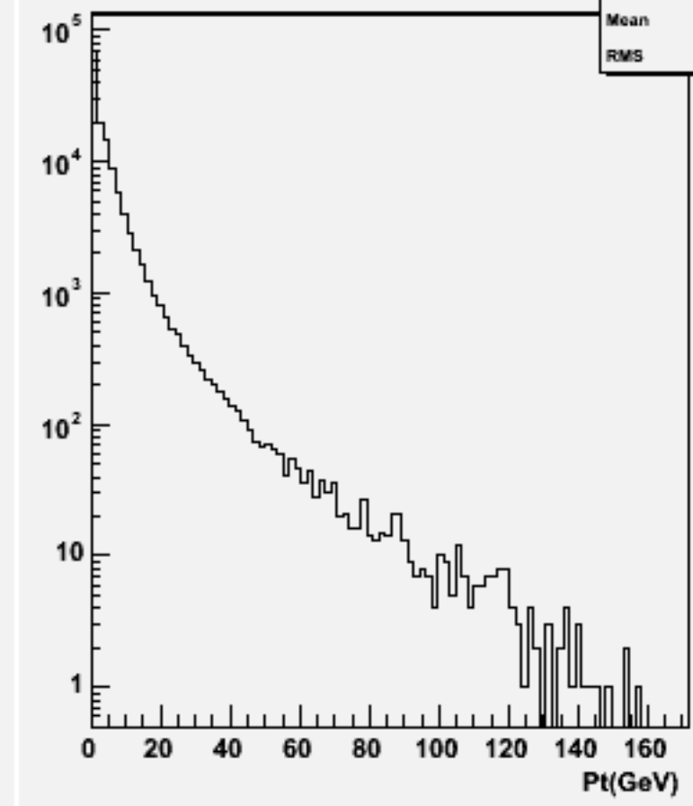
Start point Z : w102483 e1e1e2e2e3e3_o
