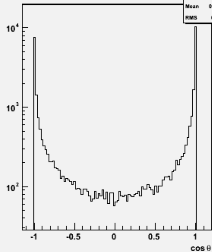
Jet cos \theta (All jets)w102483 e1e1e2e2e3e3_o
