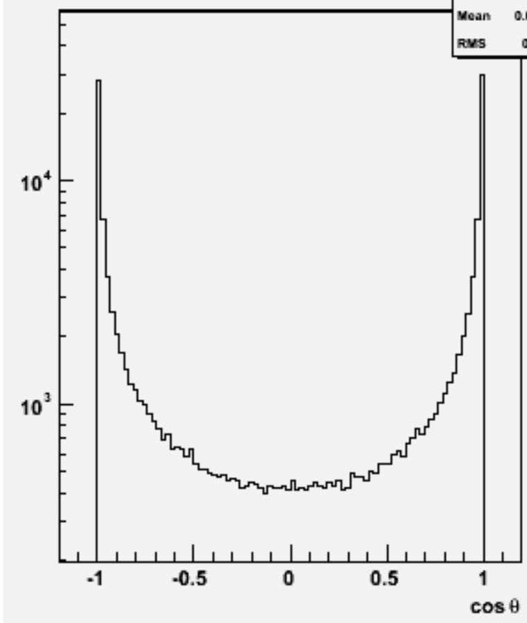
Particle cos \theta : w102483 e1e1e2e2e3e3_o
