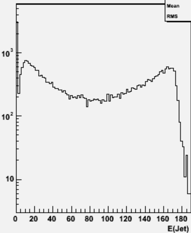
Jet energies(All jets)w102483 e1e1e2e2e3e3_o
