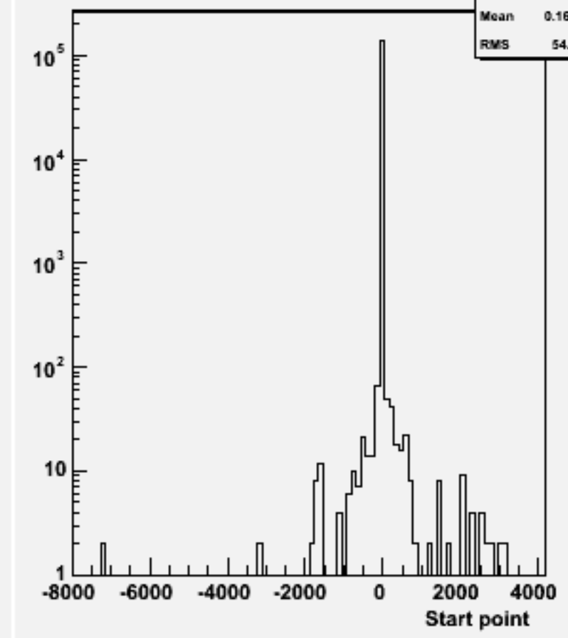
Start point Z : w102483 e1e1e2e2e3e3_o
