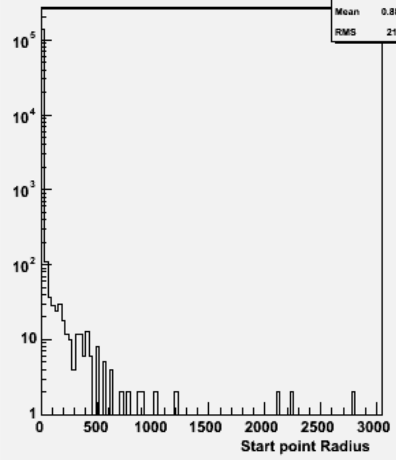
Start point R : w102483 e1e1e2e2e3e3_o
