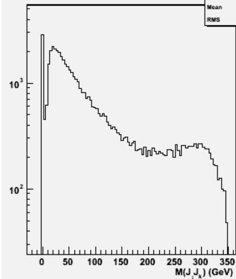
2jets mass(All comb)w102483 e1e1e2e2e3e3_o
