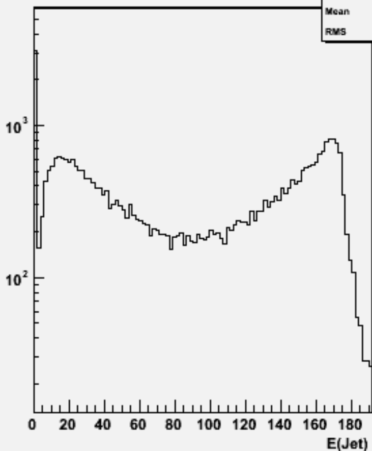
Jet energies(All jets)w102482 e1e1e2e2e2e2_o
