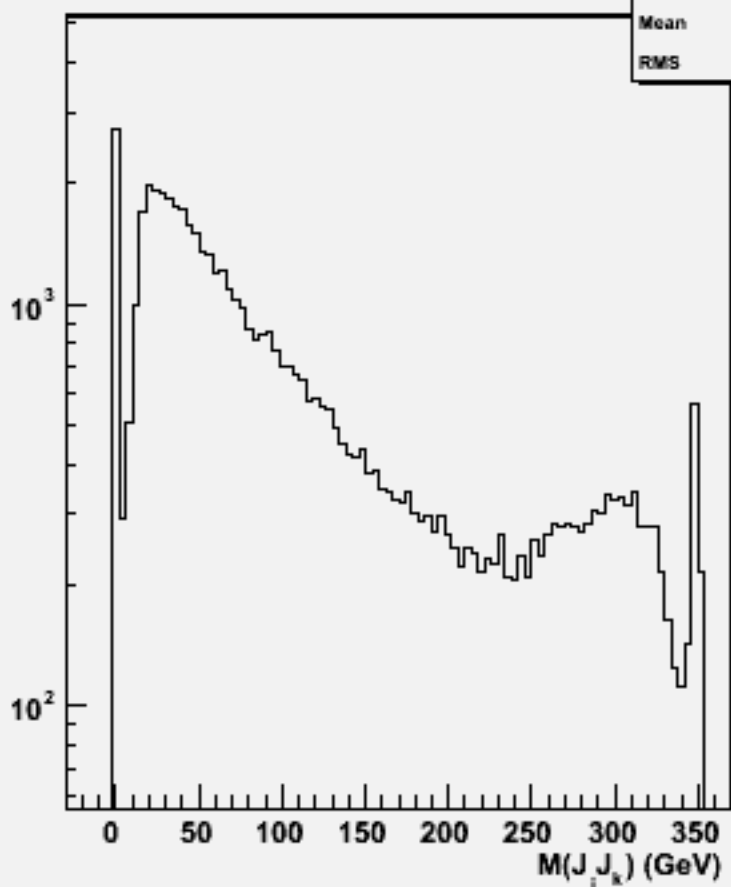
2jets mass(All comb)w102482 e1e1e2e2e2e2_o
