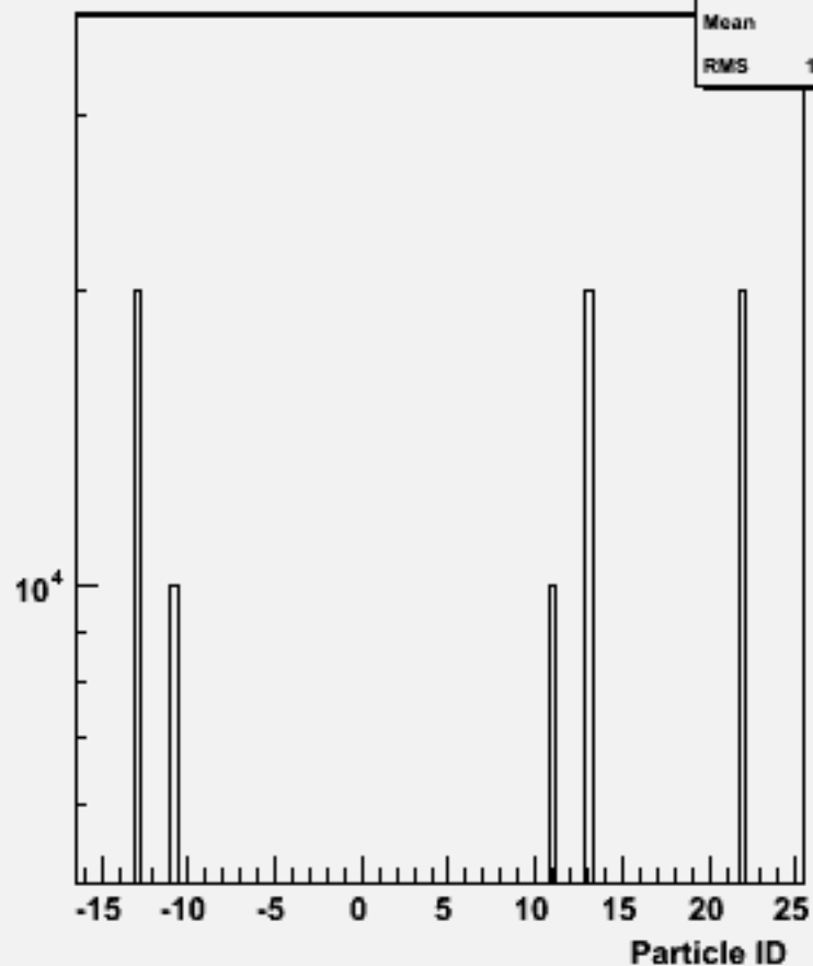
Particle ID : w102482 e1e1e2e2e2e2_o
