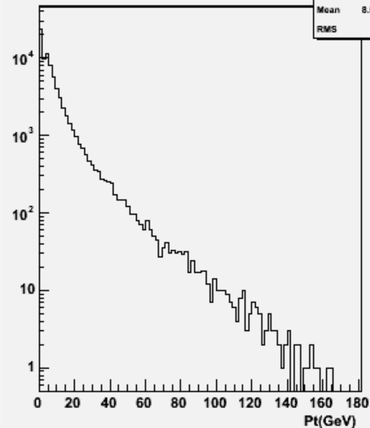
Particle Pt : w102482 e1e1e2e2e2e2_o
