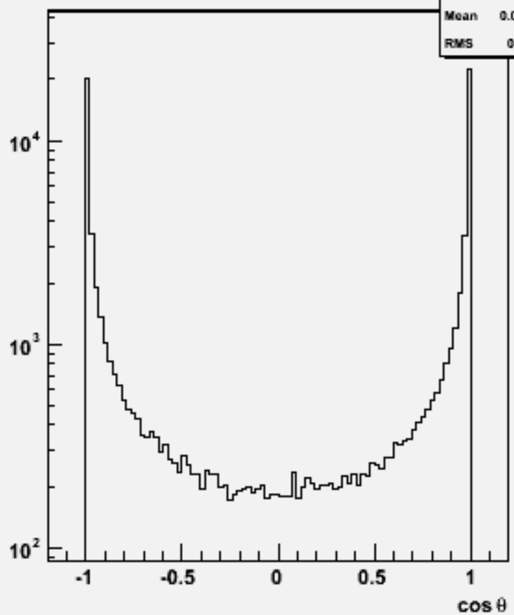
Particle cos \theta : w102482 e1e1e2e2e2e2_o
