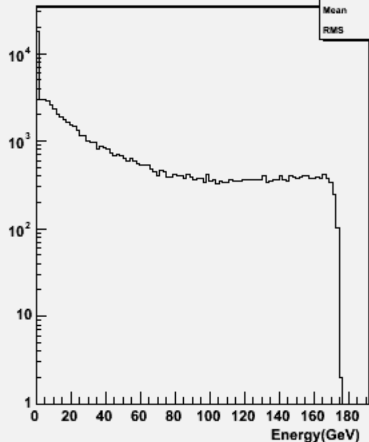
Particle Energy : w102482 e1e1e2e2e2e2_o
