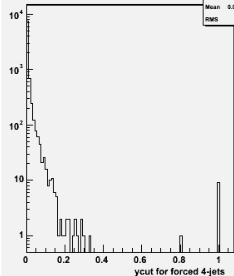
Ycut for 4-jets :w102482 e1e1e2e2e2e2_o
