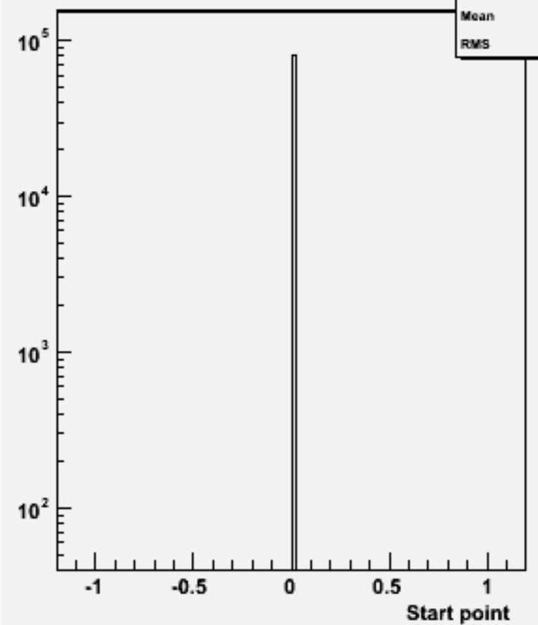
Start point Z : w102482 e1e1e2e2e2e2_o
