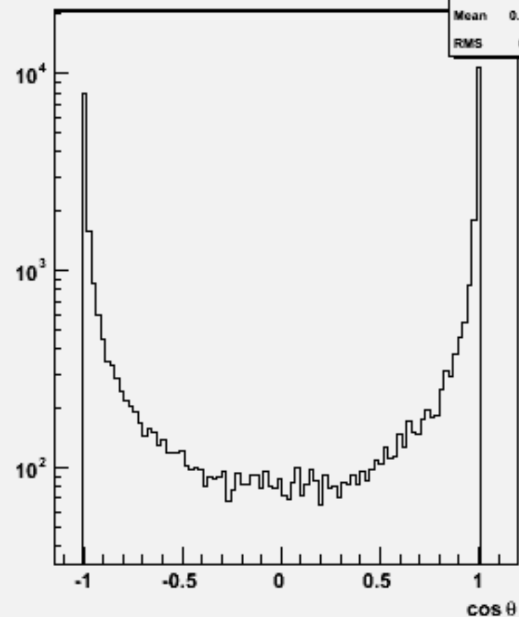
Jet cos \theta (All jets)w102482 e1e1e2e2e2e2_o
