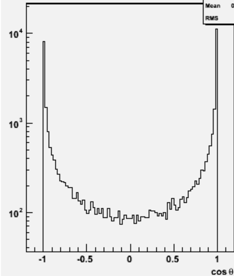
Jet cos \theta (All jets)w102481 e1e1e2e2e2e2_o
