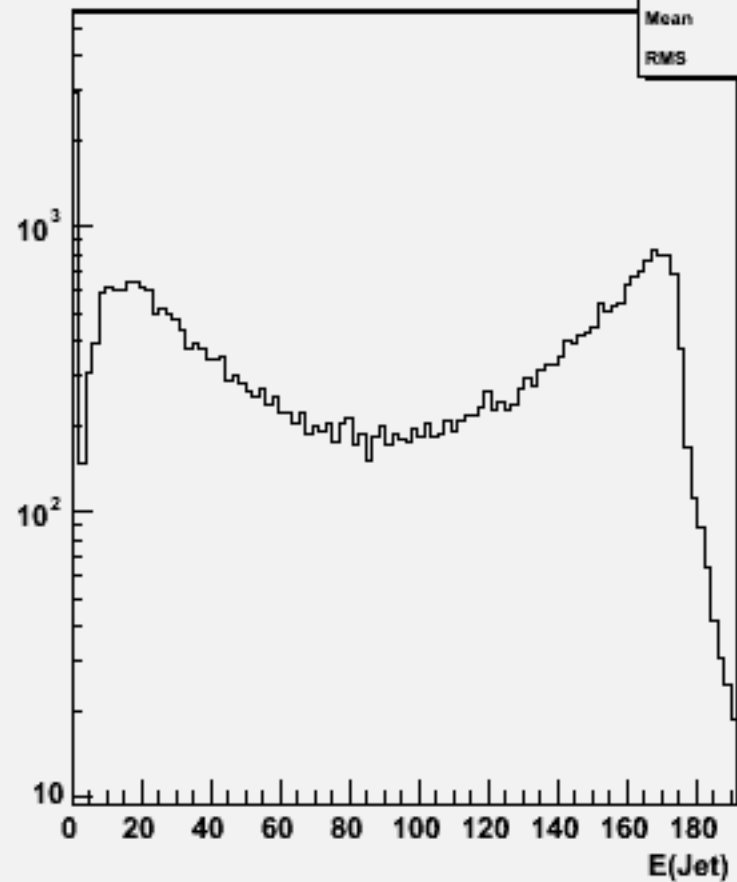
Jet energies(All jets)w102481 e1e1e2e2e2e2_o
