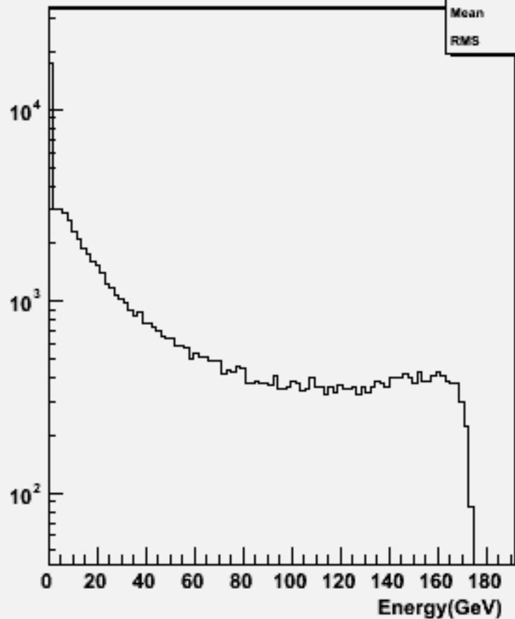
Start point R : w102481 e1e1e2e2e2e2_o
