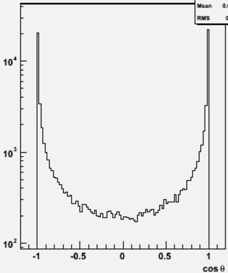
Particle cos \theta : w102481 e1e1e2e2e2e2_o
