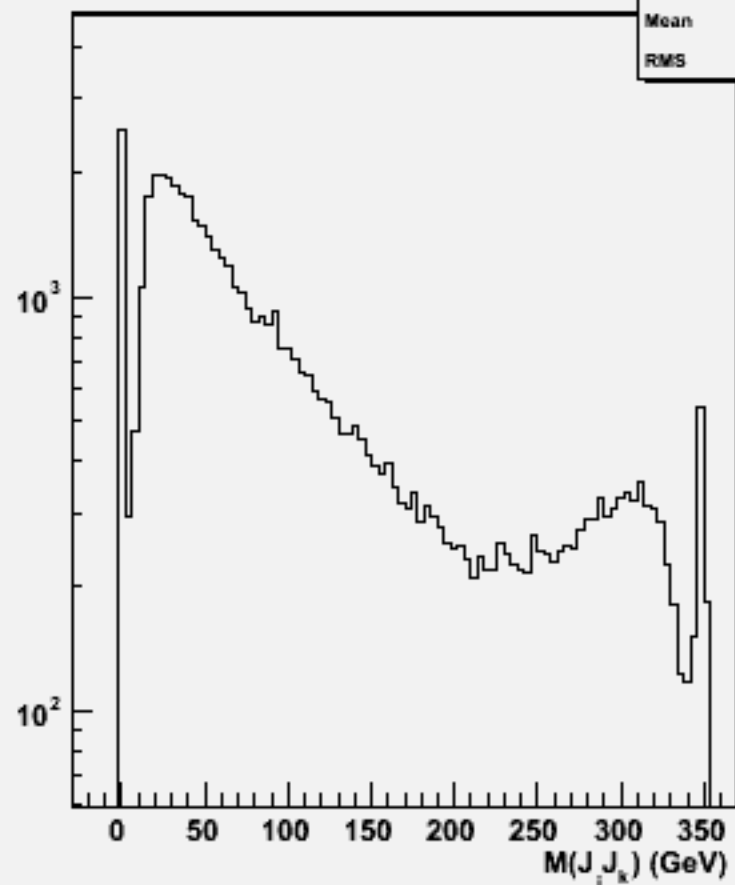
2jets mass(All comb)w102481 e1e1e2e2e2e2_o
