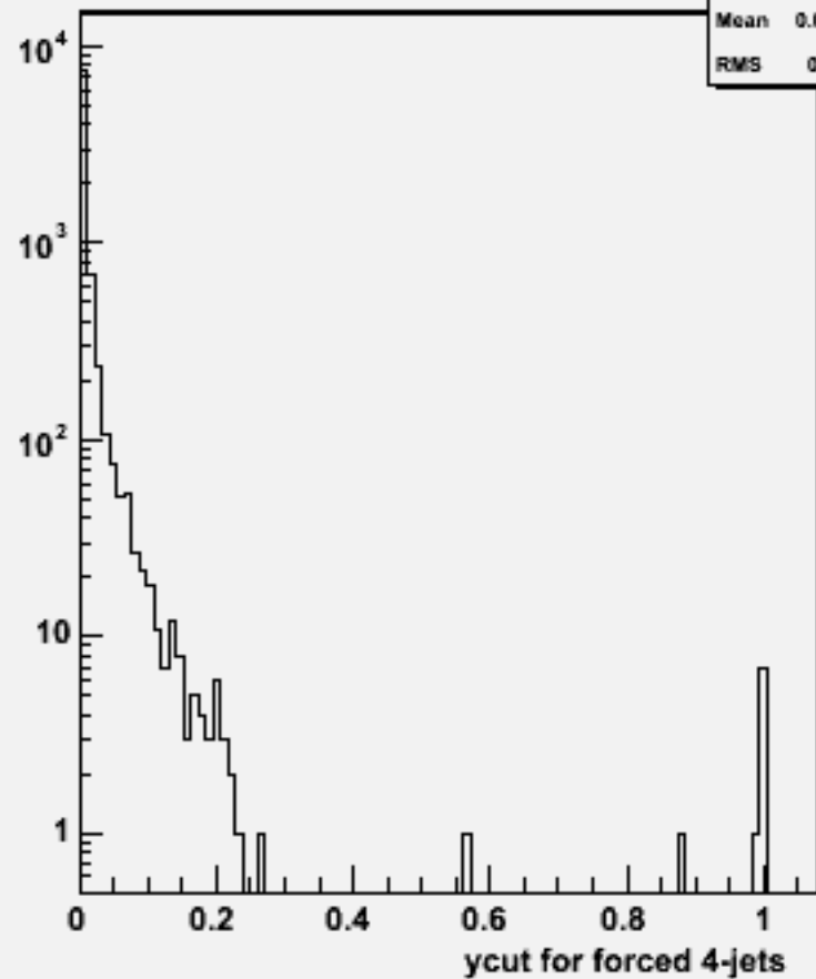
Ycut for 4-jets :w102481 e1e1e2e2e2e2_o
