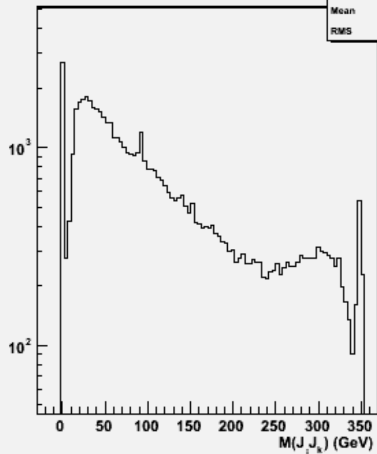
2jets mass(All comb)w102480 e1e1e2e2e2e2_o
