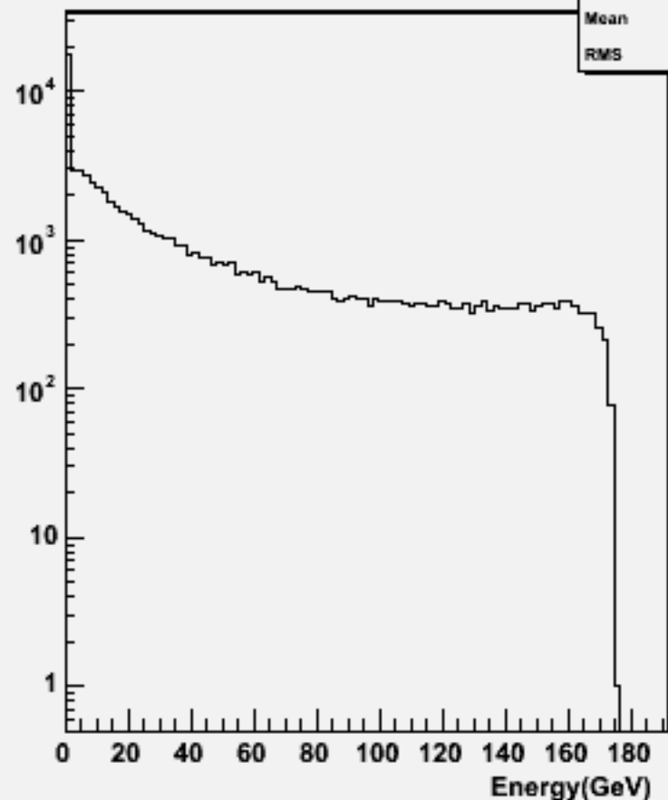
Particle Energy : w102480 e1e1e2e2e2e2_o
