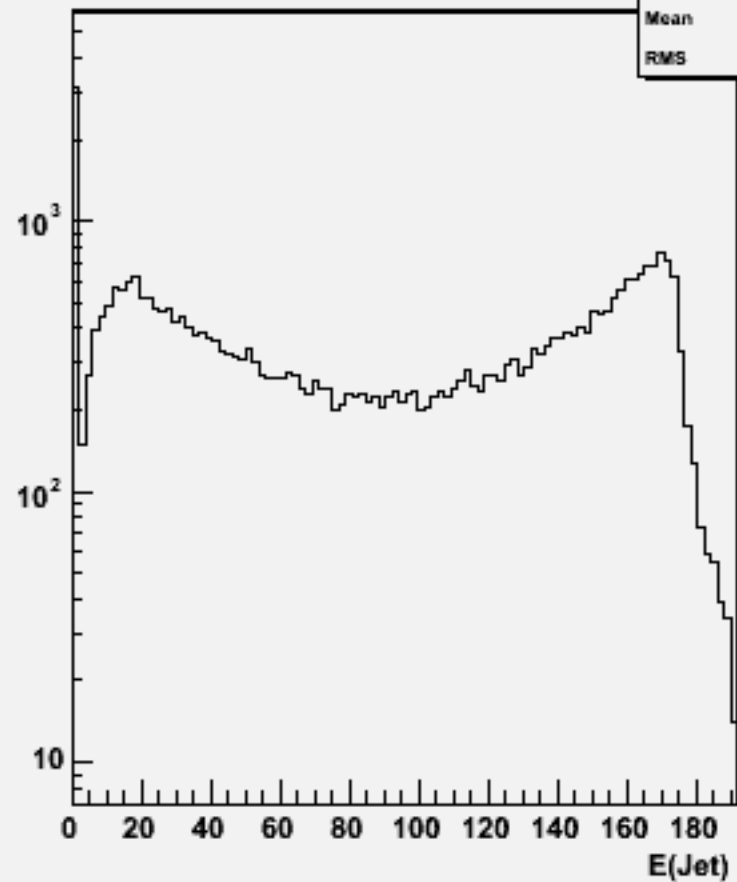
Jet energies(All jets)w102480 e1e1e2e2e2e2_o
