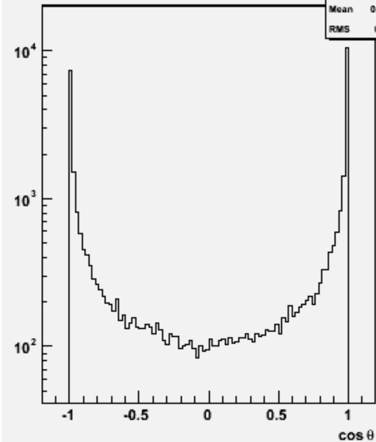
Jet cos \theta (All jets)w102480 e1e1e2e2e2e2_o
