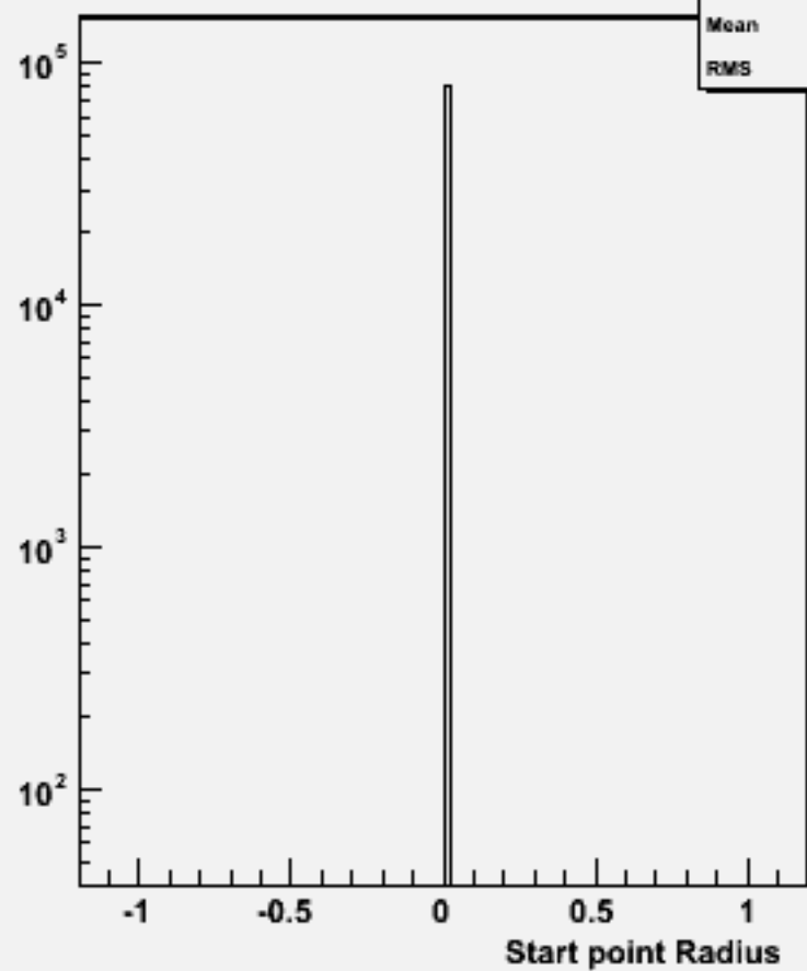
Start point R : w102480 e1e1e2e2e2e2_o
