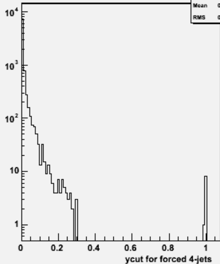
Ycut for 4-jets :w102480 e1e1e2e2e2e2_o
