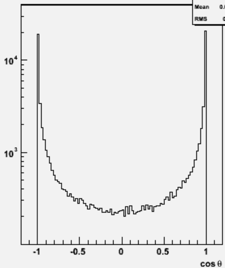
Particle cos \theta : w102480 e1e1e2e2e2e2_o
