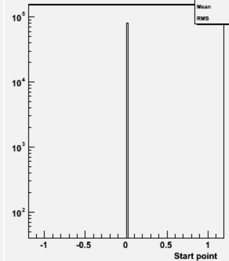
Start point Z : w102480 e1e1e2e2e2e2_o
