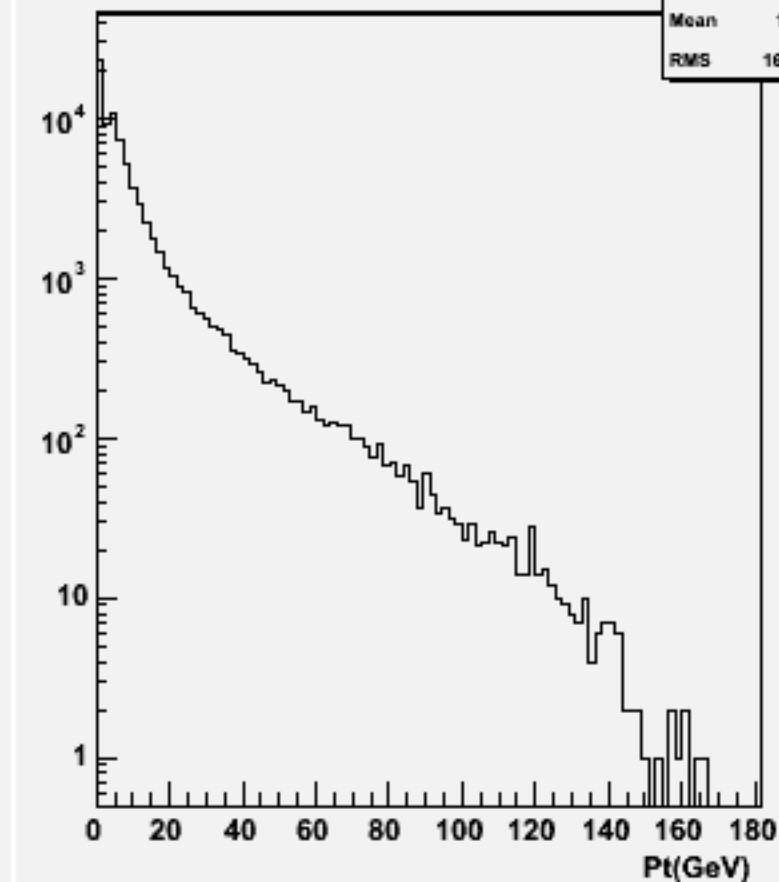
Particle Pt : w102480 e1e1e2e2e2e2_o
