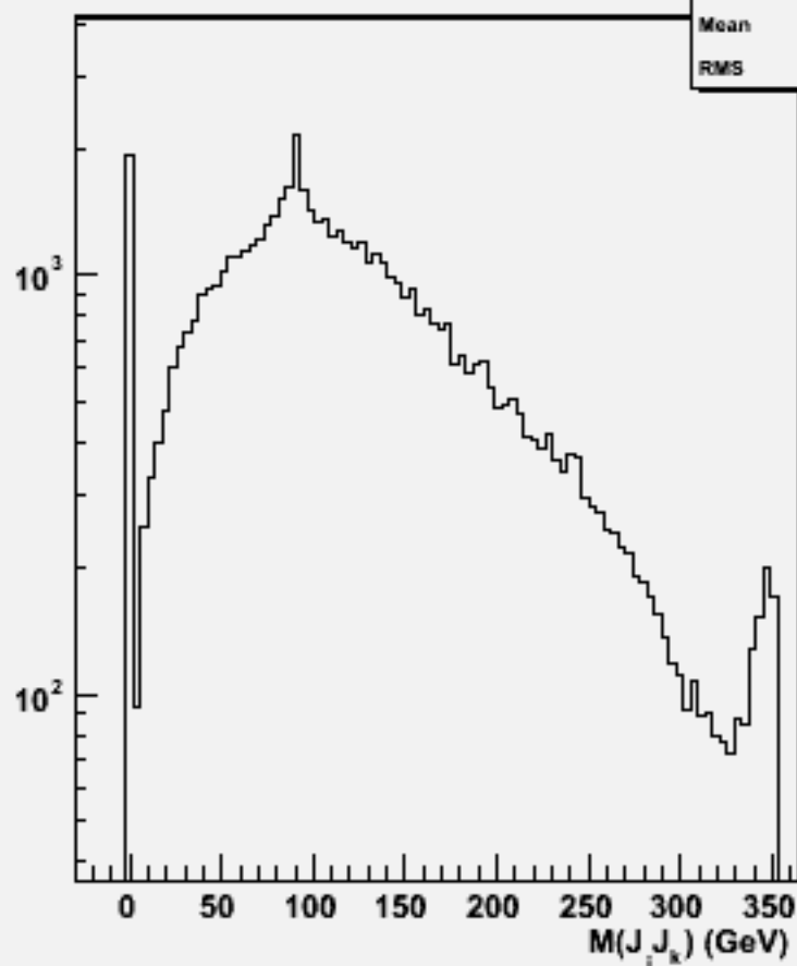
2jets mass(All comb)w102477 e1e1e1e1bb_o
