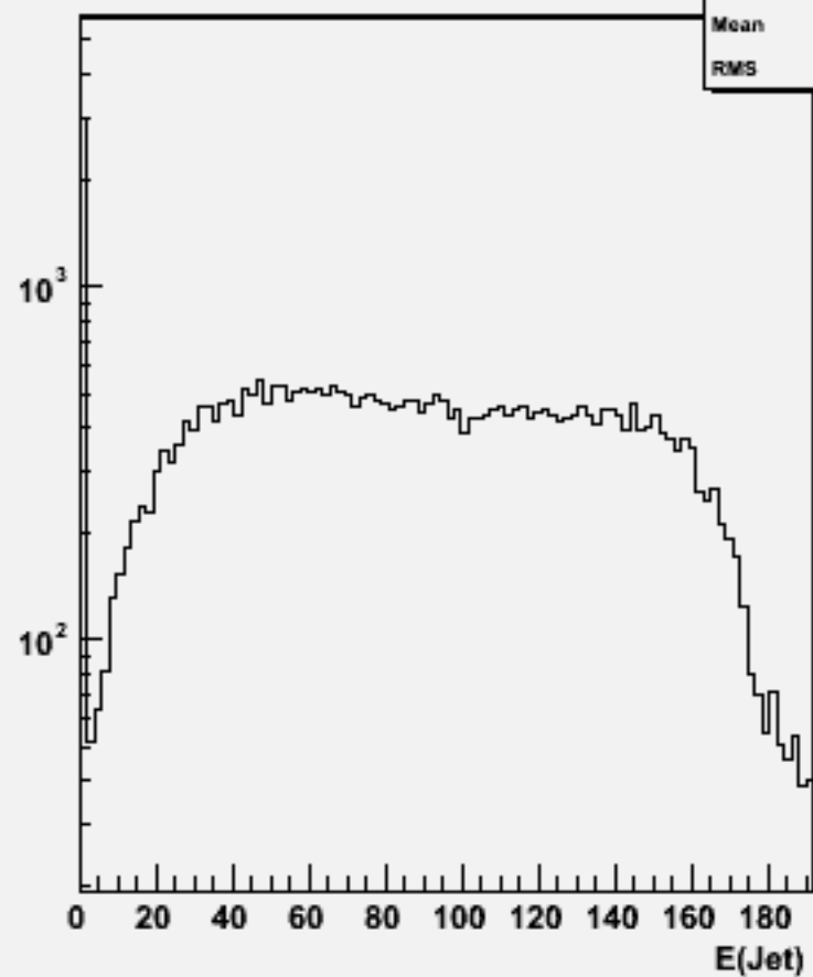
Jet energies(All jets)w102477 e1e1e1e1bb_o
