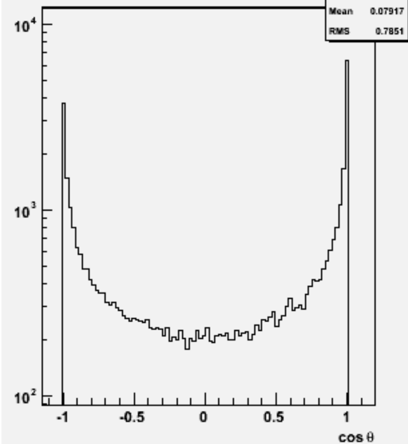
Jet cos \theta (All jets)w102477 e1e1e1e1bb_o
