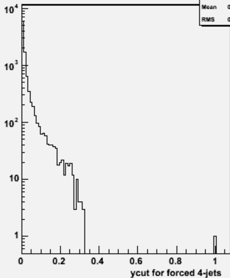
Ycut for 4-jets :w102477 e1e1e1e1bb_o
