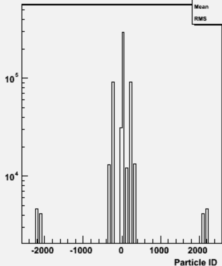
Particle ID : w102476 e1e1e1e1bb_o
