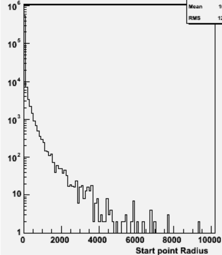
Start point R : w102476 e1e1e1e1bb_o
