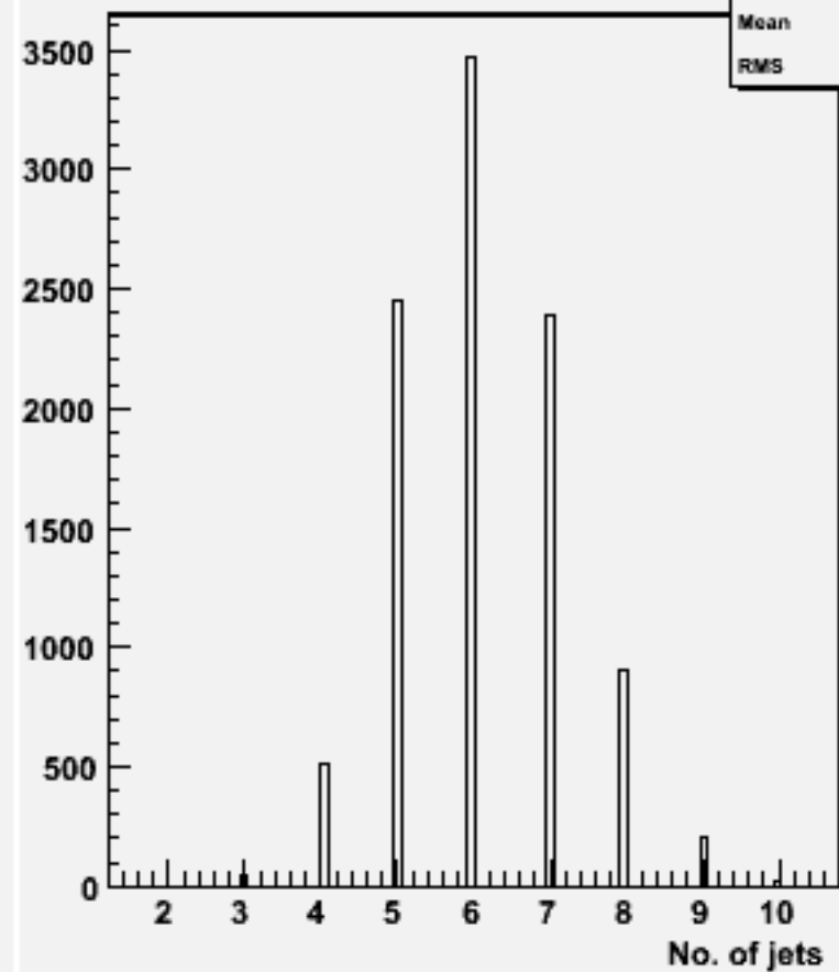
No. jets (ycut=0.001) : w102476 e1e1e1e1bb_o
