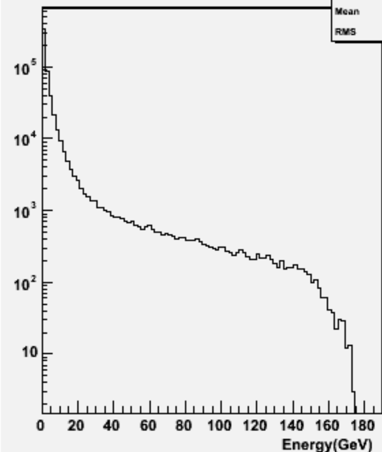
Particle Energy : w102476 e1e1e1e1bb_o
