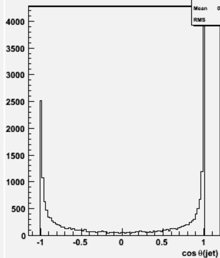
cos \theta for 2-jets :w102476 e1e1e1e1bb_o
