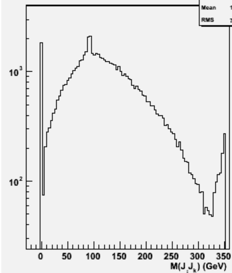
2jets mass(All comb)w102476 e1e1e1e1bb_o
