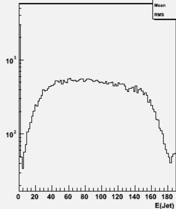
Jet energies(All jets)w102476 e1e1e1e1bb_o
