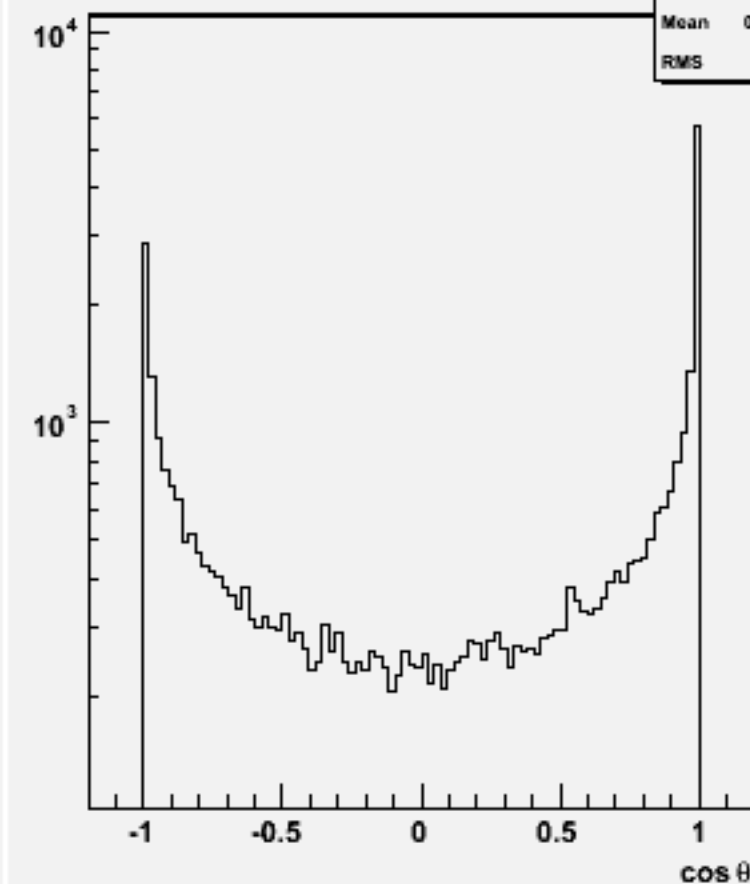
Jet cos \theta (All jets)w102476 e1e1e1e1bb_o
