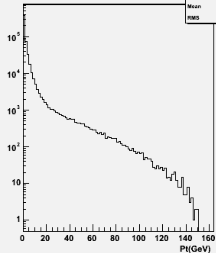
Particle Pt : w102476 e1e1e1e1bb_o
