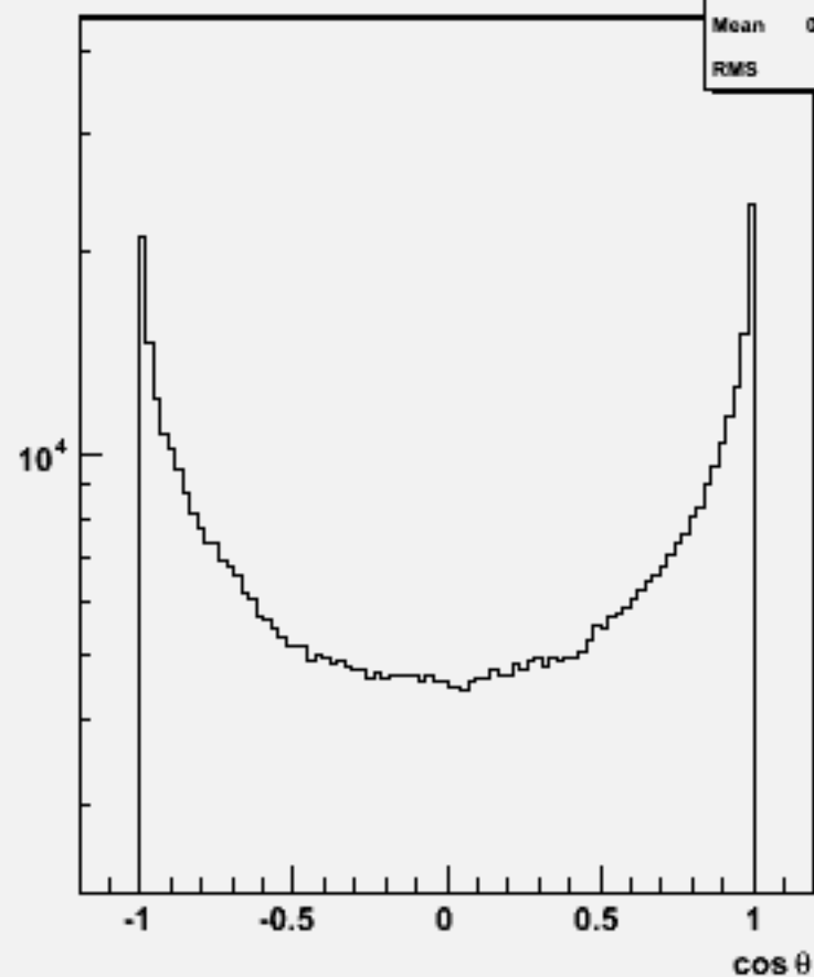
Particle cosθ : w102476 e1e1e1e1bb_o
