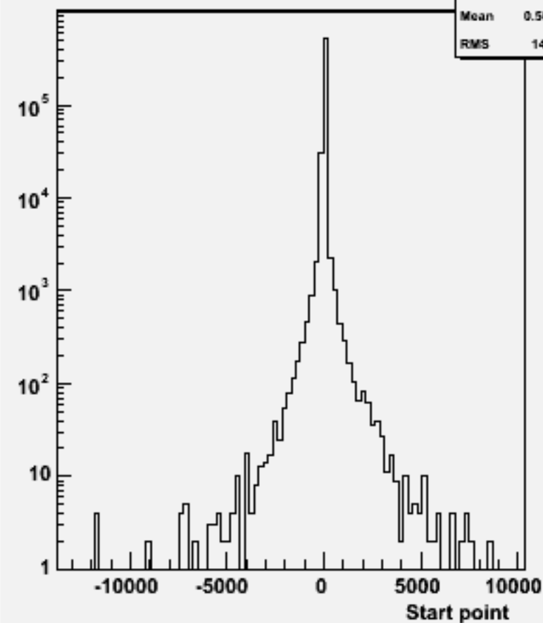
Start point Z : w102476 e1e1e1e1bb_o
