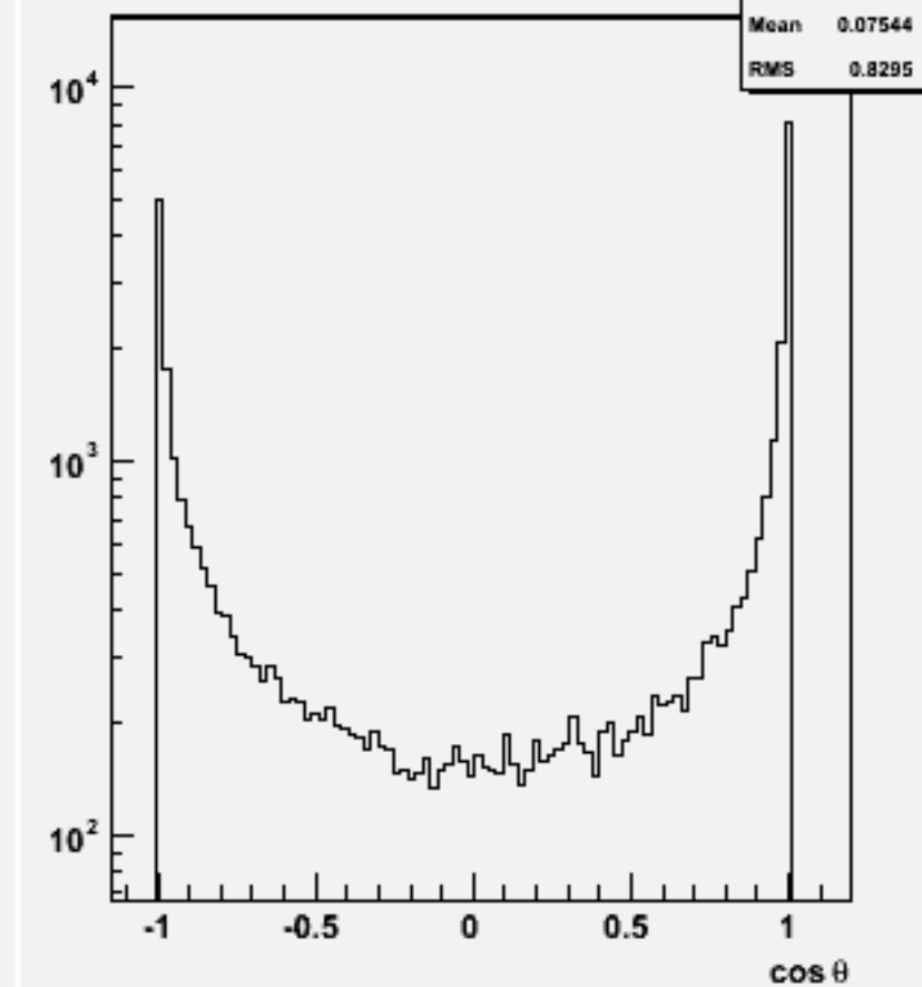
Jet cos \theta (All jets)w102474 e1e1e1e1ss_o
