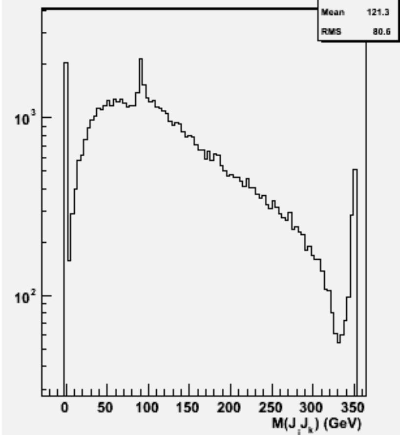
2jets mass(All comb)w102474 e1e1e1e1ss_o
