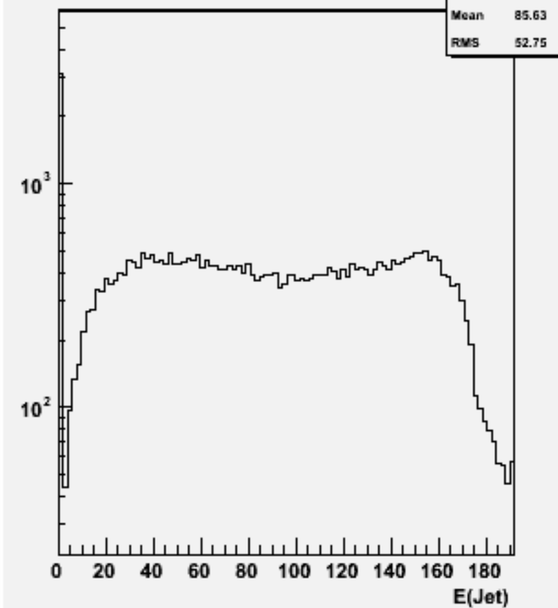
Jet energies(All jets)w102474 e1e1e1e1ss_o
