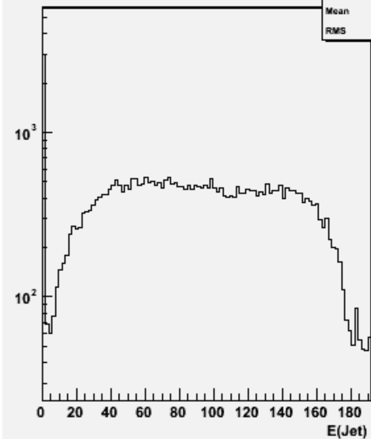
Jet energies(All jets)w102473 e1e1e1e1ss_o
