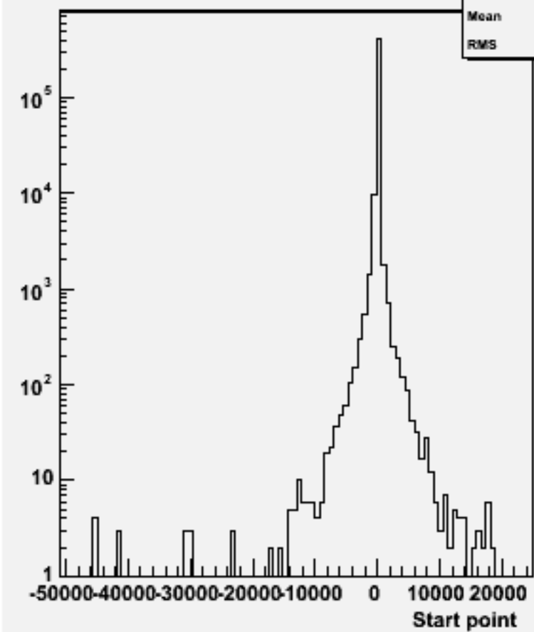
Start point Z : w102473 e1e1e1e1ss_o
