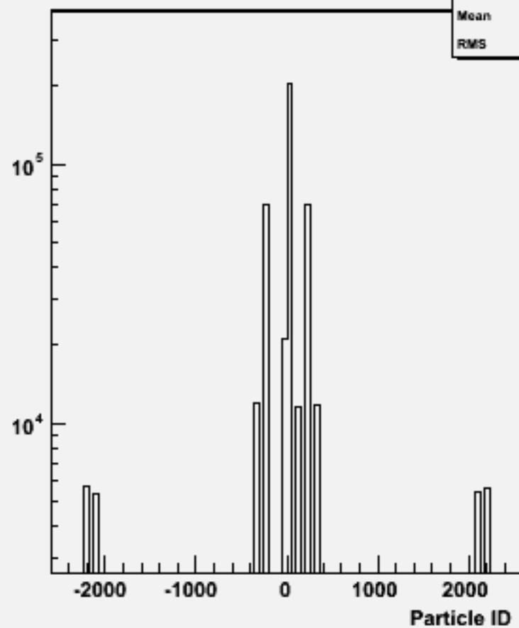
Particle ID : w102473 e1e1e1e1ss_o
