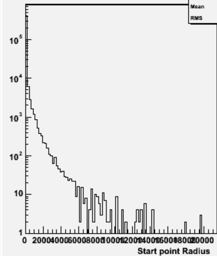
Start point R : w102473 e1e1e1e1ss_o
