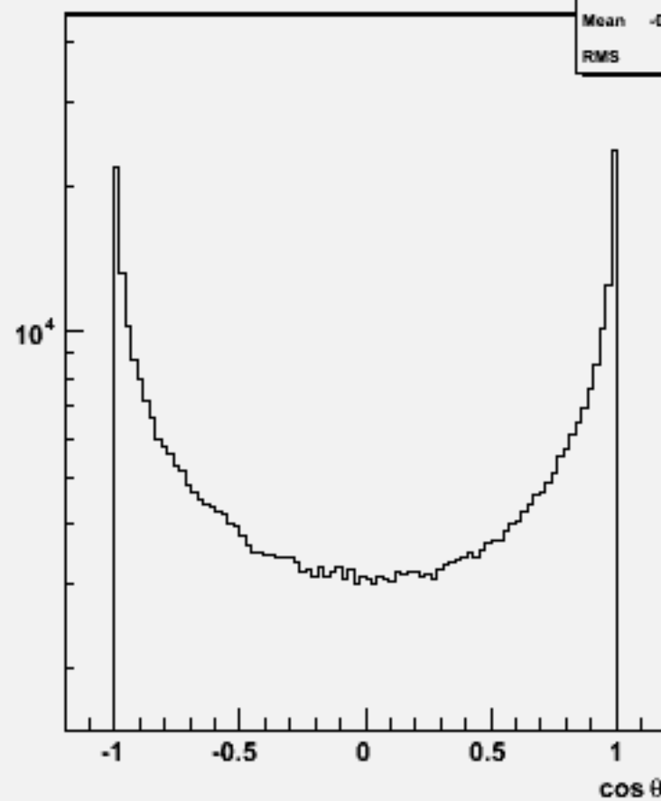
Particle cosθ : w102473 e1e1e1e1ss_o
