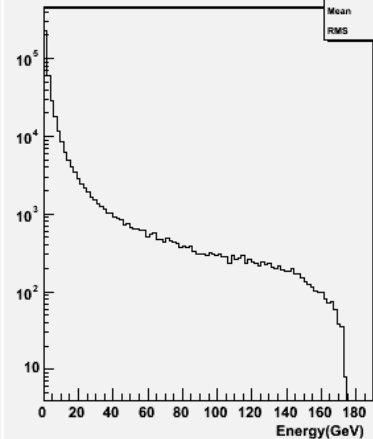
Particle Energy : w102473 e1e1e1e1ss_o
