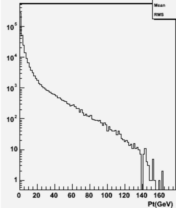
Particle Pt : w102473 e1e1e1e1ss_o
