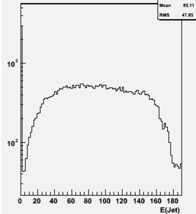
Jet energies(All jets)w102472 e1e1e1e1ss_o
