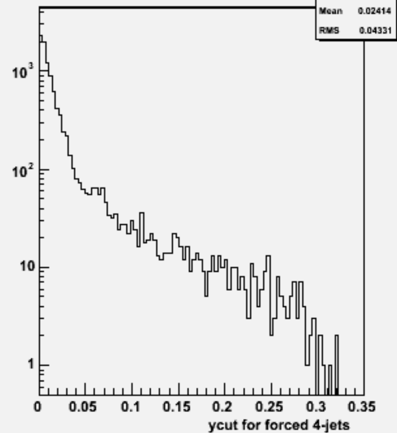
Ycut for 4-jets :w102472 e1e1e1e1ss_o
