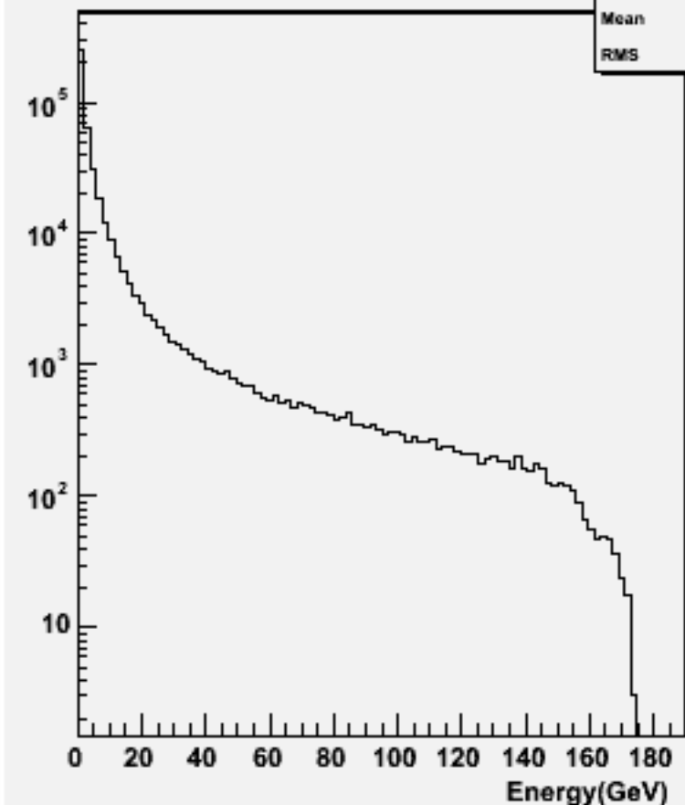
Particle Energy : w102472 e1e1e1e1ss_o
