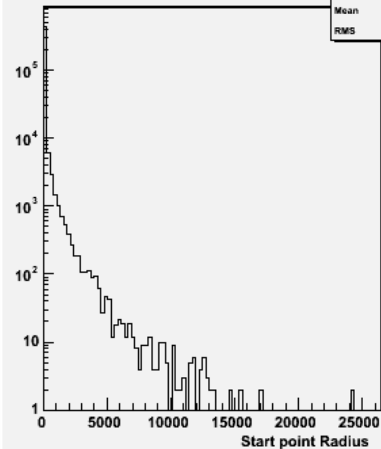
Start point R : w102472 e1e1e1e1ss_o
