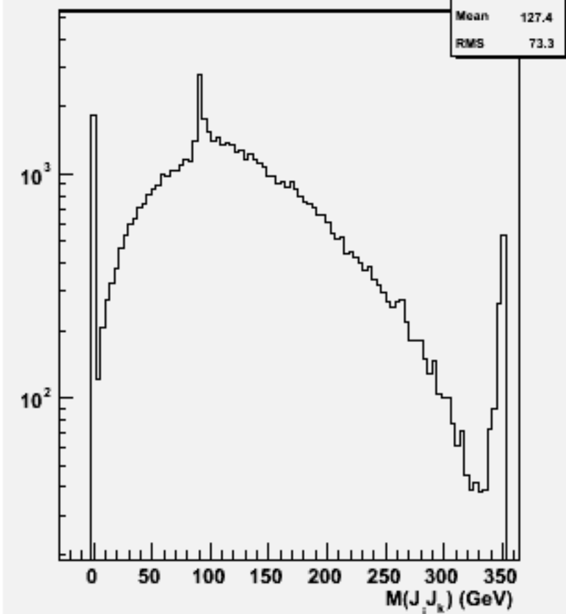
2jets mass(All comb)w102472 e1e1e1e1ss_o
