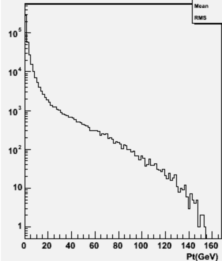
Particle Pt : w102472 e1e1e1e1ss_o
