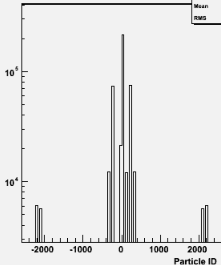
Particle ID : w102472 e1e1e1e1ss_o
