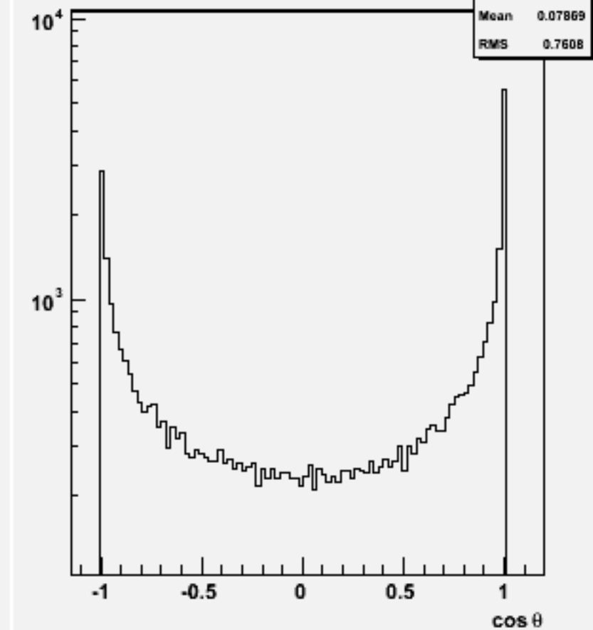
Jet cos \theta (All jets)w102472 e1e1e1e1ss_o
