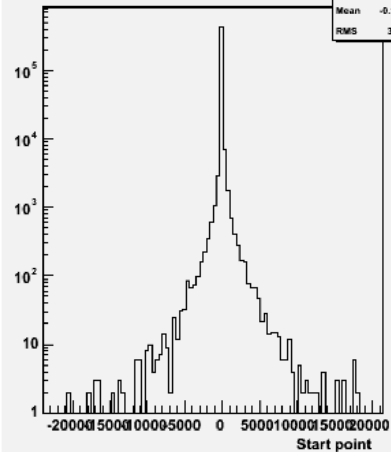
Start point Z : w102472 e1e1e1e1ss_o
