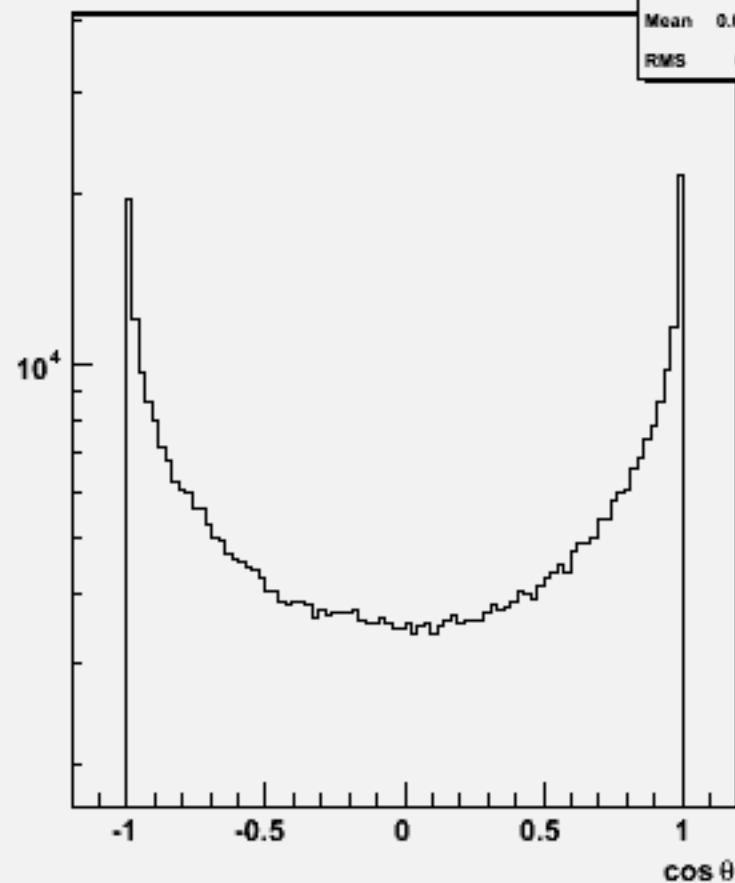
Particle cos \theta : w102472 e1e1e1e1ss_o
