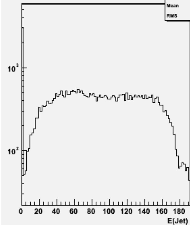
Jet energies(All jets)w102469 e1e1e1e1dd_o
