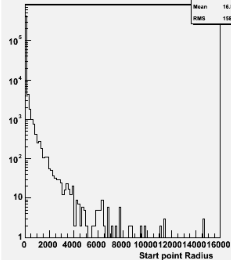
Start point R : w102469 e1e1e1e1dd_o
