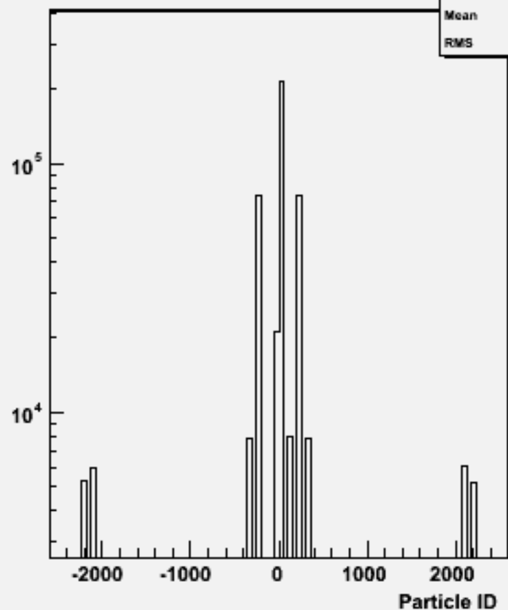
Particle ID : w102469 e1e1e1e1dd_o
