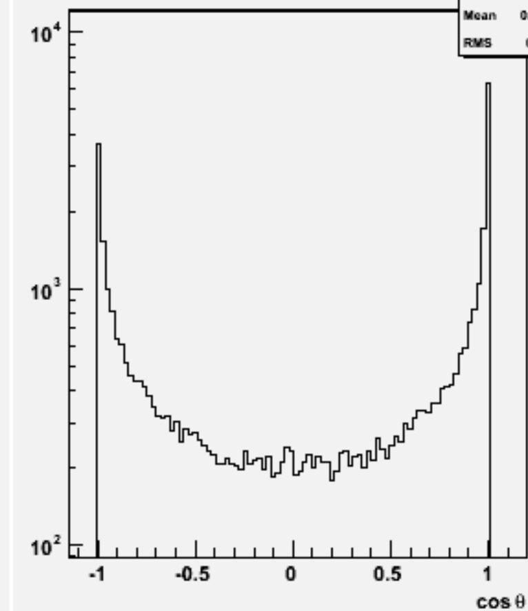
Jet cos \theta (All jets)w102469 e1e1e1e1dd_o
