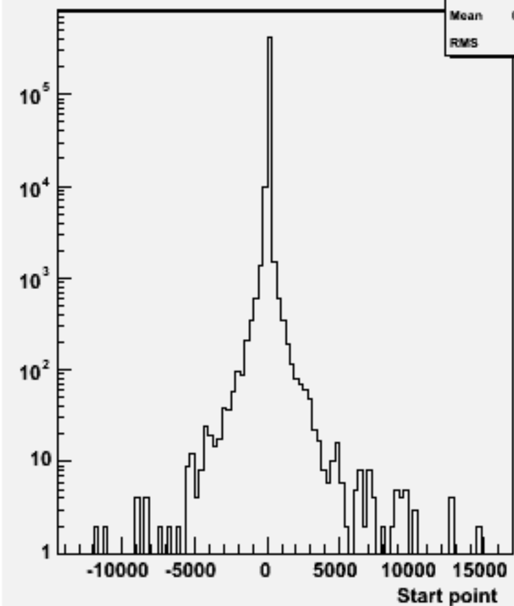
Start point Z : w102469 e1e1e1e1dd_o
