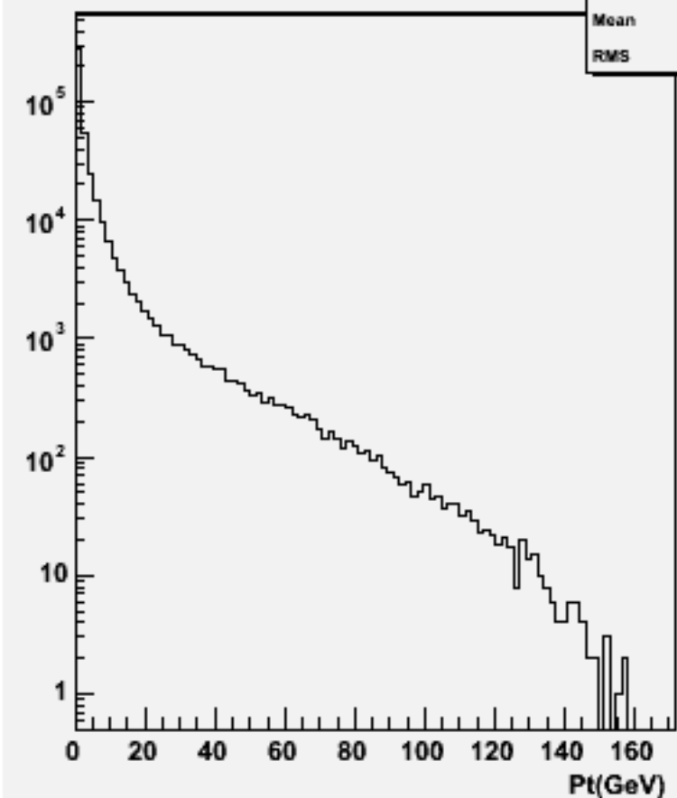
Particle Pt : w102469 e1e1e1e1dd_o
