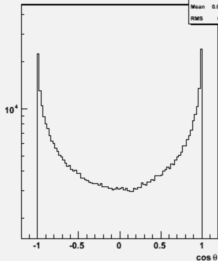
Particle cos \theta : w102469 e1e1e1e1dd_o
