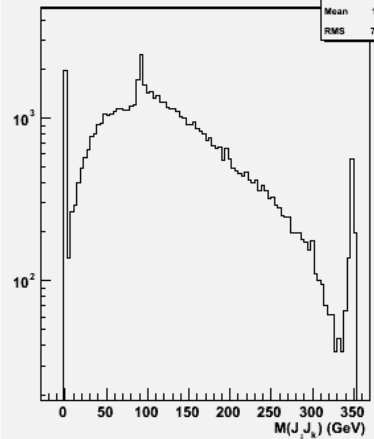
2jets mass(All comb)w102469 e1e1e1e1dd_o
