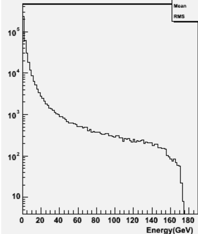
Particle Energy : w102469 e1e1e1e1dd_o
