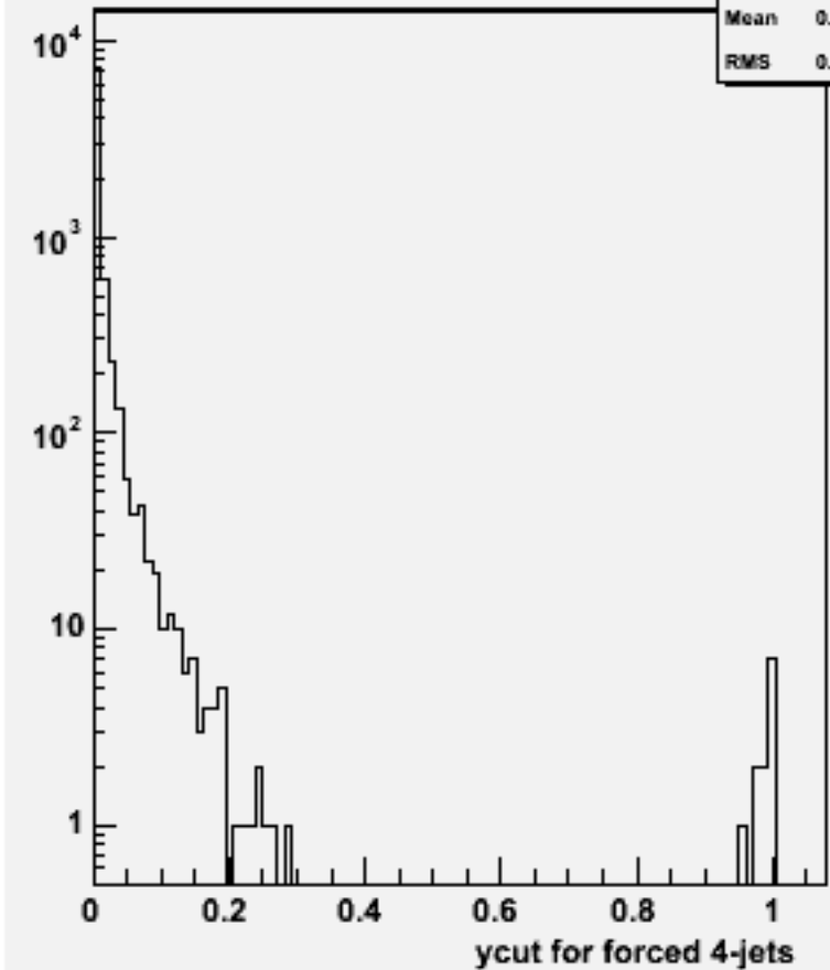
Ycut for 4-jets :w102466 e1e1e1e1e3e3_o
