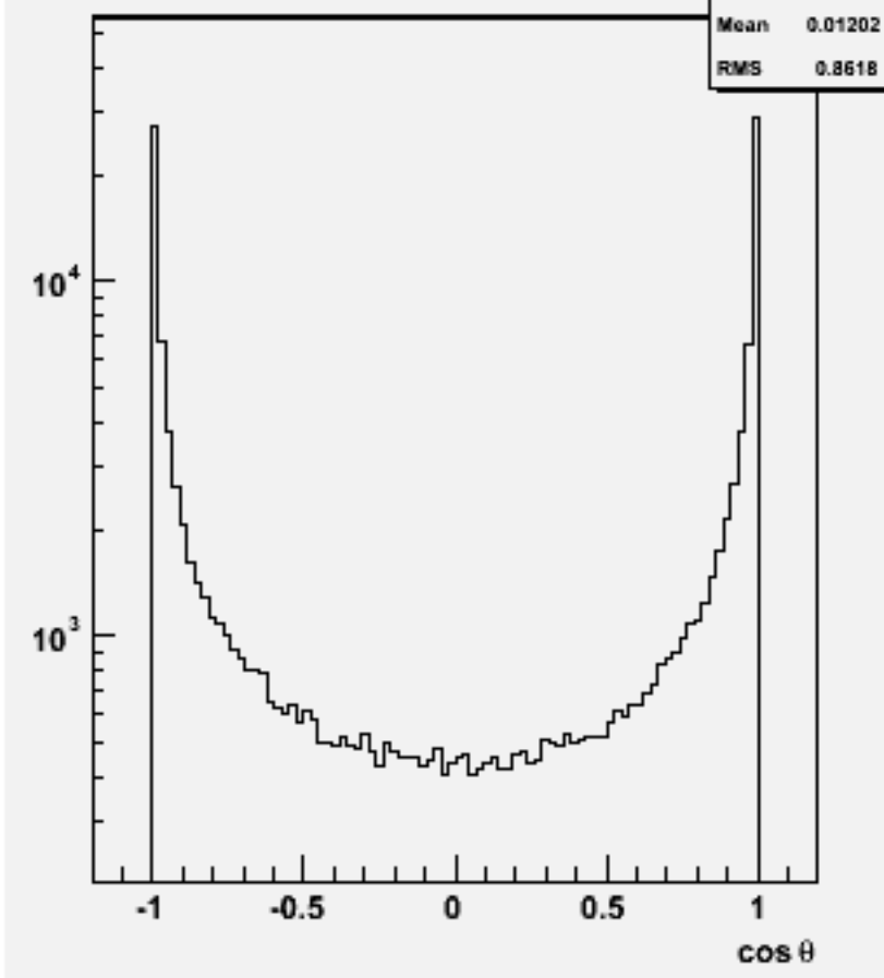
Particle cos \theta : w102466 e1e1e1e1e3e3_o
