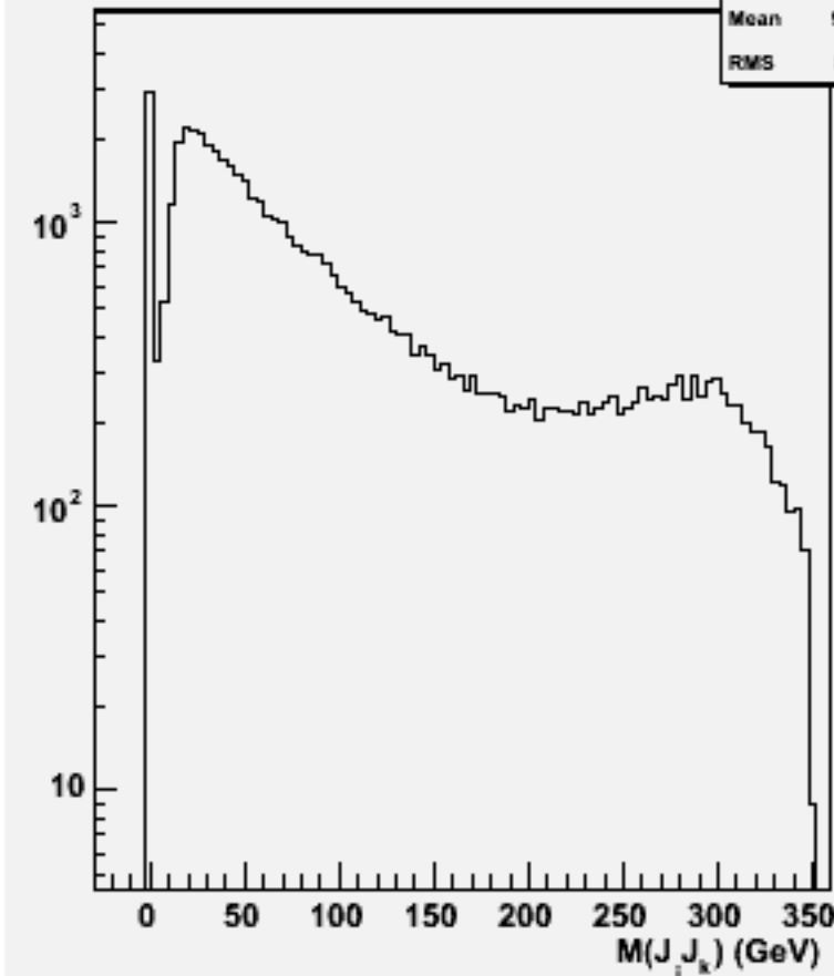
2jets mass(All comb)w102466 e1e1e1e1e3e3_o
