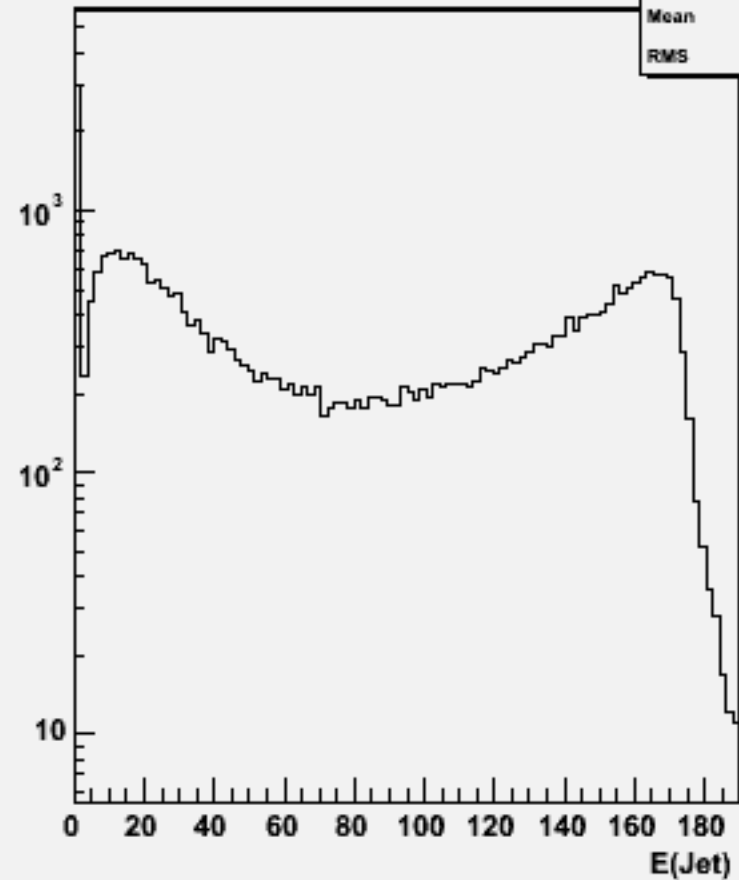
Jet energies(All jets)w102466 e1e1e1e1e3e3_o
