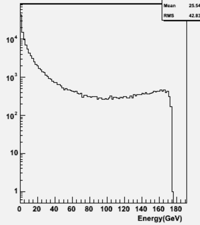
Start point R : w102466 e1e1e1e1e3e3_o
