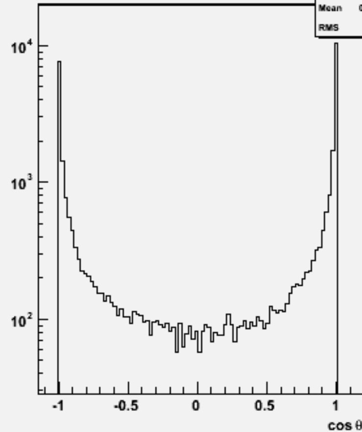
Jet cos \theta (All jets)w102466 e1e1e1e1e3e3_o
