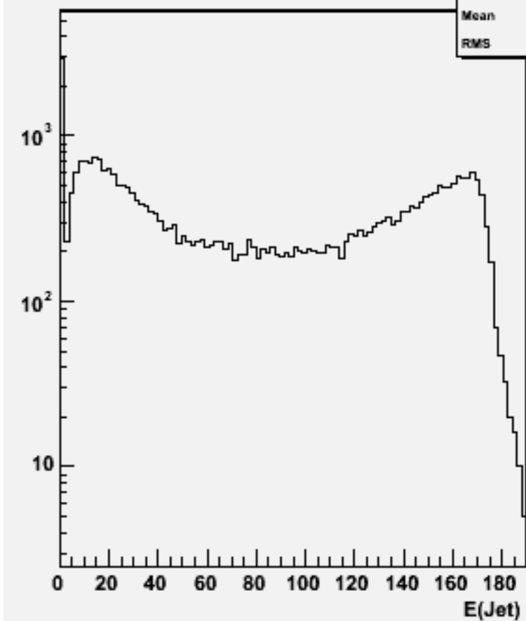
Jet energies(All jets)w102465 e1e1e1e1e3e3_o
