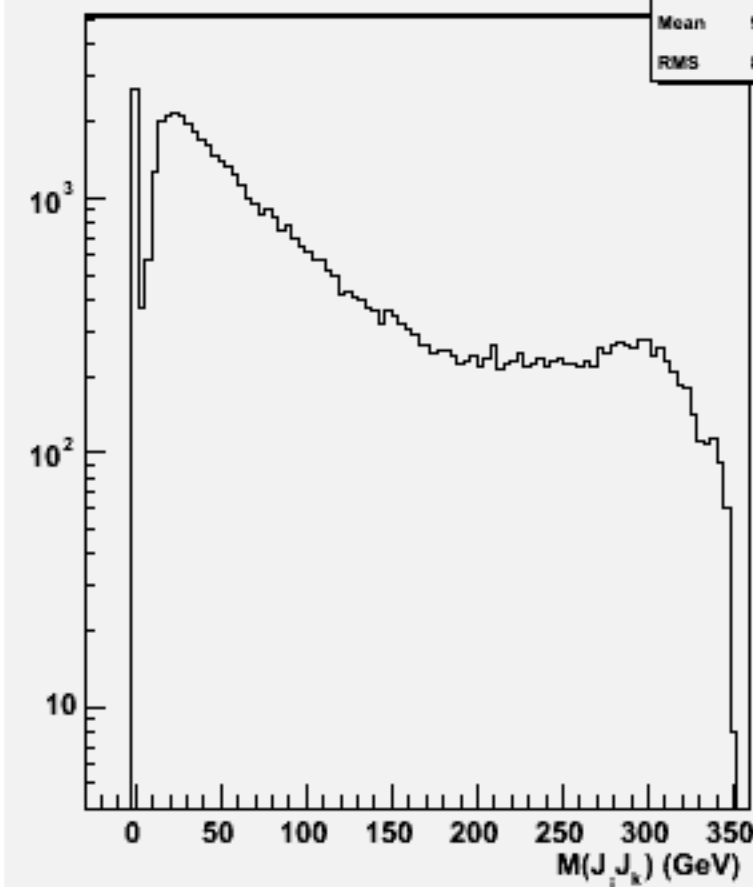
2jets mass(All comb)w102465 e1e1e1e1e3e3_o
