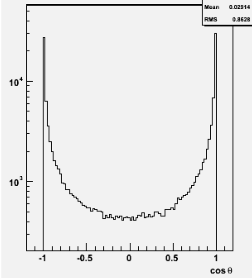
Particle cos θ : w102465 e1e1e1e1e3e3_o
