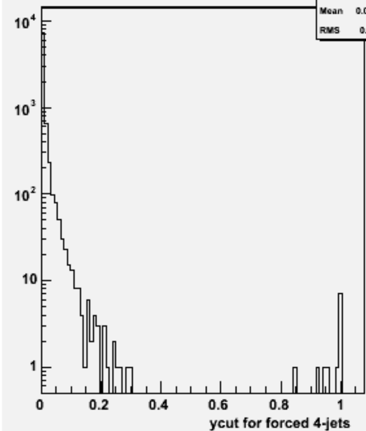
Ycut for 4-jets :w102465 e1e1e1e1e3e3_o
