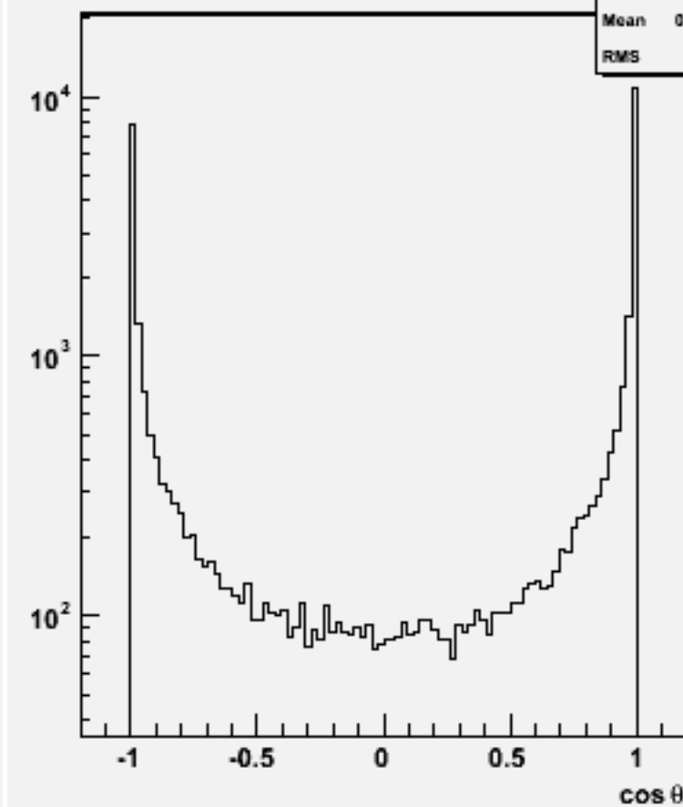
Jet cos \theta (All jets)w102465 e1e1e1e1e3e3_o
