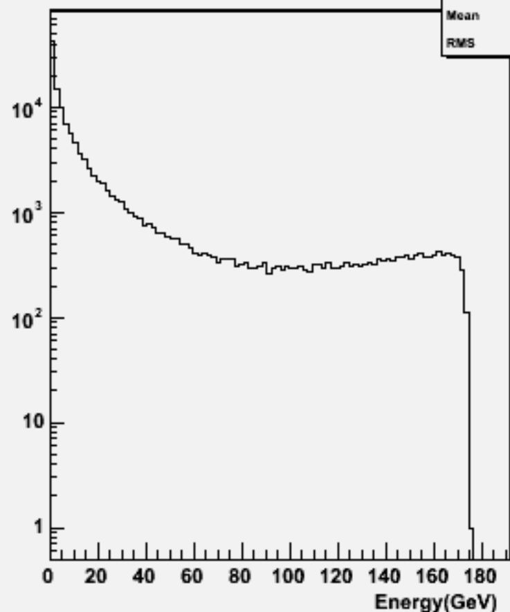
Particle Energy : w102464 e1e1e1e1e3e3_o
