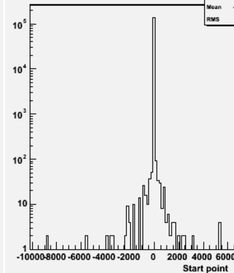
Start point Z : w102464 e1e1e1e1e3e3_o
