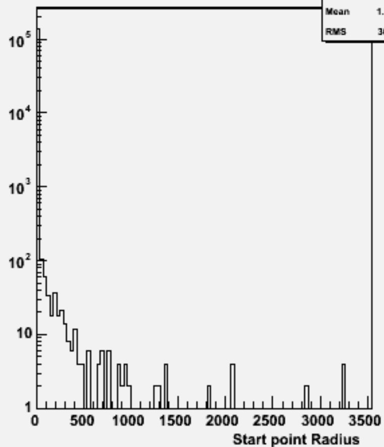
Start point R : w102464 e1e1e1e1e3e3_o
