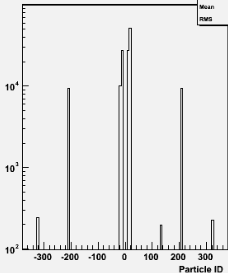
Particle ID : w102464 e1e1e1e1e3e3_o
