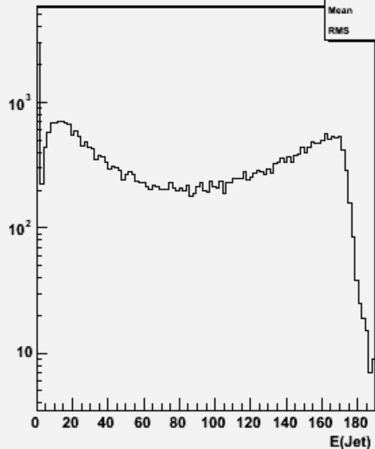
Jet energies(All jets)w102464 e1e1e1e1e3e3_o
