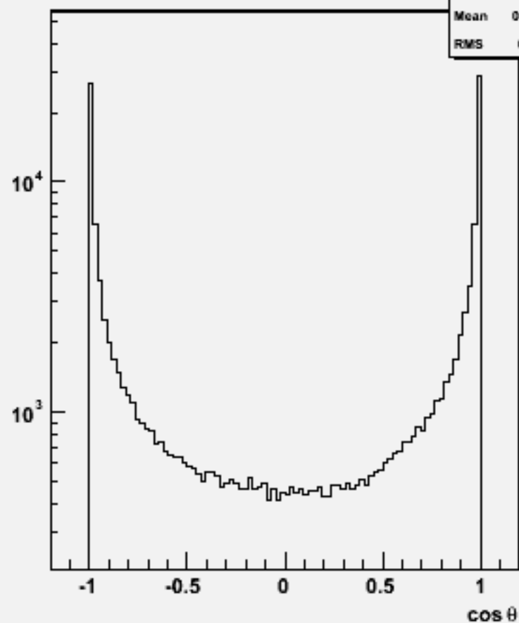
Particle cos \theta : w102464 e1e1e1e1e3e3_o
