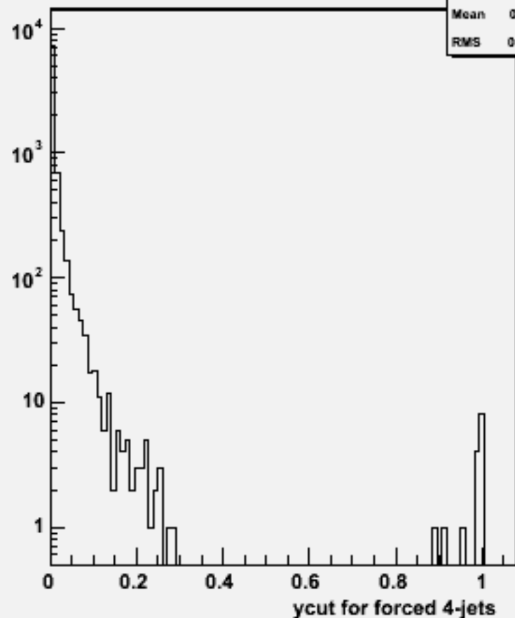
Ycut for 4-jets :w102464 e1e1e1e1e3e3_o
