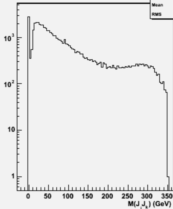
2jets mass(All comb)w102464 e1e1e1e1e3e3_o
