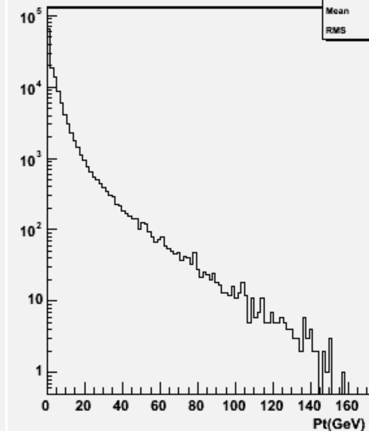
Particle Pt : w102464 e1e1e1e1e3e3_o
