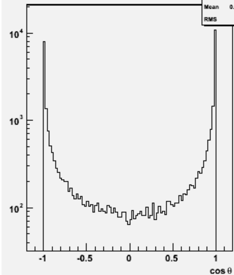
Jet cos \theta (All jets)w102463 e1e1e1e1e3e3_o
