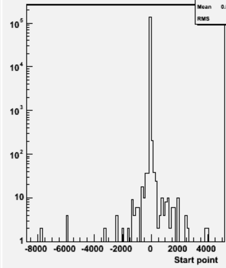
Start point Z : w102463 e1e1e1e1e3e3_o
