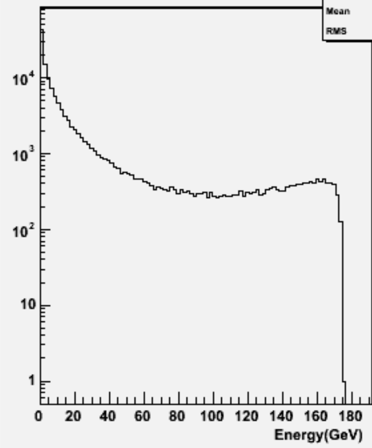
Start point R : w102463 e1e1e1e1e3e3_o
