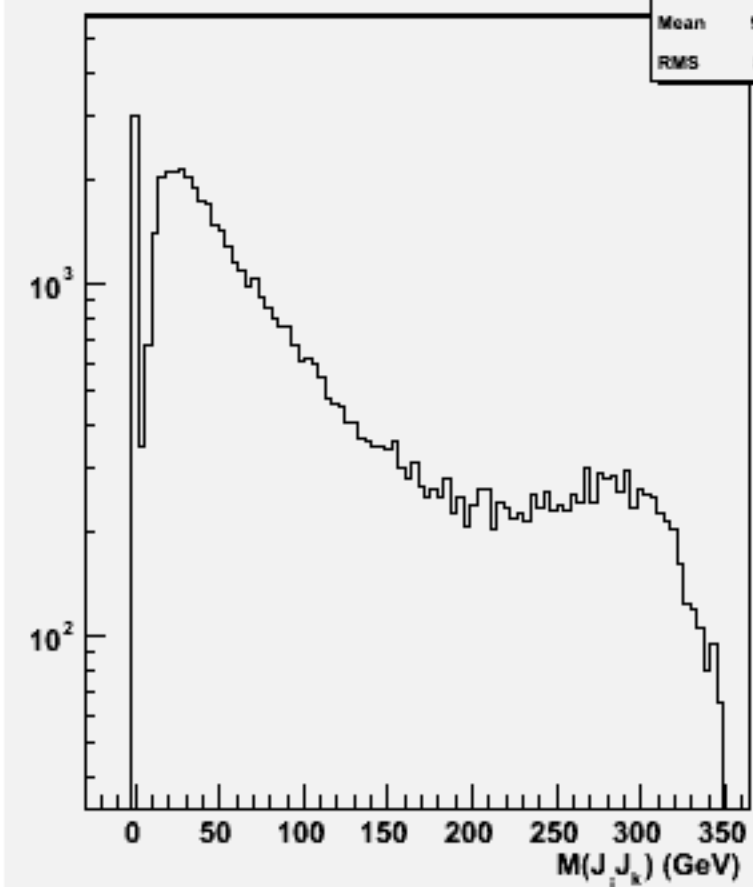
2jets mass(All comb)w102463 e1e1e1e1e3e3_o
