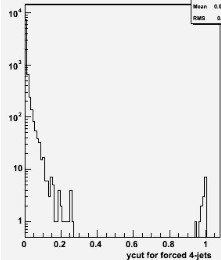
Ycut for 4-jets :w102463 e1e1e1e1e3e3_o
