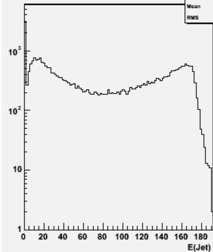
Jet energies(All jets)w102463 e1e1e1e1e3e3_o
