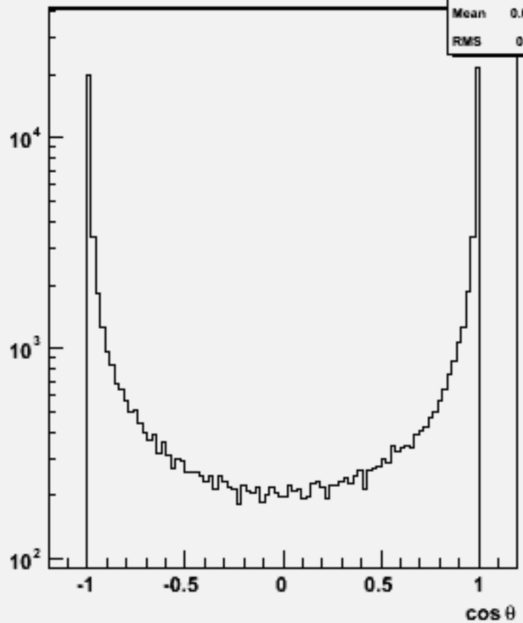
Particle cos \theta : w102461 e1e1e1e1e2e2_o
