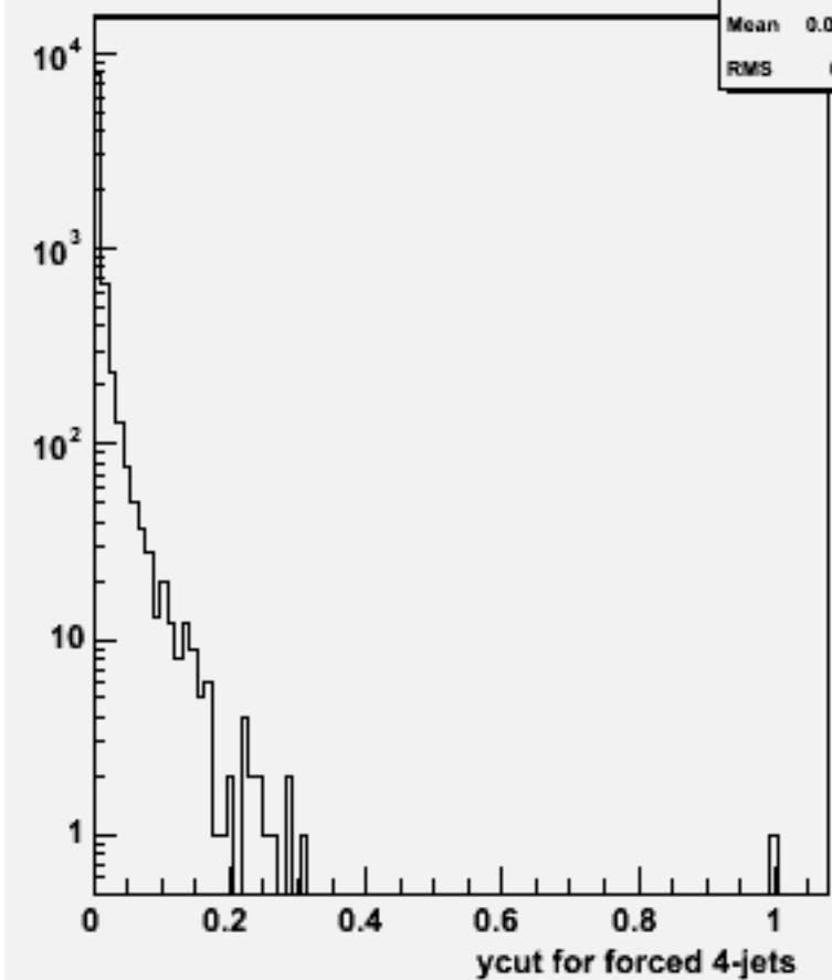
Ycut for 4-jets :w102461 e1e1e1e1e2e2_o
