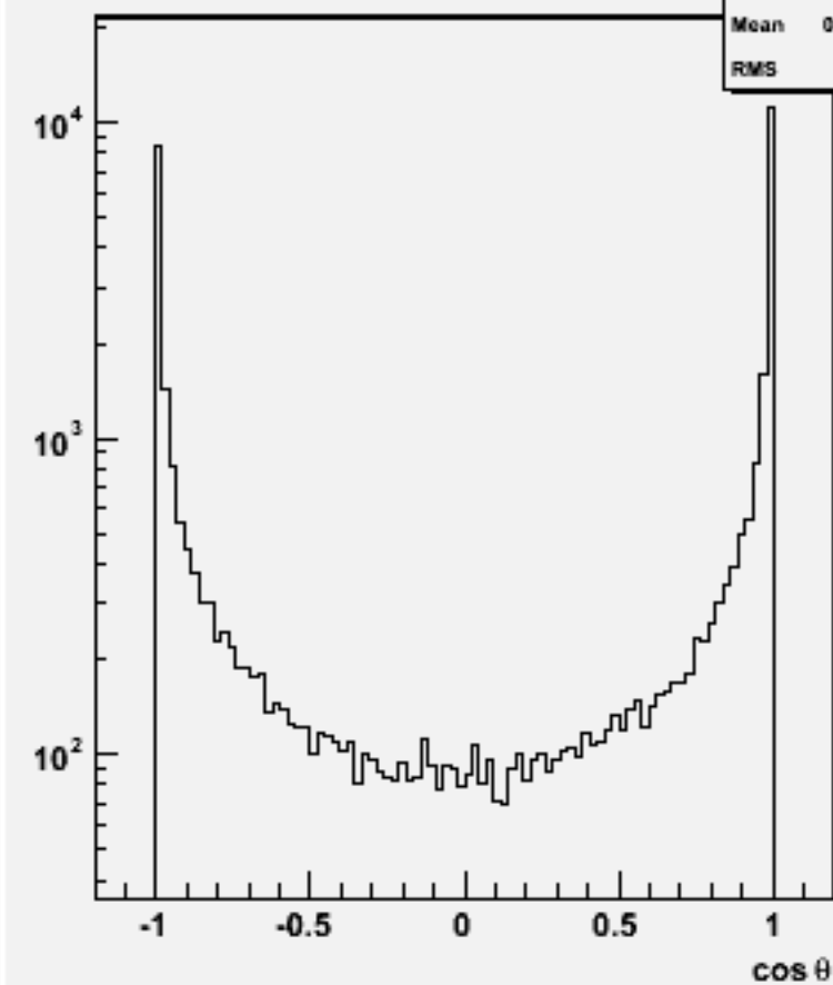
Jet cos \theta (All jets)w102461 e1e1e1e1e2e2_o
