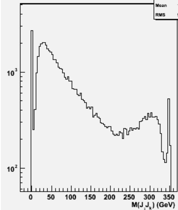
2jets mass(All comb)w102461 e1e1e1e1e2e2_o
