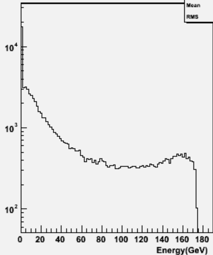
Start point R : w102461 e1e1e1e1e2e2_o
