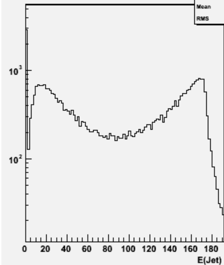
Jet energies(All jets)w102461 e1e1e1e1e2e2_o
