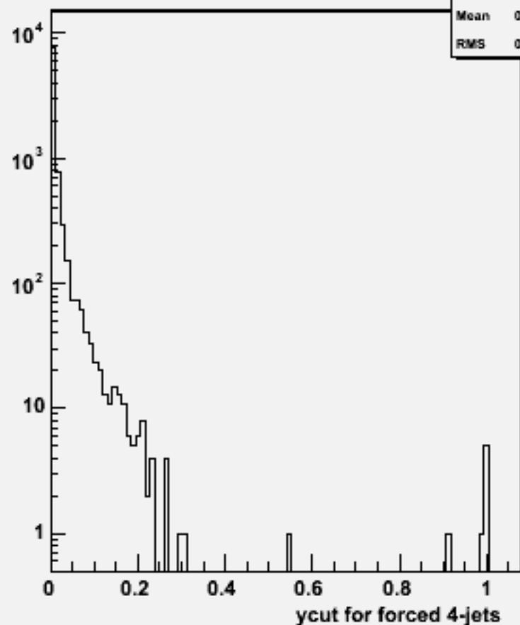
Ycut for 4-jets :w102460 e1e1e1e1e2e2_o
