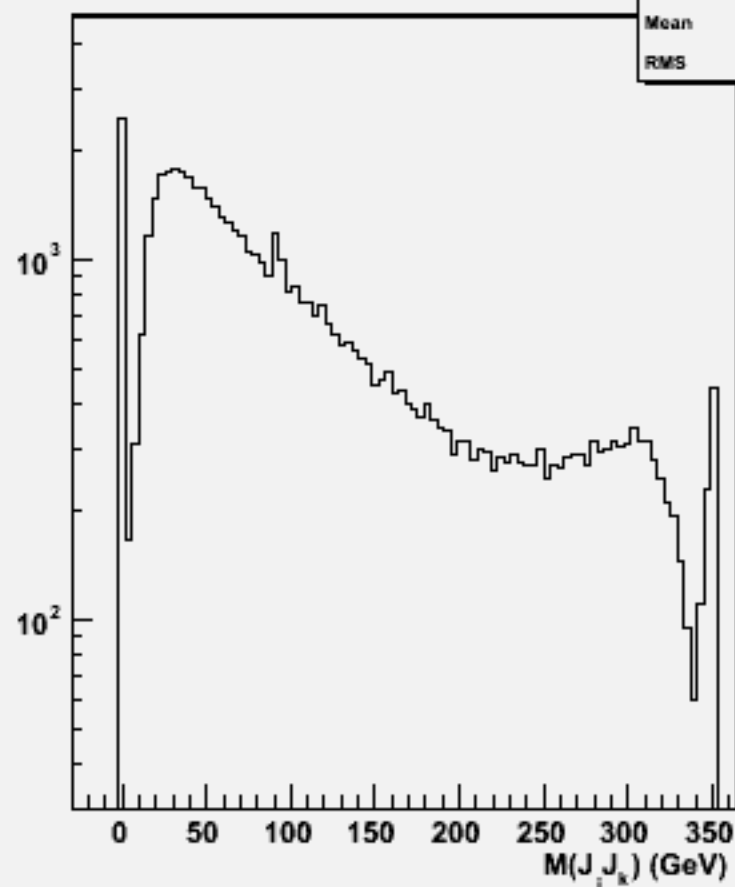
2jets mass(All comb)w102460 e1e1e1e1e2e2_o
