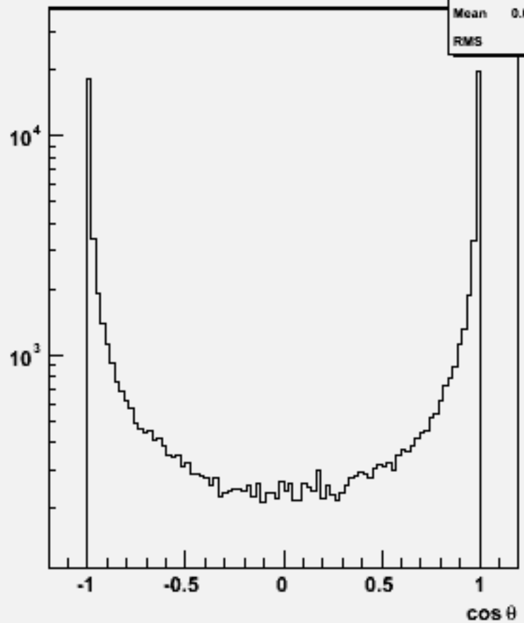
Particle cos \theta : w102460 e1e1e1e1e2e2_o
