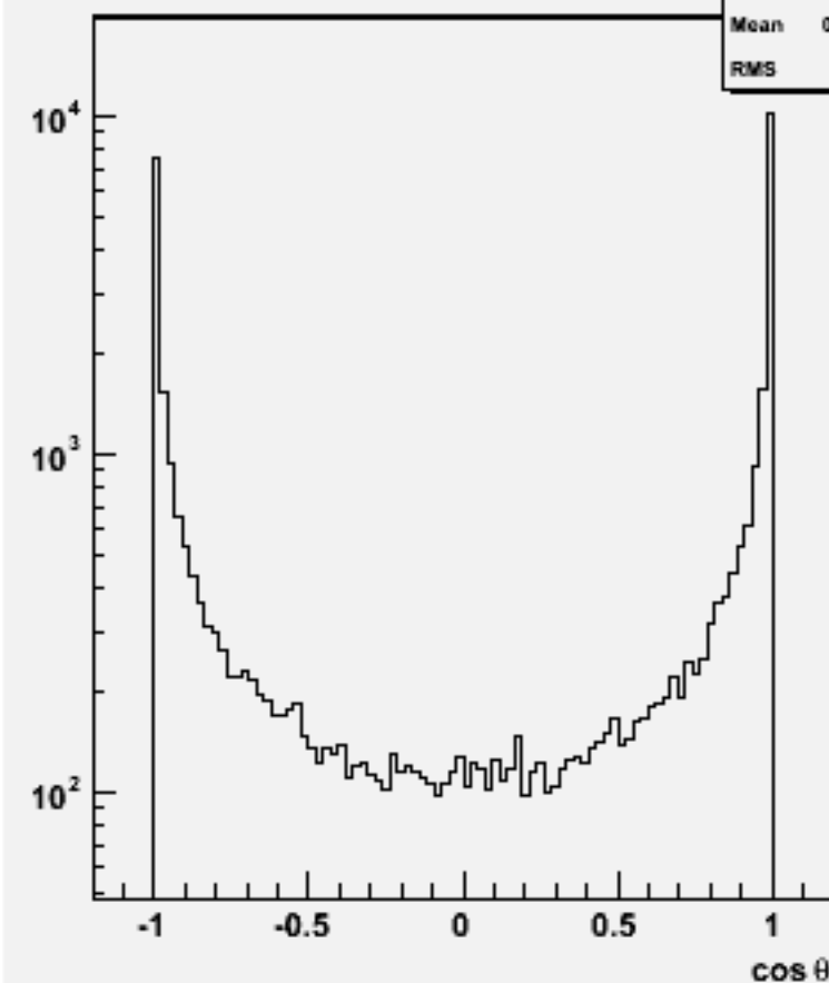
Jet cos \theta (All jets)w102460 e1e1e1e1e2e2_o
