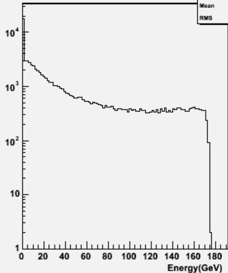
Start point R : w102460 e1e1e1e1e2e2_o
