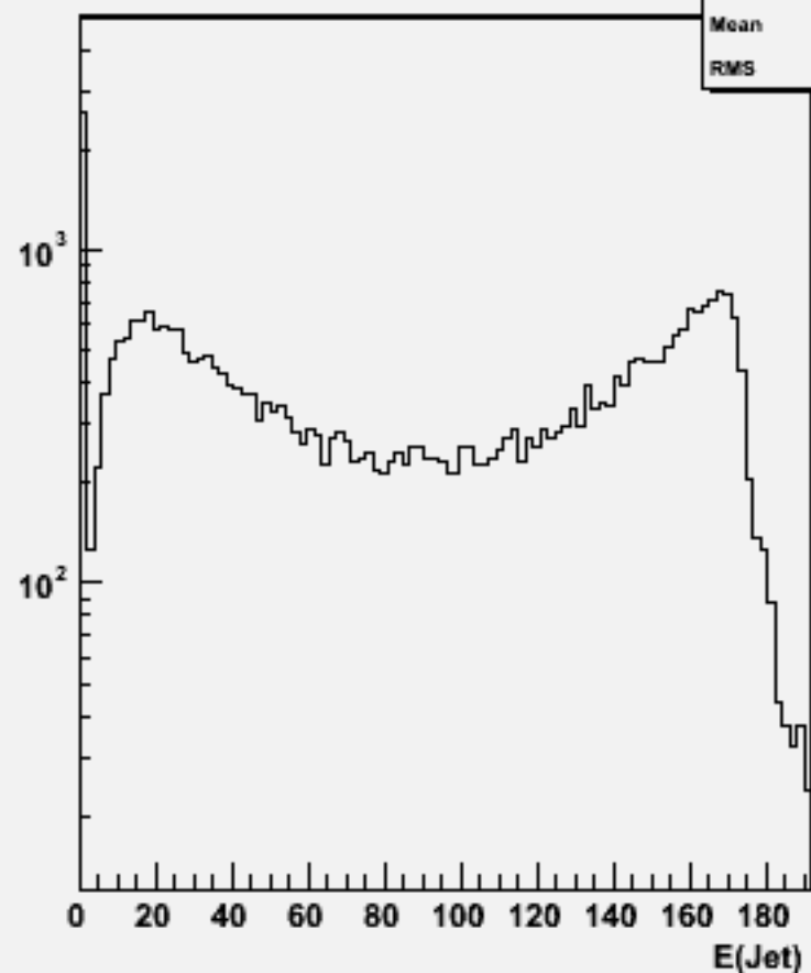
Jet energies(All jets)w102460 e1e1e1e1e2e2_o
