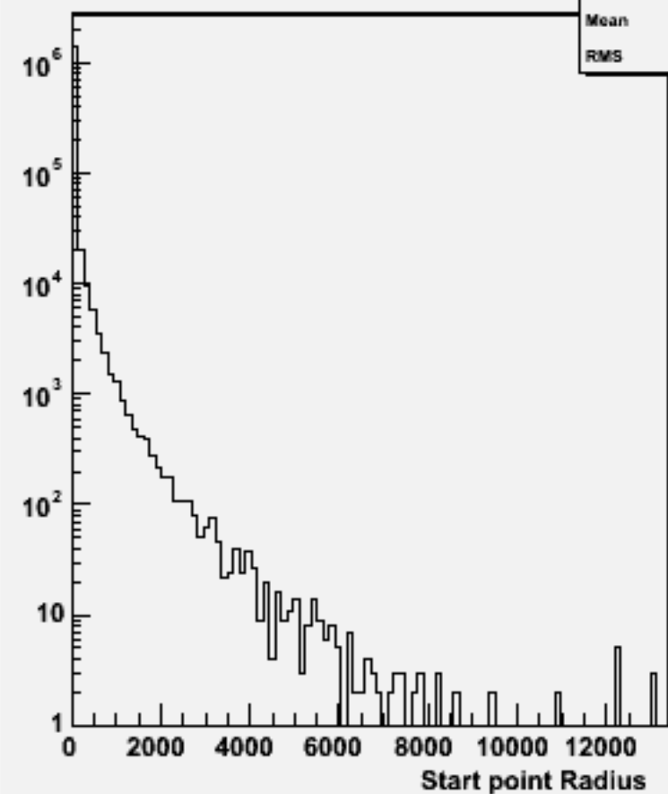
Start point R : w102452 ccbbbb_o
