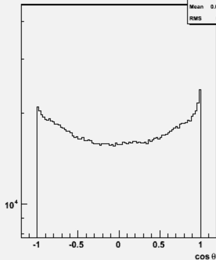
Particle cosθ : w102452 ccbbbb_o
