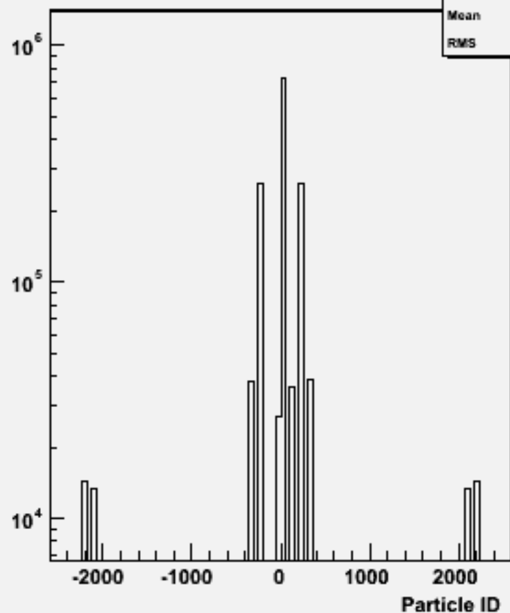
Particle ID : w102452 ccbbbb_o
