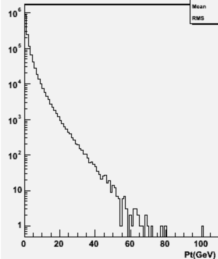
Particle Pt : w102452 ccbbbb_o
