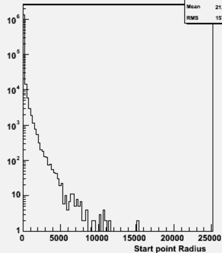
Start point R : w102448 ccddbb_o
