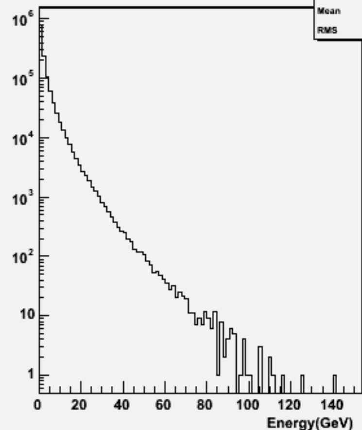
Start point R : w102448 ccddbb_o
