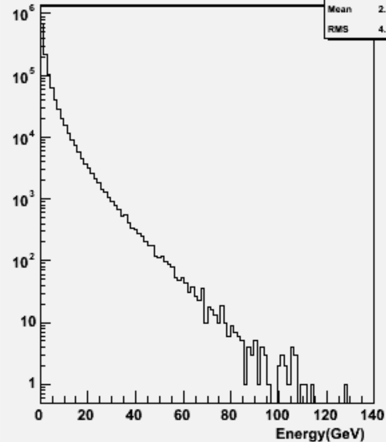
Start point R : w102444 ccdddd_o
