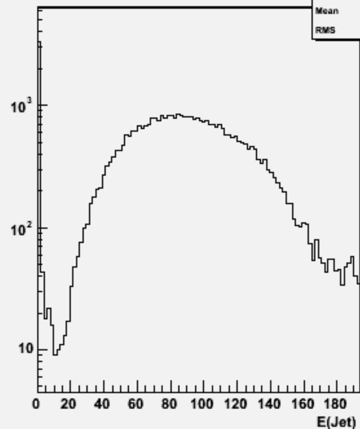
Jet energies(All jets)w102444 ccdddd_o
