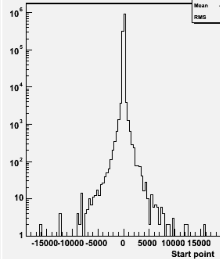
Start point Z : w102444 ccdddd_o
